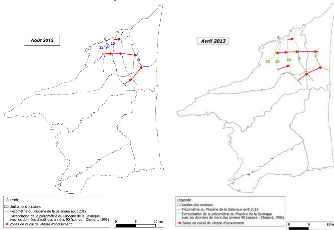
Figure 18 : Zones de calcul de vitesse d'écoulement dans le Pliocène de la Salanque
