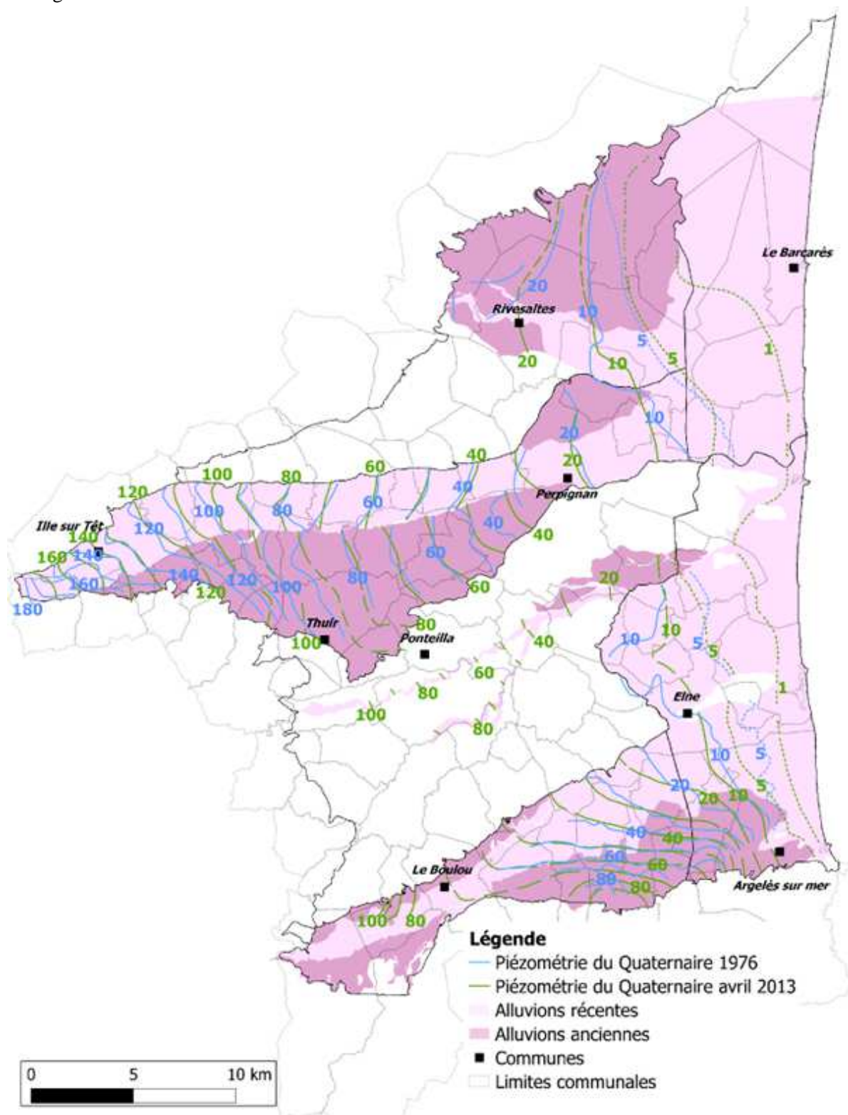
Figure 10 : Piézométries 1976 et 2013 du Quaternaire
