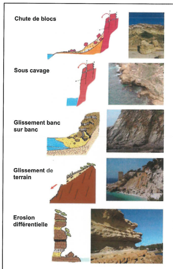
Figure 4 : Typologie des instabilités et des érosions dans le contexte des falaises côtières en région PACA (Source : BRGM, 2005)
