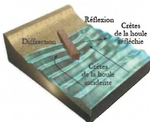
Figure 3 : Transformations de la houle à l'approche des côtes (Source : SDAGE bassin Rhône Méditerranée et bassin Corse, 2005)
