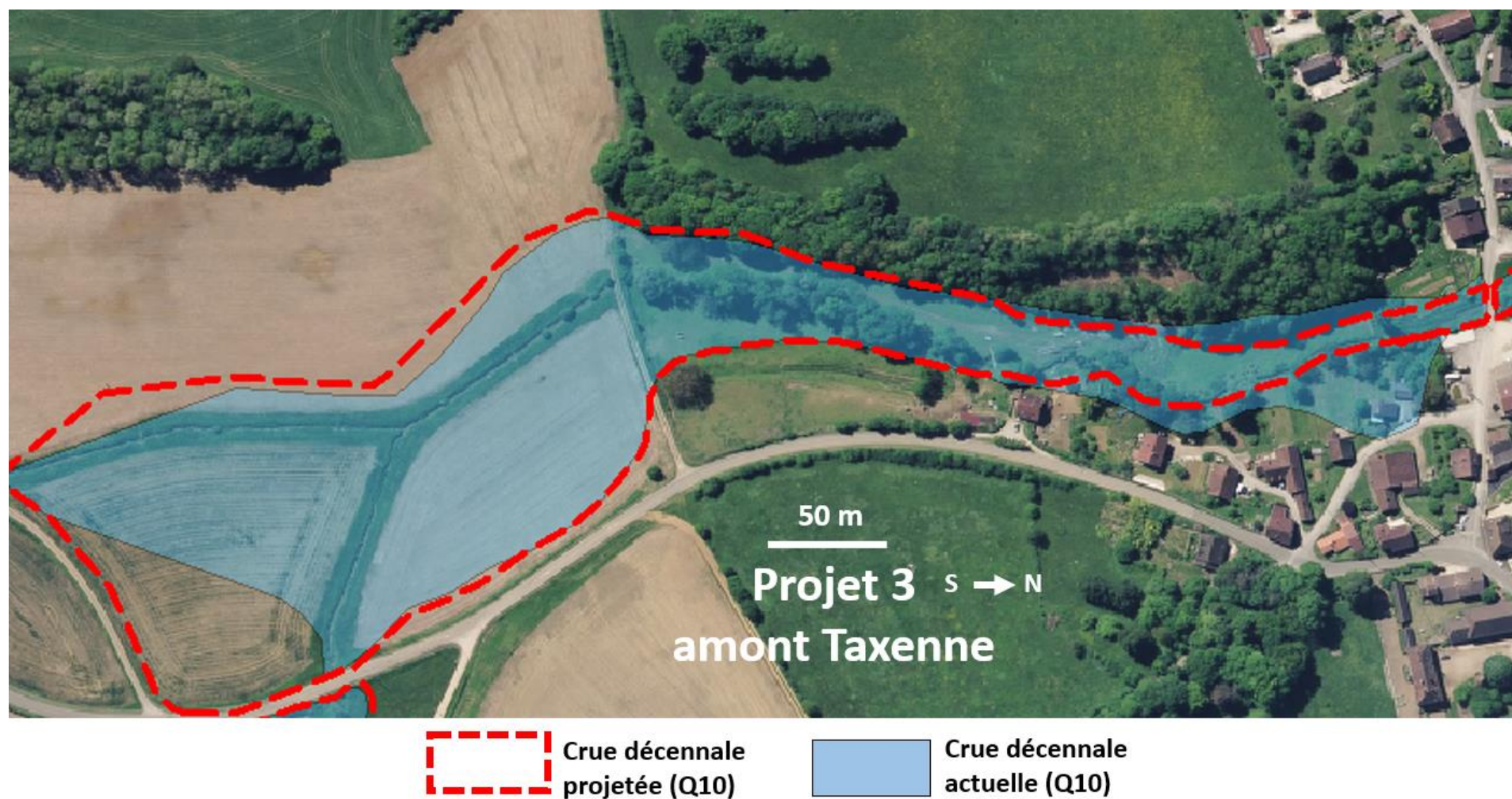
Figure 15.37 : Zones inondables actuelles et futures en crue décennale pour le projet « 3 Amont Taxenne »
