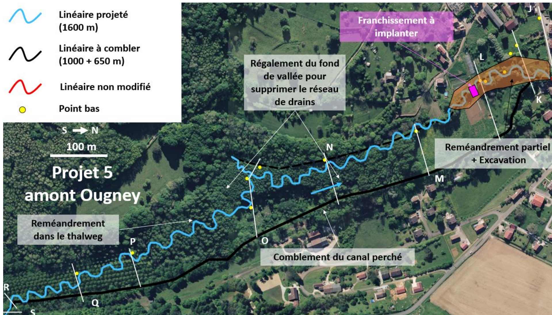
Figure 20.6 : Détails du projet 5 Amont Ougney
