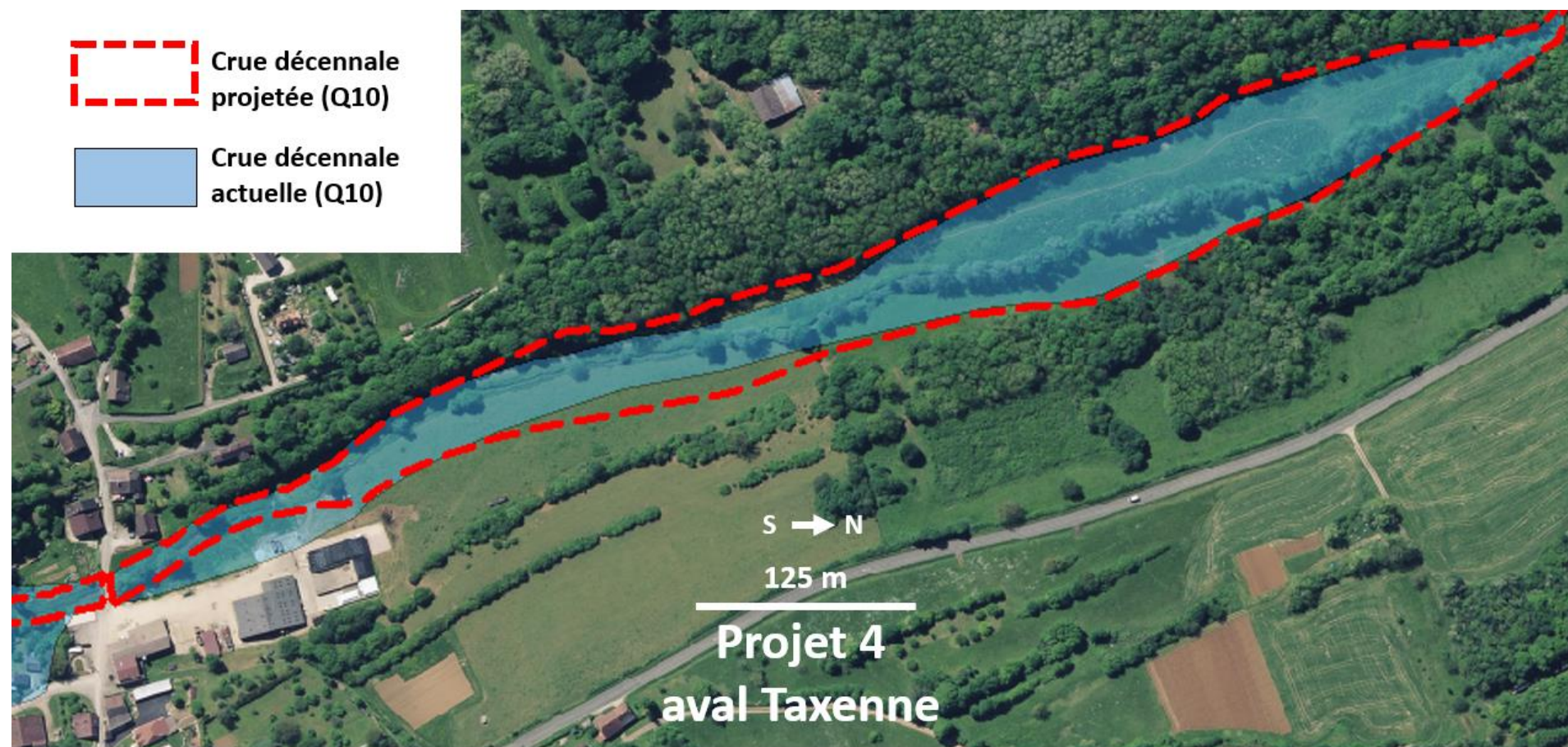
Figure 15.40 : Zones inondables actuelles et futures en crue décennale pour le projet « 4 Aval Taxenne »
