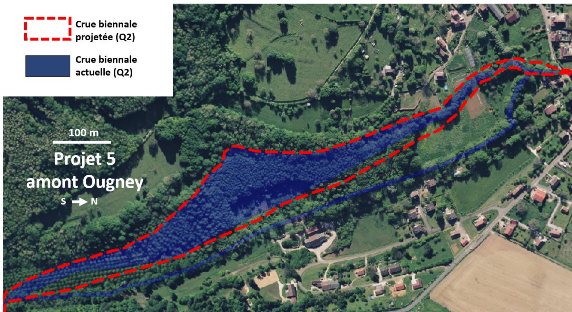
Figure 15.42 : Zones inondables actuelles et futures en crue biennale pour le projet « 5 Amont Ougney »
