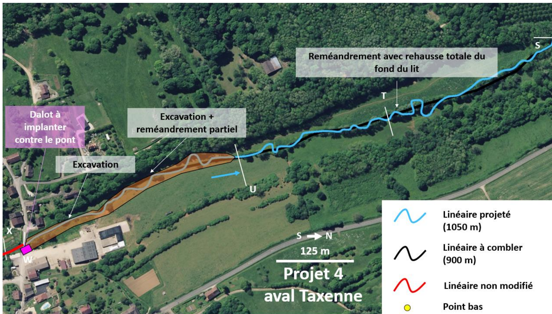
Figure 6.14 : Stratégie de restauration pour le projet « 4 Aval Taxenne »
