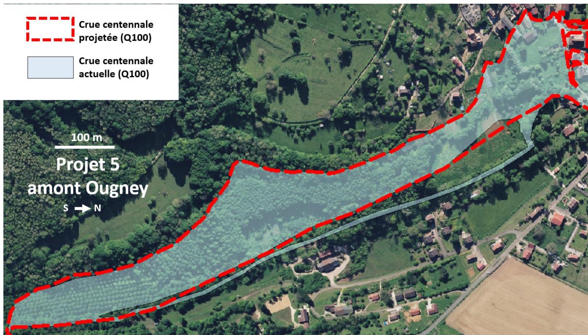
Figure 15.44 : Zones inondables actuelles et futures en crue centennale pour le projet « 5 Amont Ougney »
