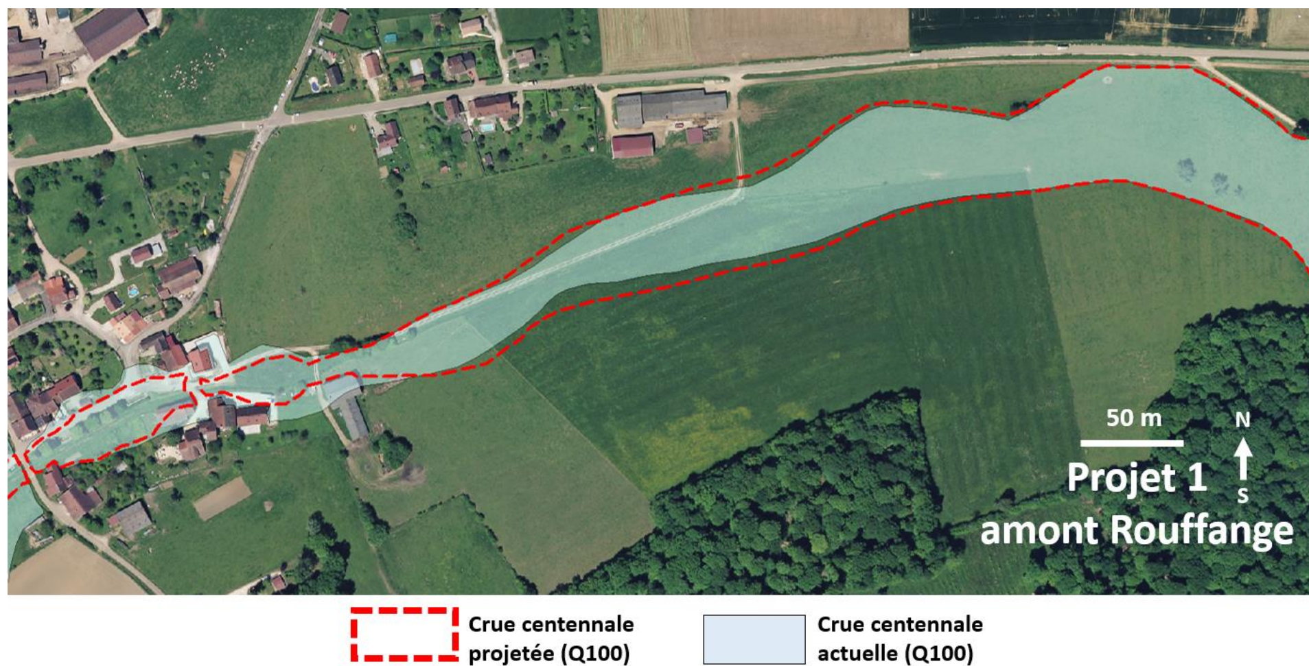
Figure 15.32 : Zones inondables actuelles et futures en crue centennale pour le projet « 1 Amont Rouffange »
