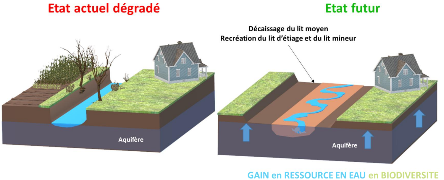
Figure 6.8 : Principe d'aménagement préconisé sur les secteurs à aléas d'inondation contraignants.
