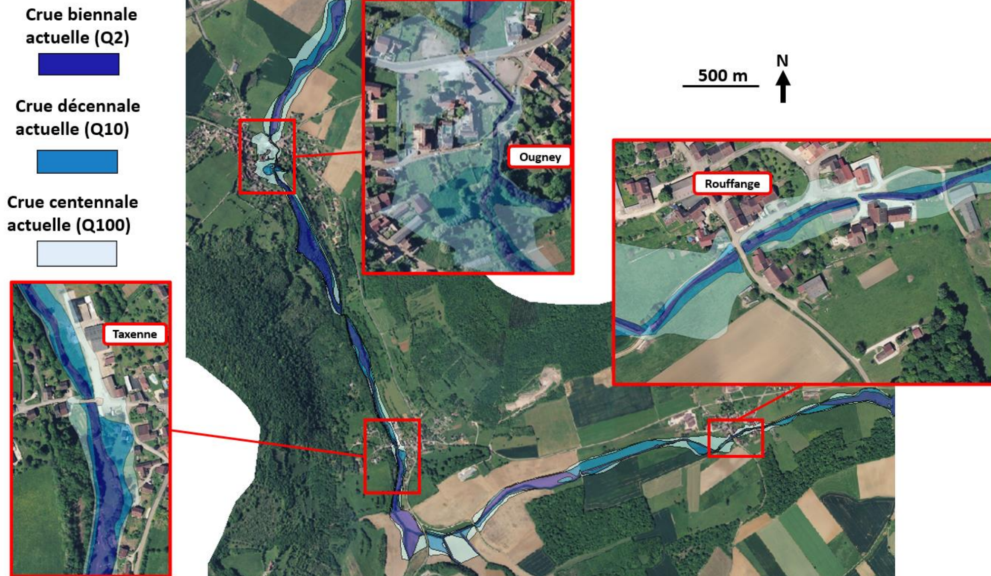
Figure 15.4 : cartes des inondations de la Vèze sur les communes de Rouffange, Taxenne et Ougney.
