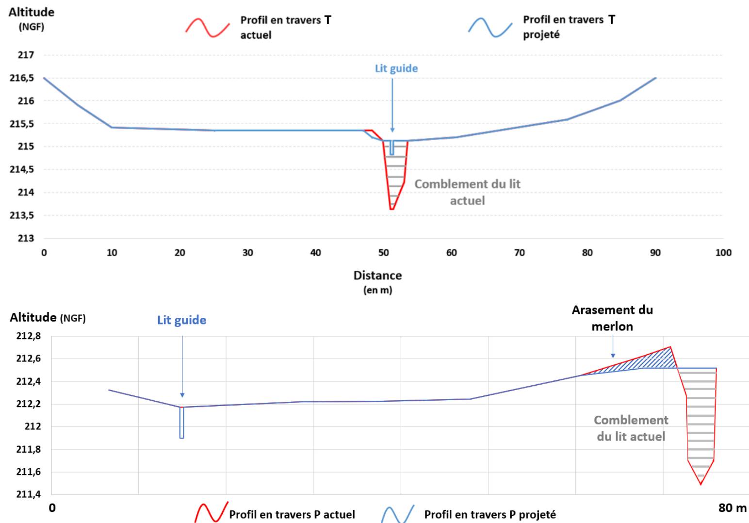
Figure 6.6 : Profil en travers P et T actuel et projeté.
