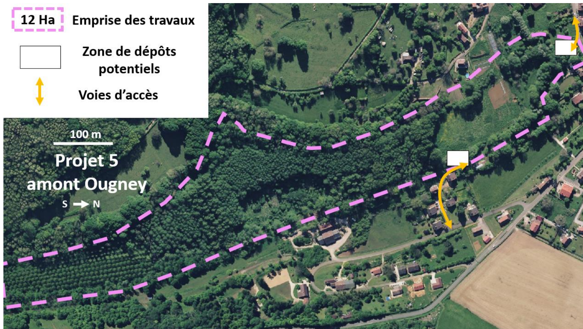
Figure 9.5 : Voies d'accès au chantier (flèches blanches) et zone de dépôts pressenties (carrés blancs) pour le projet « 5 Amont Ougney ».
