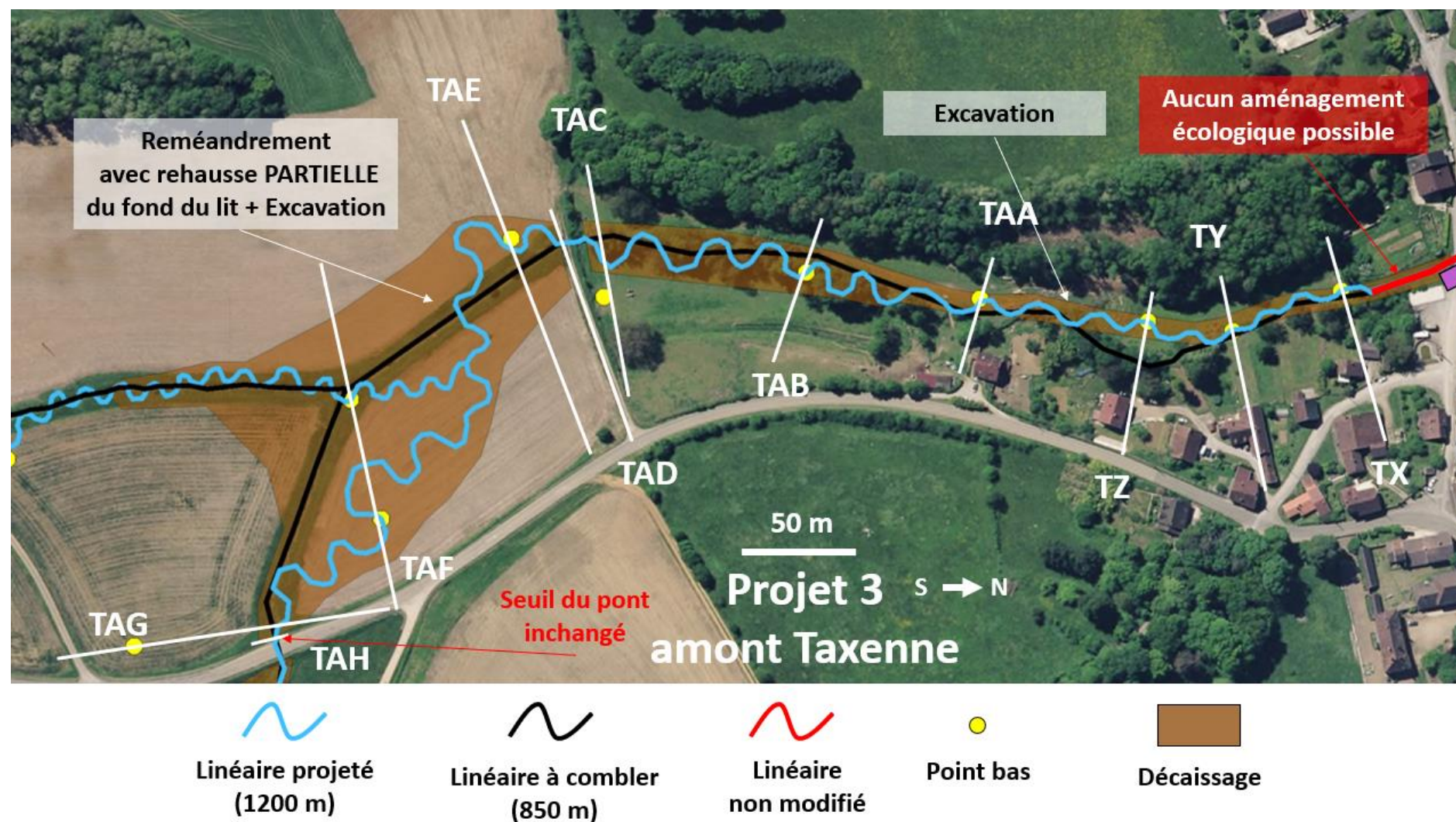
Figure 20.4 : Détails du projet 3 Amont Taxenne
