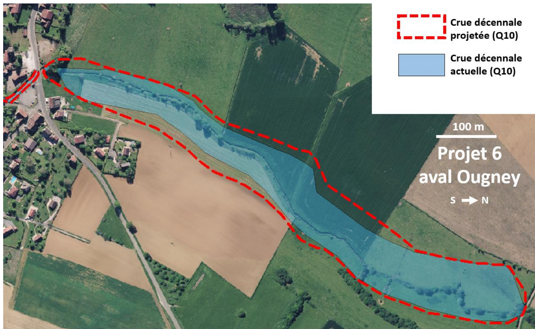
Figure 15.46 : Zones inondables actuelles et futures en crue décennale pour le projet « 6 Aval Ougney »
