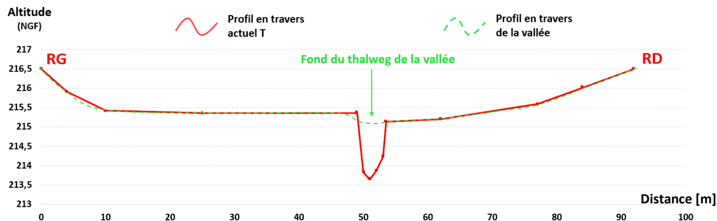
Figure 6.3 : Profil en travers actuel montrant la déconnexion latérale de la Vèze de plus de 1,5 m.
