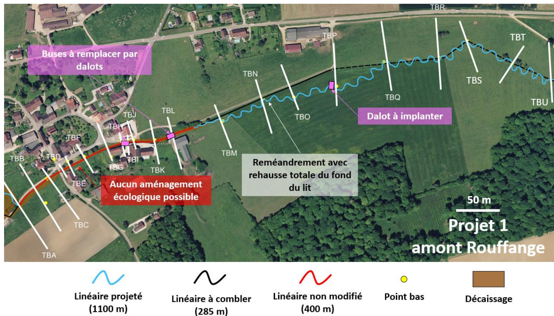
Figure 21.2 : Détails du projet 1 Amont Rouffange
