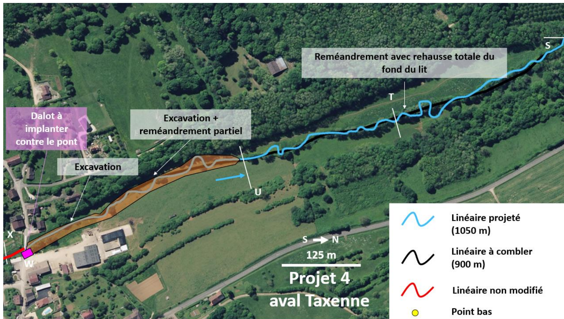
Figure 20.5 : Détails du projet 4 Aval Taxenne
