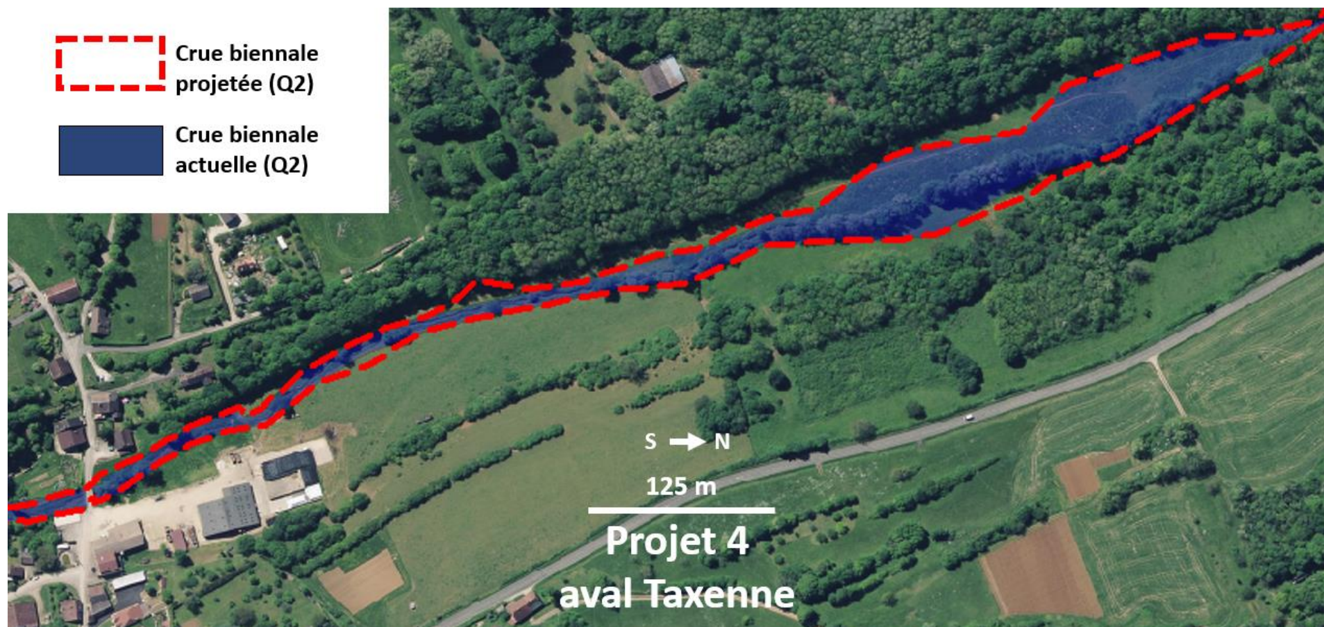
Figure 15.39 : Zones inondables actuelles et futures en crue biennale pour le projet « 4 Aval Taxenne »
