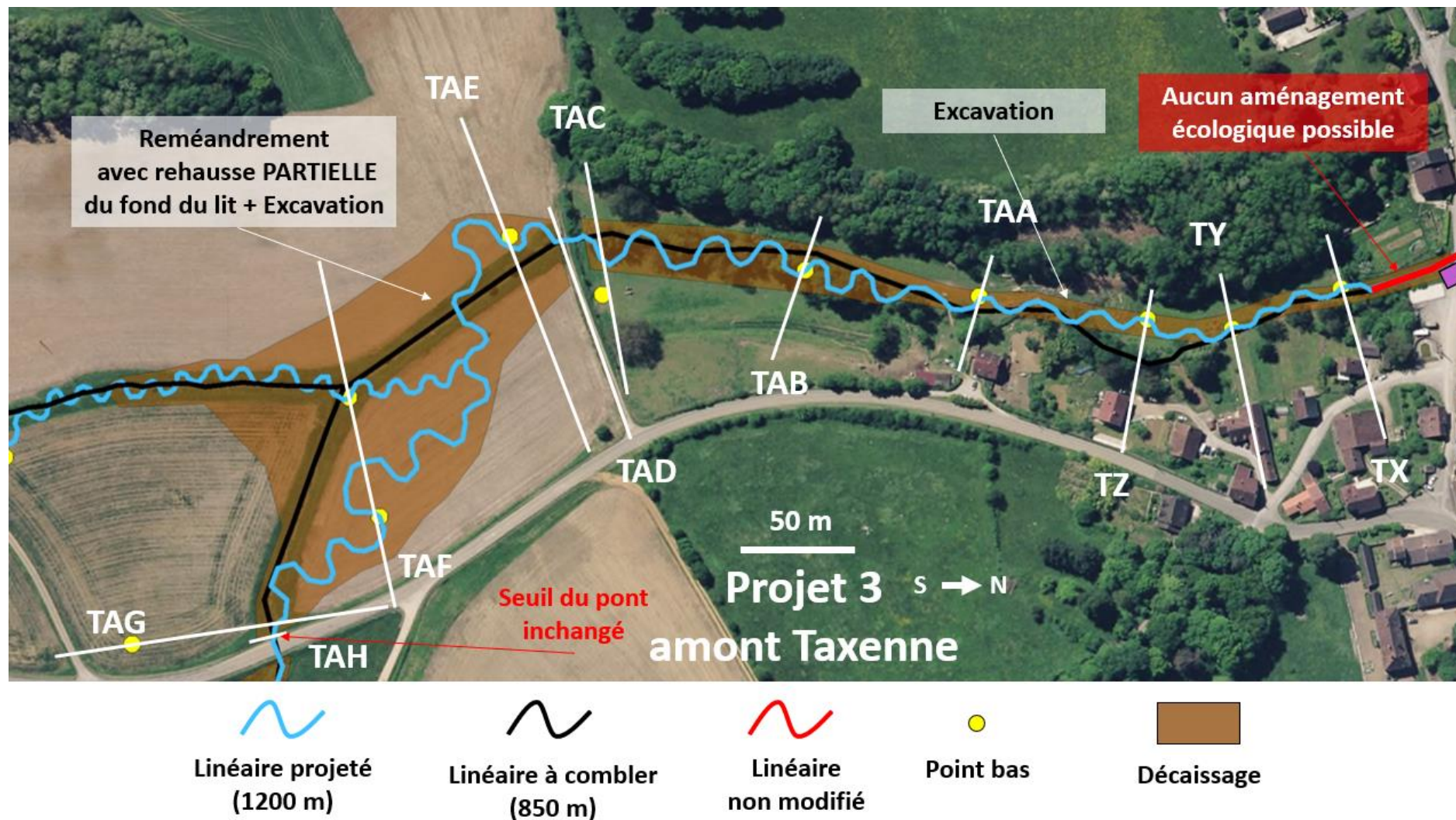
Figure 21.4 : Détails du projet 3 Amont Taxenne
