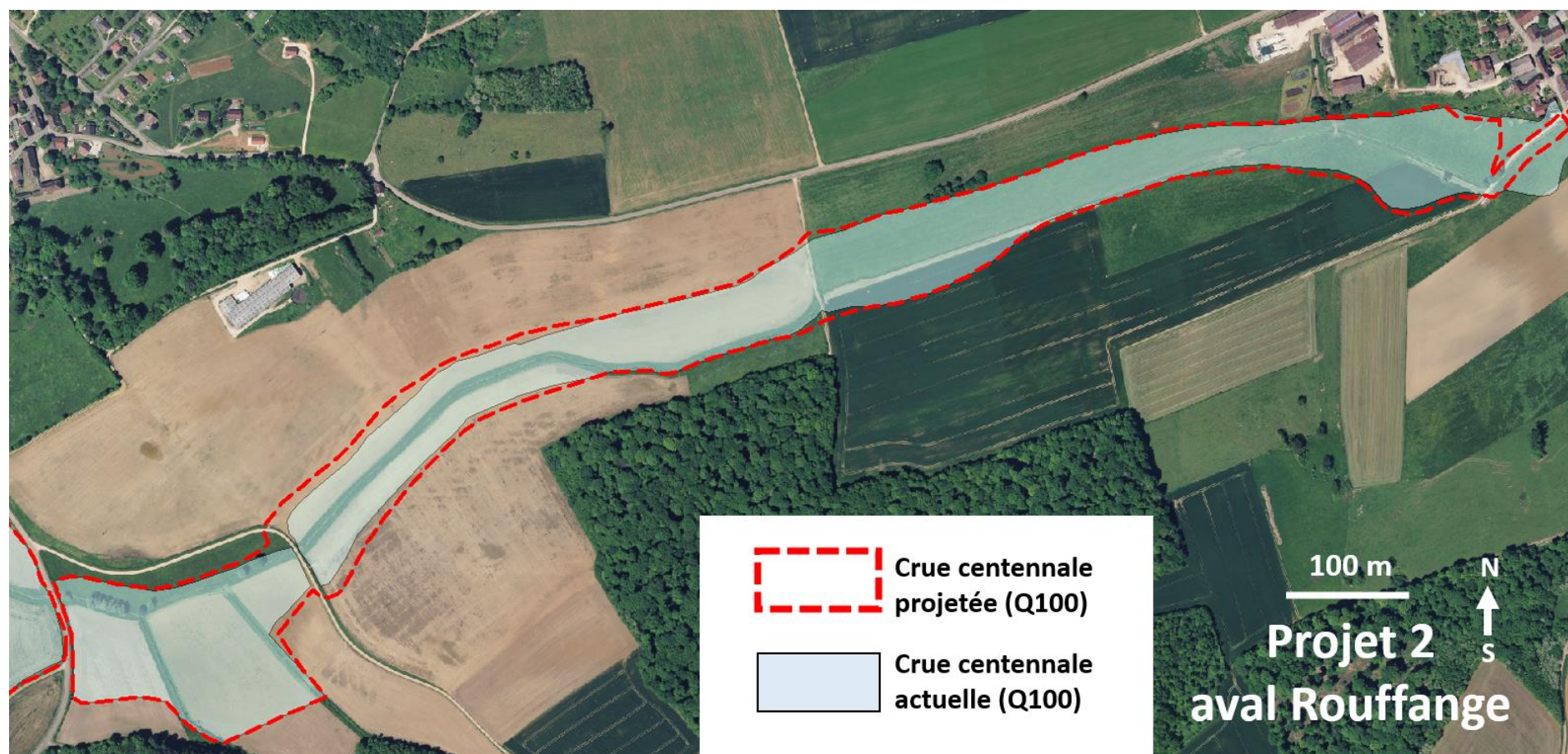
Figure 15.35 : Zones inondables actuelles et futures en crue centennale pour le projet « 2 Aval Rouffange »
