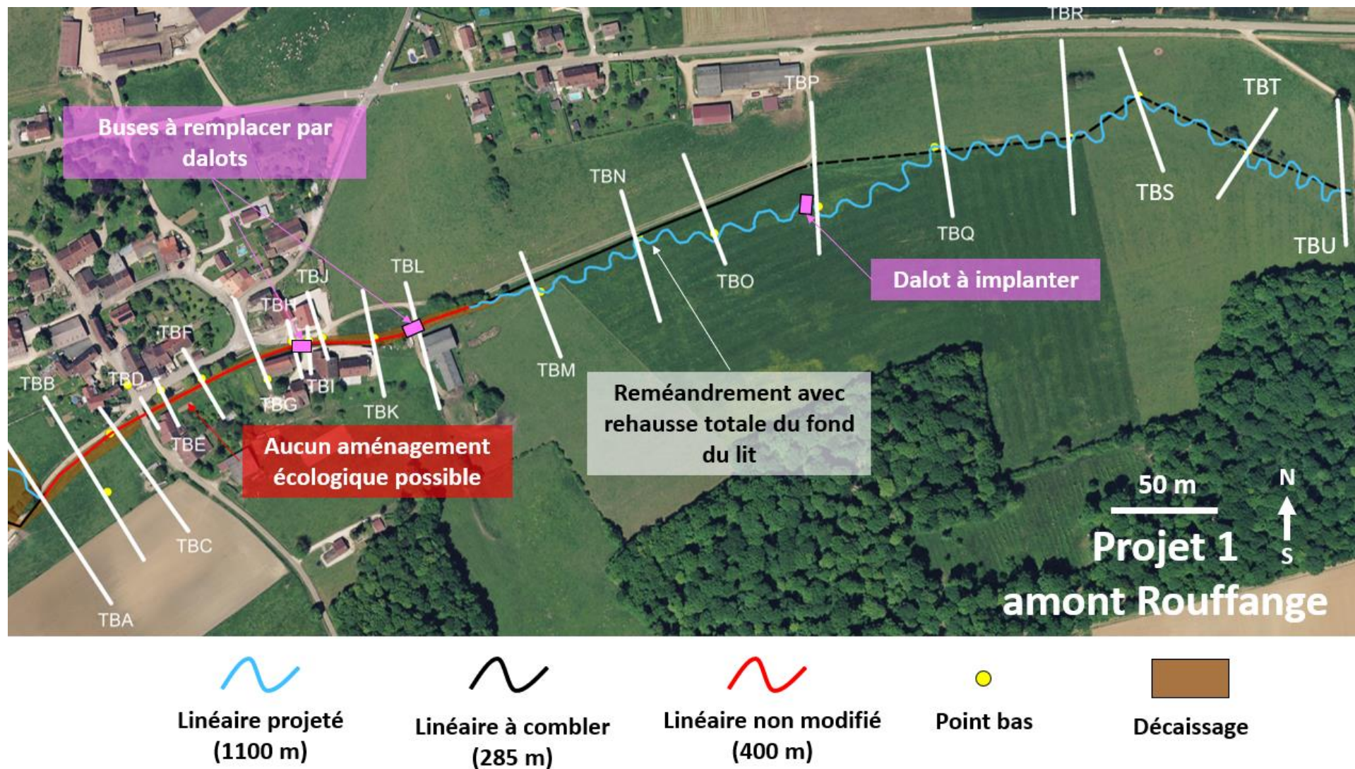
Figure 6.11 : Stratégie de restauration pour le projet « 1 Amont Rouffange »
