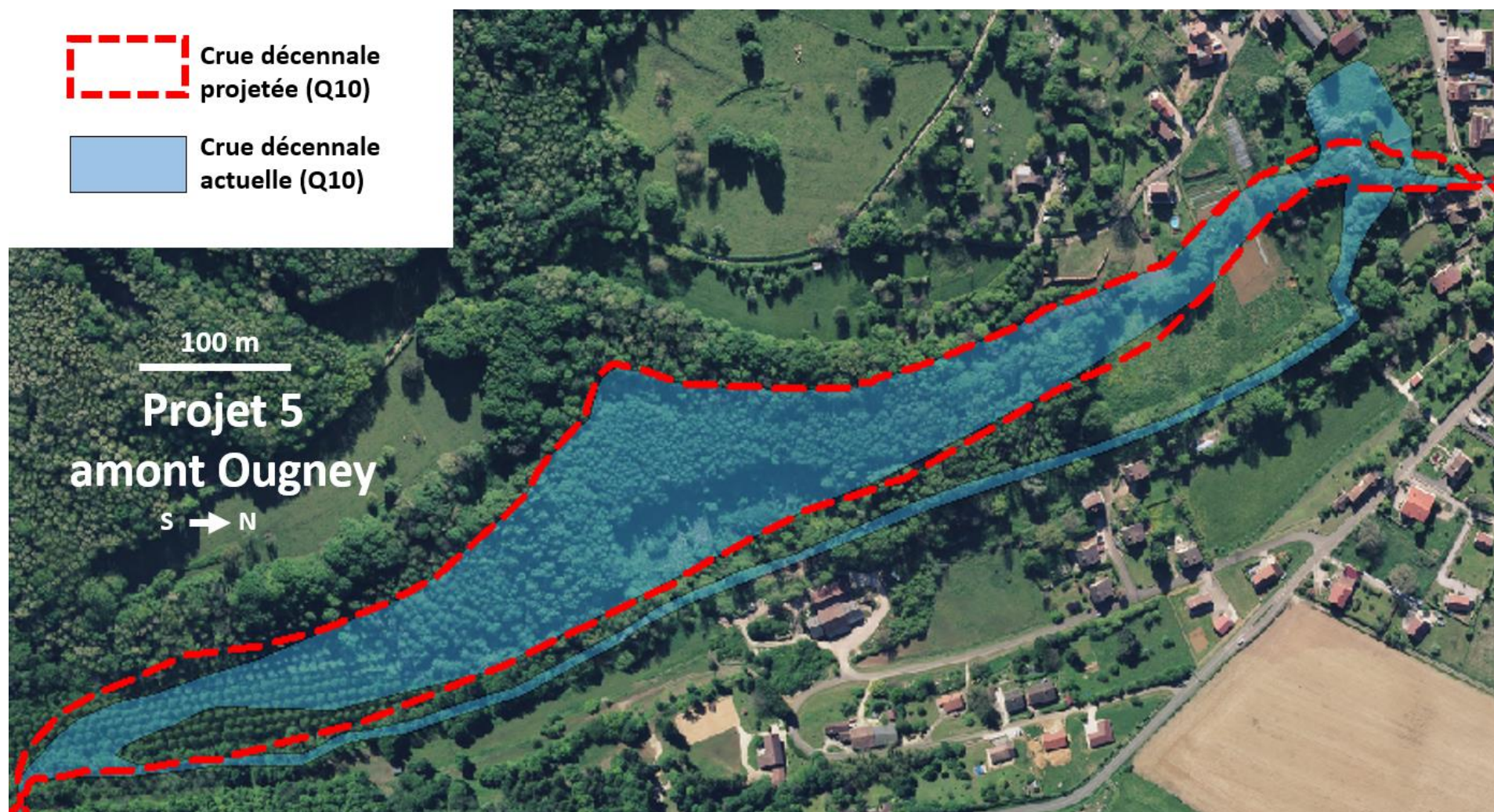
Figure 15.43 : Zones inondables actuelles et futures en crue décennale pour le projet « 5 Amont Ougney »
