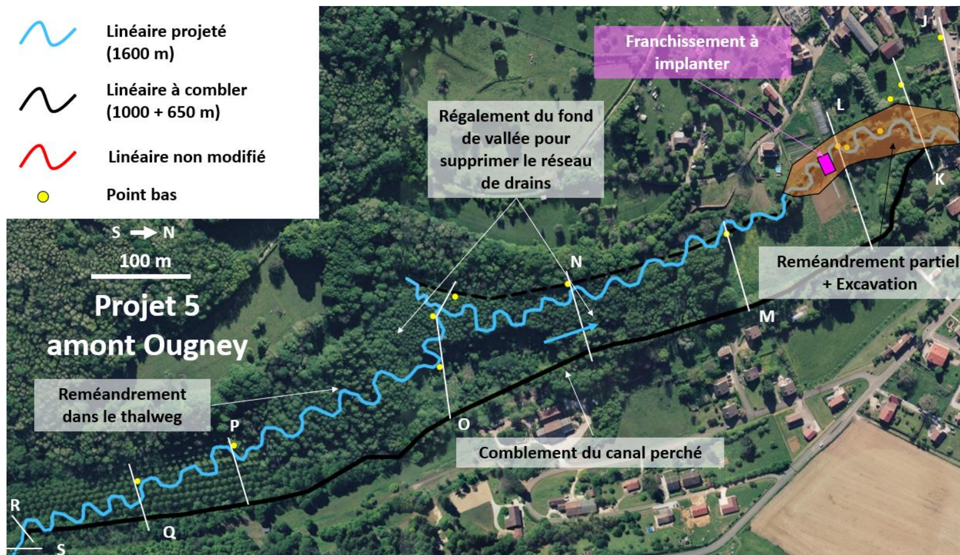
Figure 6.15 : Stratégie de restauration pour le projet « 5 Amont Ougney »
