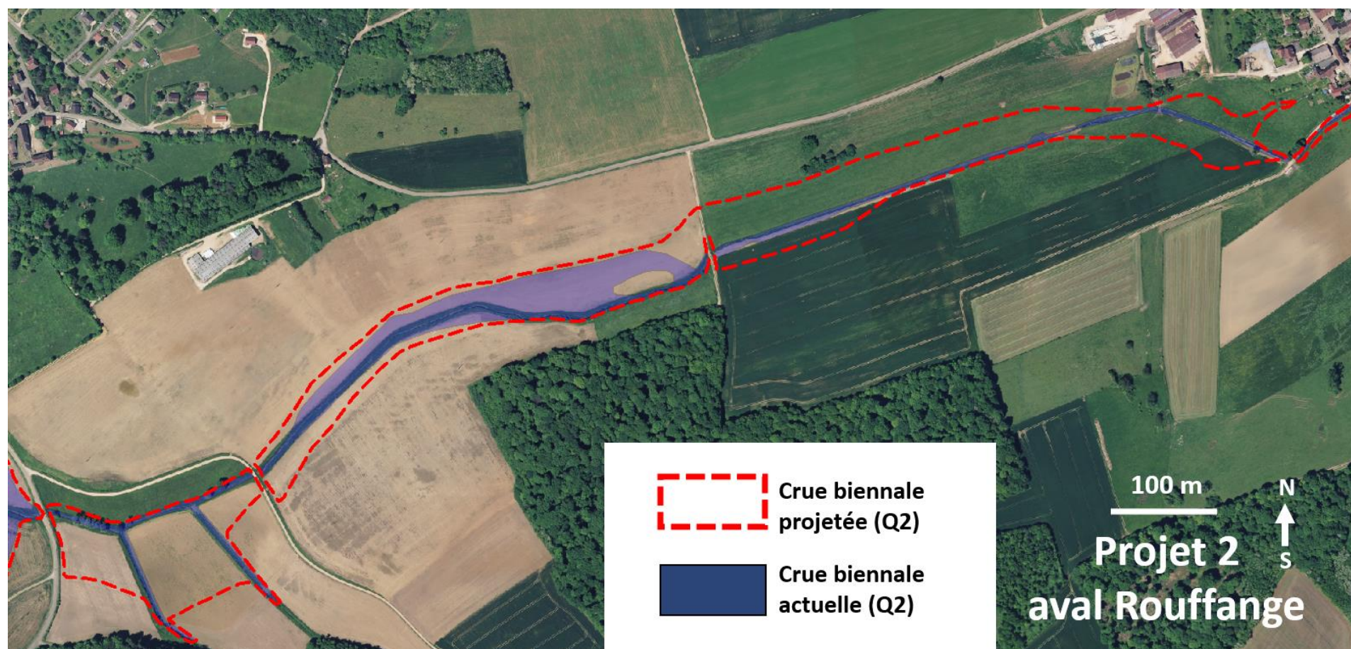
Figure 15.33 : Zones inondables actuelles et futures en crue biennale pour le projet « 2 Aval Rouffange »
