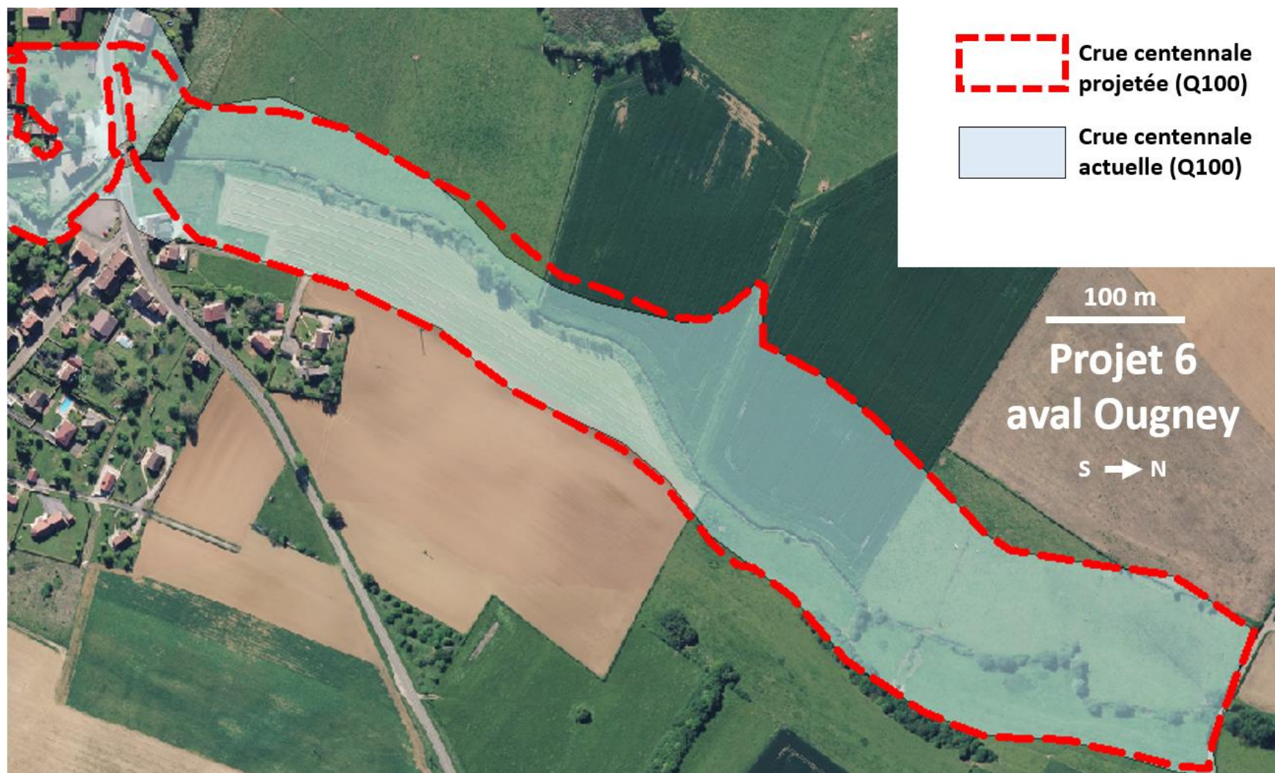
Figure 15.47 : Zones inondables actuelles et futures en crue centennale pour le projet « 6 Aval Ougney »
