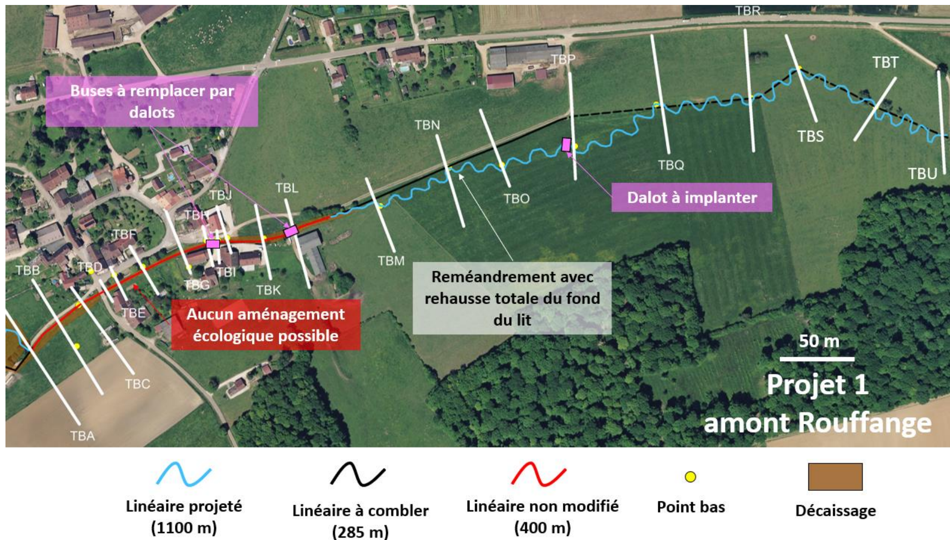
Figure 20.2 : Détails du projet 1 Amont Rouffange
