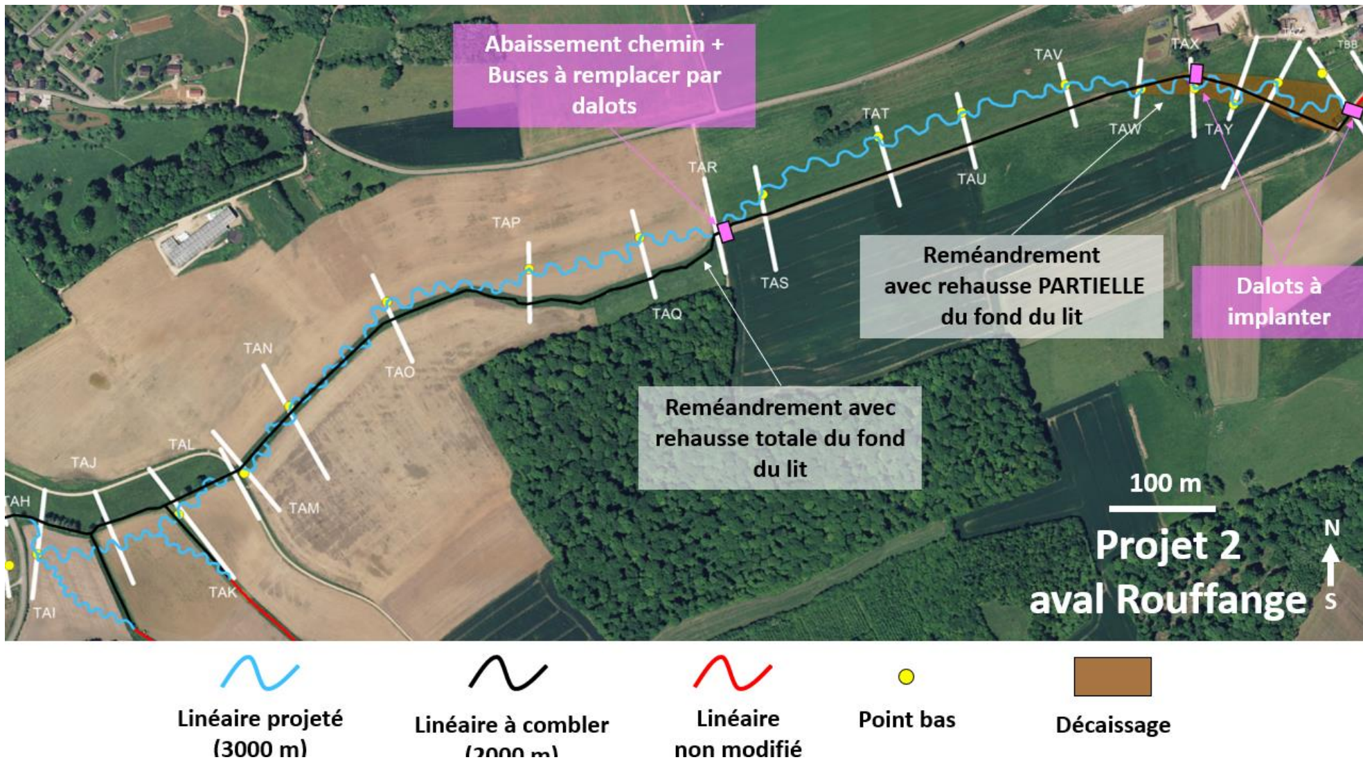
Figure 6.12 : Stratégie de restauration pour le projet « 2 Aval Rouffange »
