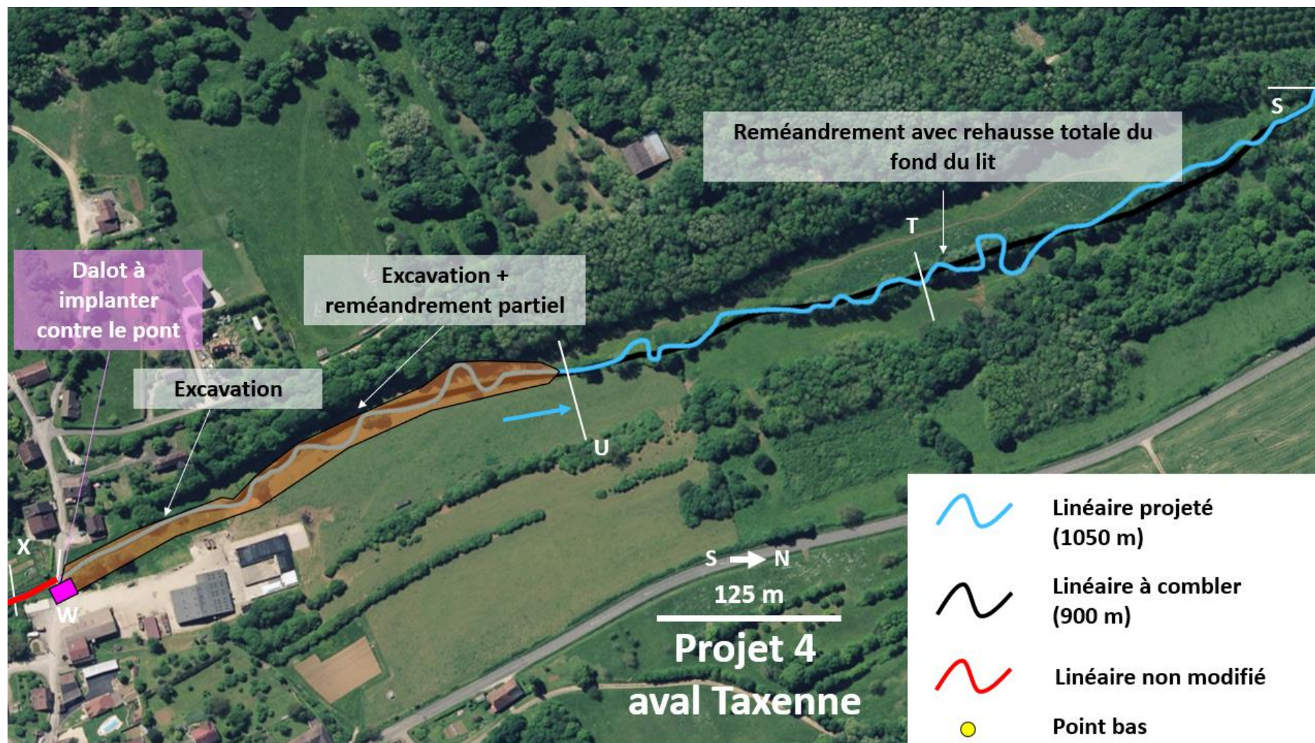
Figure 21.5 : Détails du projet 4 Aval Taxenne
