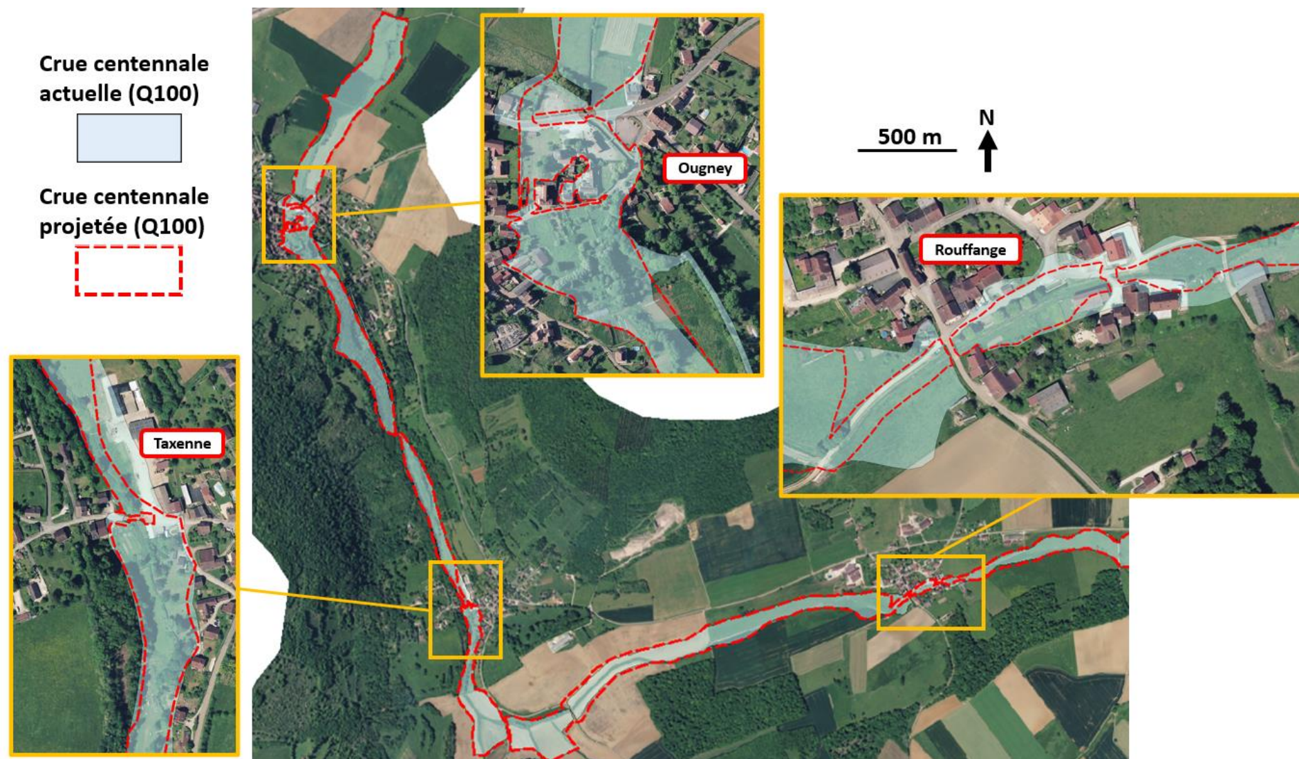
Figure 15.29 : Carte de l'évolution des inondations d'occurrence de crue centennale avant et après le projet.
