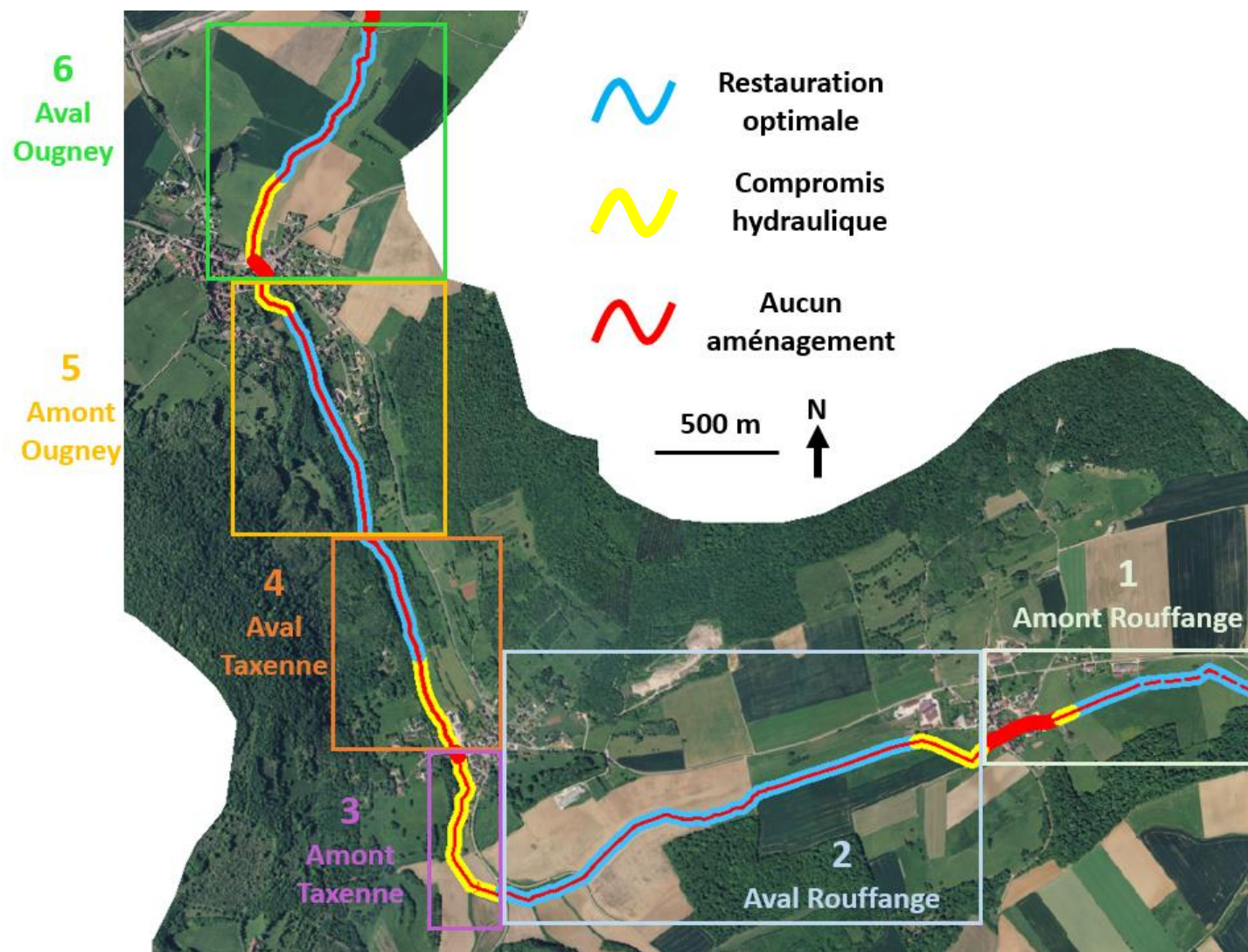
Figure 6.10 : Stratégie de restauration et découpage des 6 sous projets retenus
