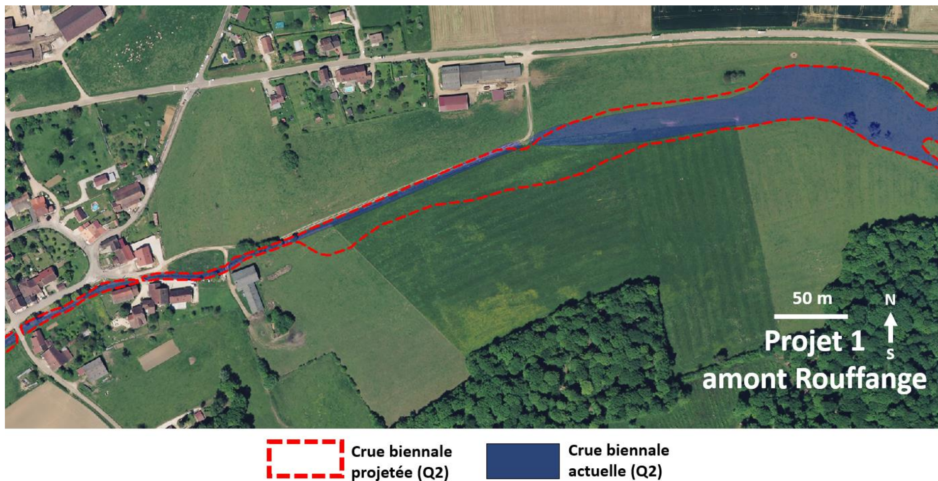
Figure 15.30 : Zones inondables actuelles et futures en crue biennale pour le projet « 1 Amont Rouffange »
