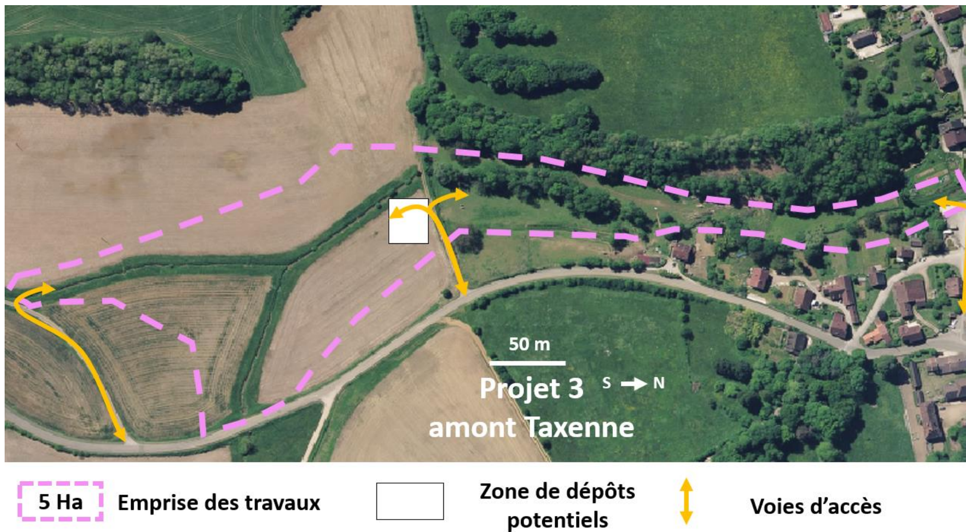
Figure 9.3 : Voies d'accès au chantier (flèches blanches) et zone de dépôts pressenties (carrés blancs) pour le projet « 3 Amont Taxenne ».
