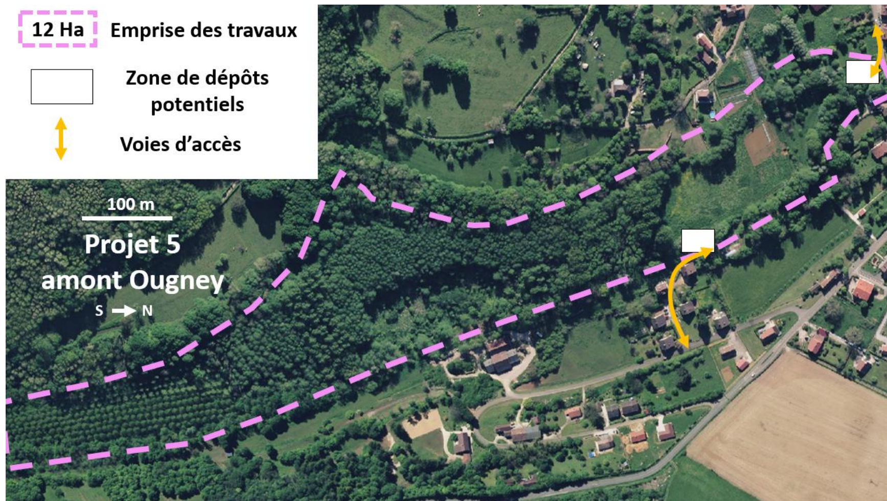
Figure 21.24 : Voies d'accès au chantier (flèches blanches) et zone de dépôts pressenties (carrés blancs) pour le projet « 5 Amont Ougney ».
