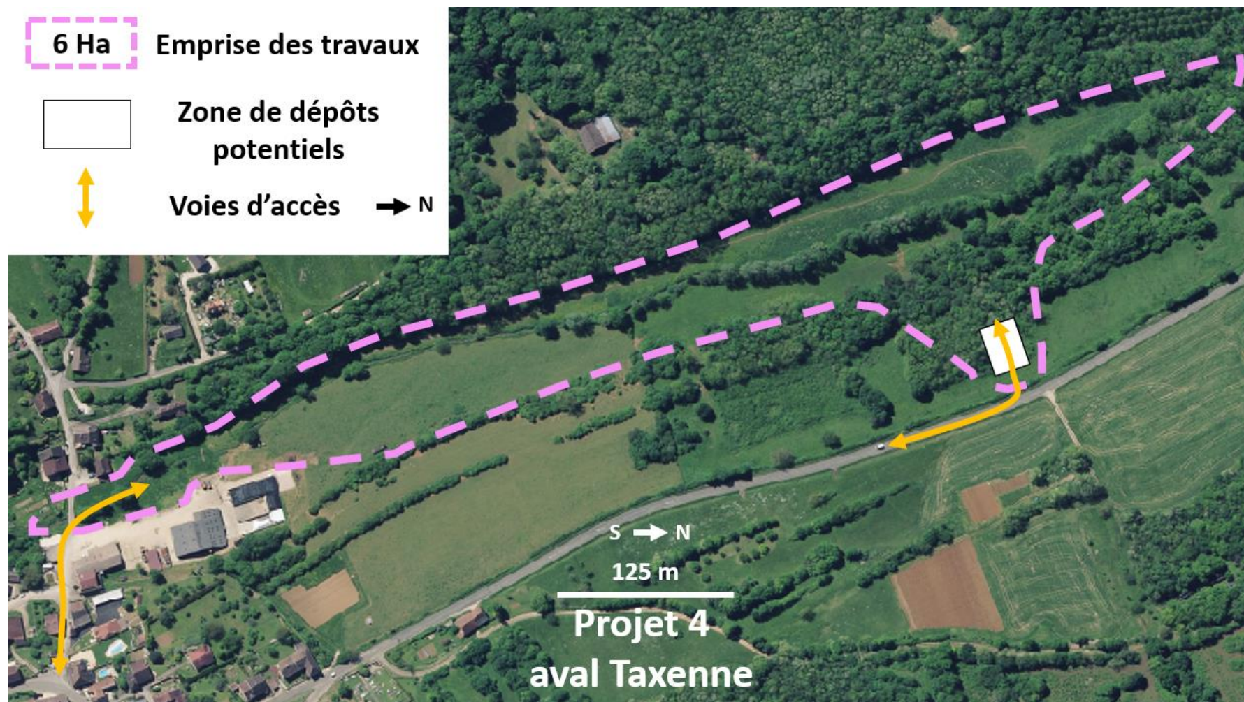
Figure 21.23 : Voies d'accès au chantier (flèches blanches) et zone de dépôts pressenties (carrés blancs) pour le projet « 4 Aval Taxenne ».
