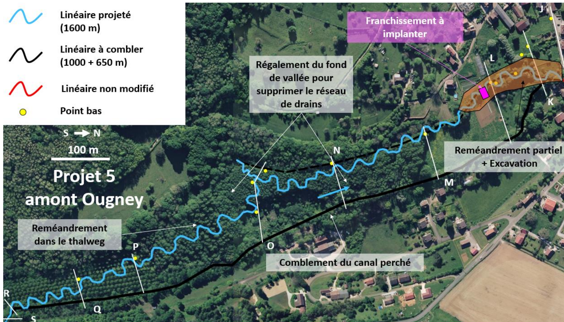
Figure 21.6 : Détails du projet 5 Amont Ougney
