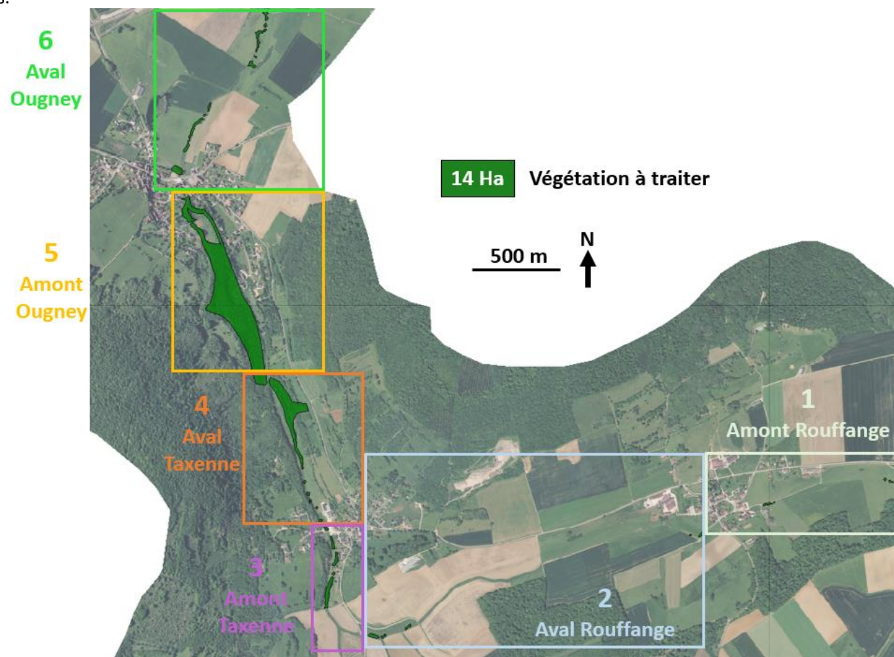
Figure 9.7 : Végétation ligneuse à déboiser pour le besoin des travaux des projets 1 à 6.
