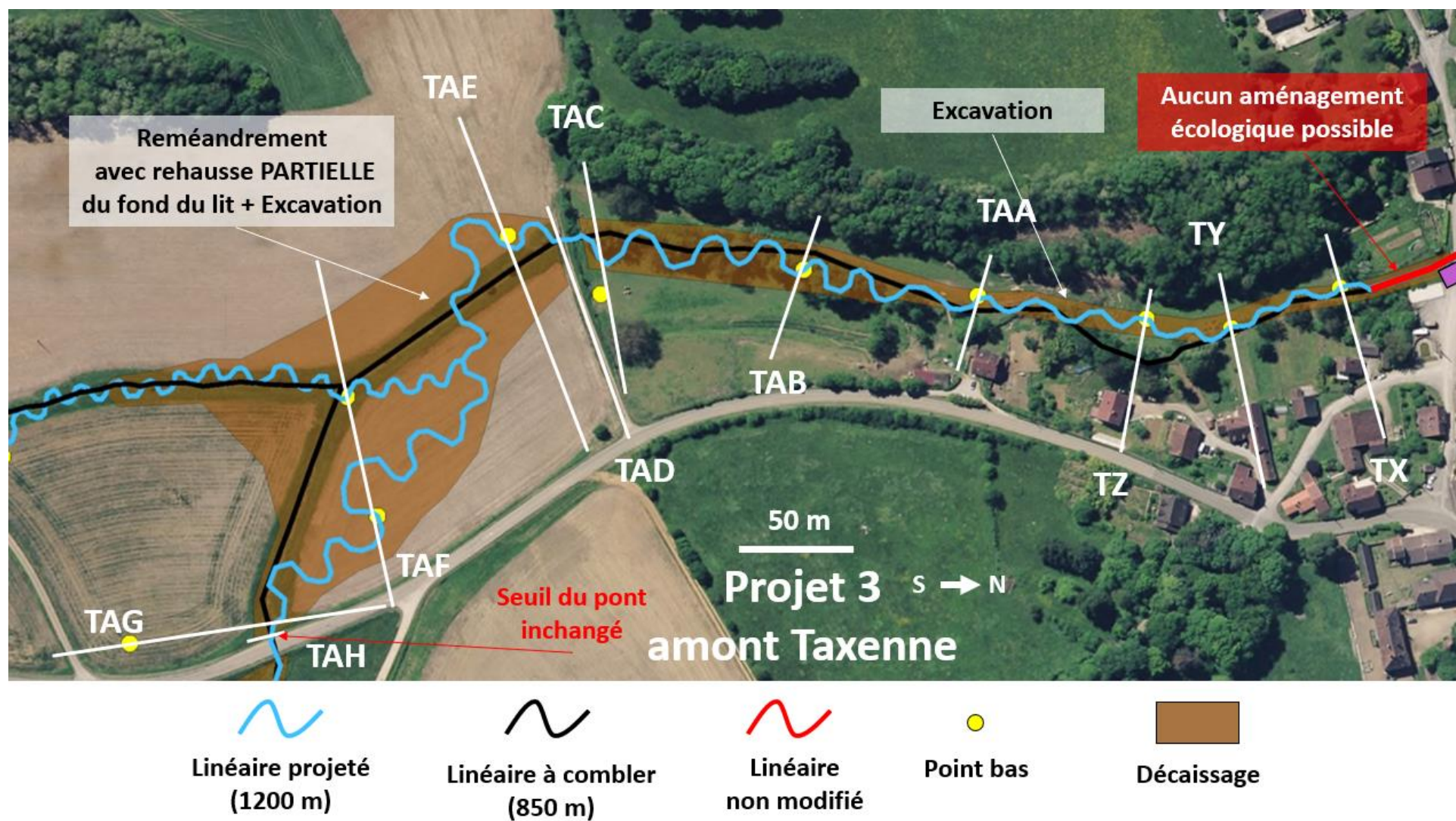
Figure 6.13 : Stratégie de restauration pour le projet « 3 Amont Taxenne »
