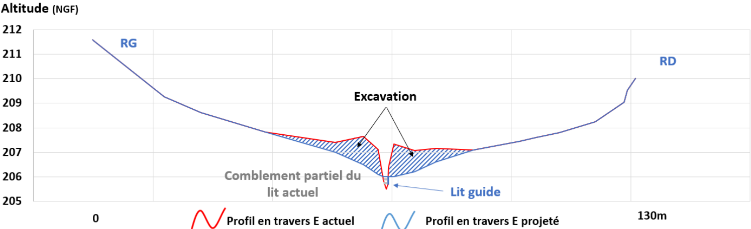
Figure 6.9 : Décaissement du lit moyen en aval immédiat d'Ougney (Profil E) pour ne pas aggraver l'aléa d'inondation
