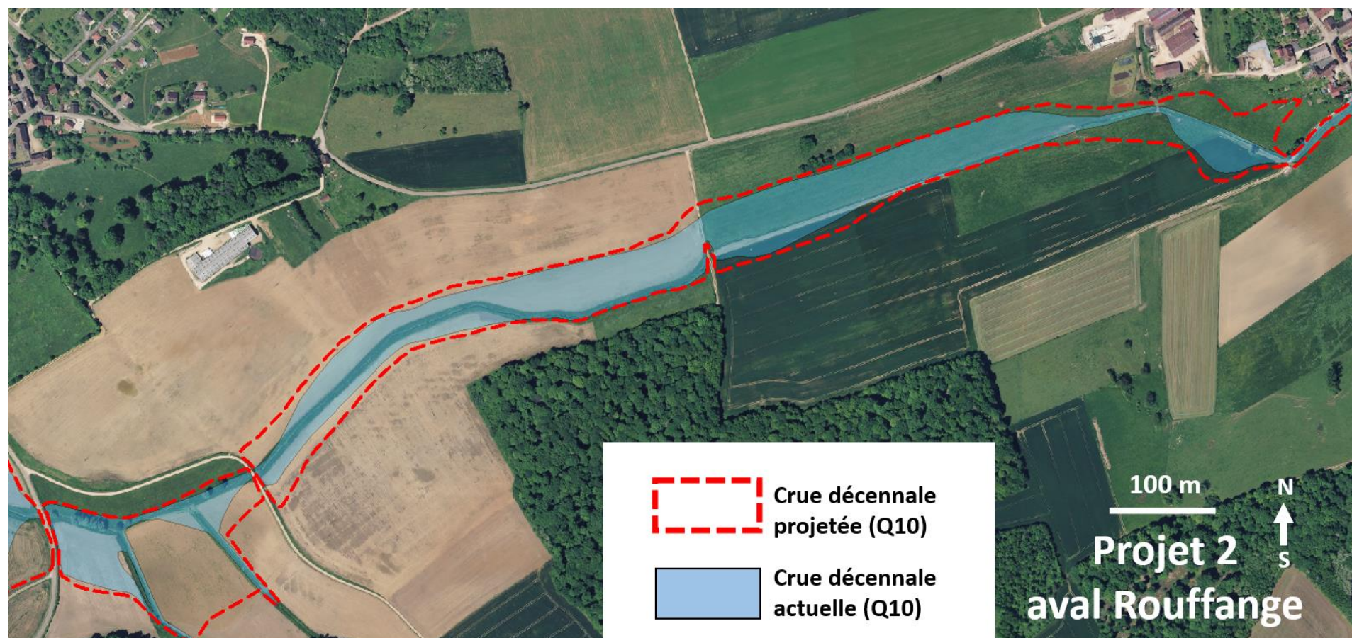
Figure 15.34 : Zones inondables actuelles et futures en crue décennale pour le projet « 2 Aval Rouffange »
