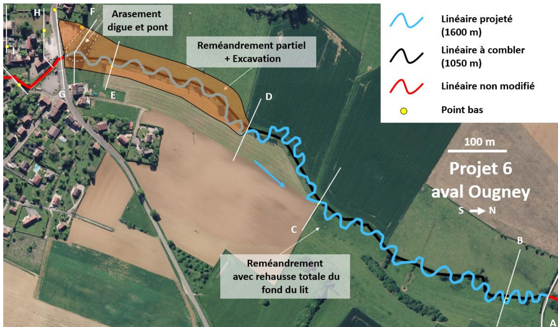
Figure 6.16 : Stratégie de restauration pour le projet «6 Aval Ougney »
