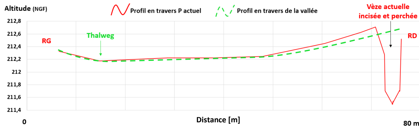
Figure 6.4 : Profil en travers actuel montrant le positionnement perché du lit de la Vèze actuelle.
