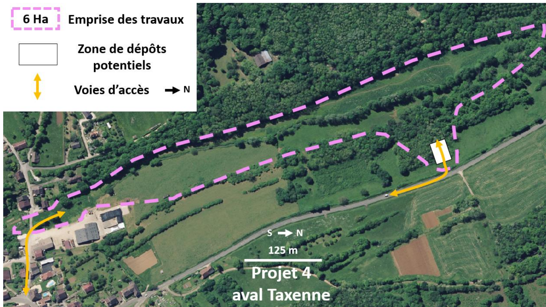
Figure 9.4 : Voies d'accès au chantier (flèches blanches) et zone de dépôts pressenties (carrés blancs) pour le projet « 4 Aval Taxenne ».
