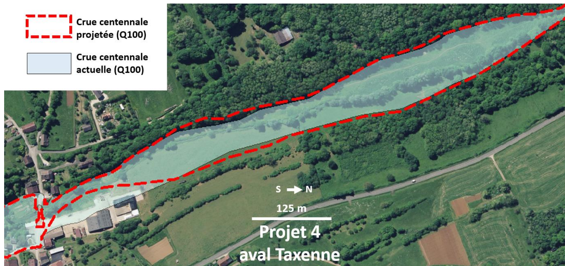
Figure 15.41 : Zones inondables actuelles et futures en crue centennale pour le projet « 4 Aval Taxenne »
