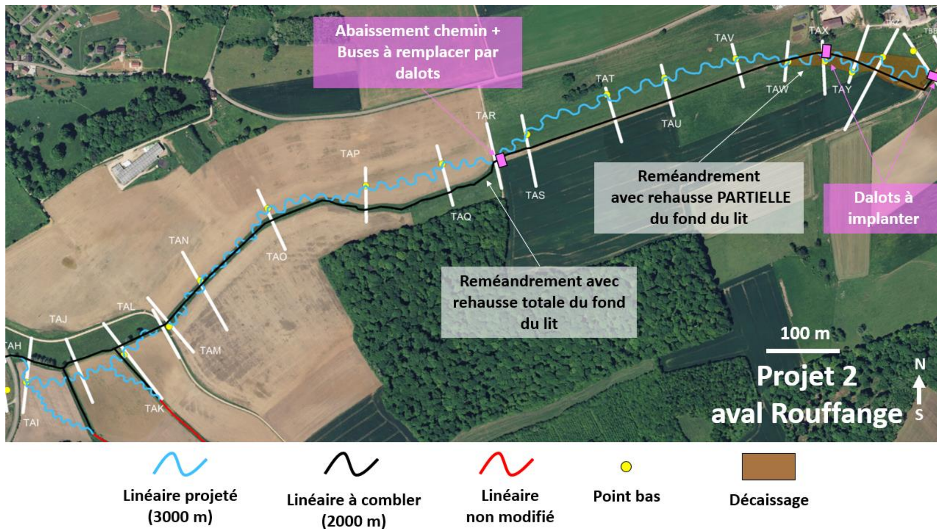
Figure 20.3 : Détails du projet 2 Aval Rouffange
