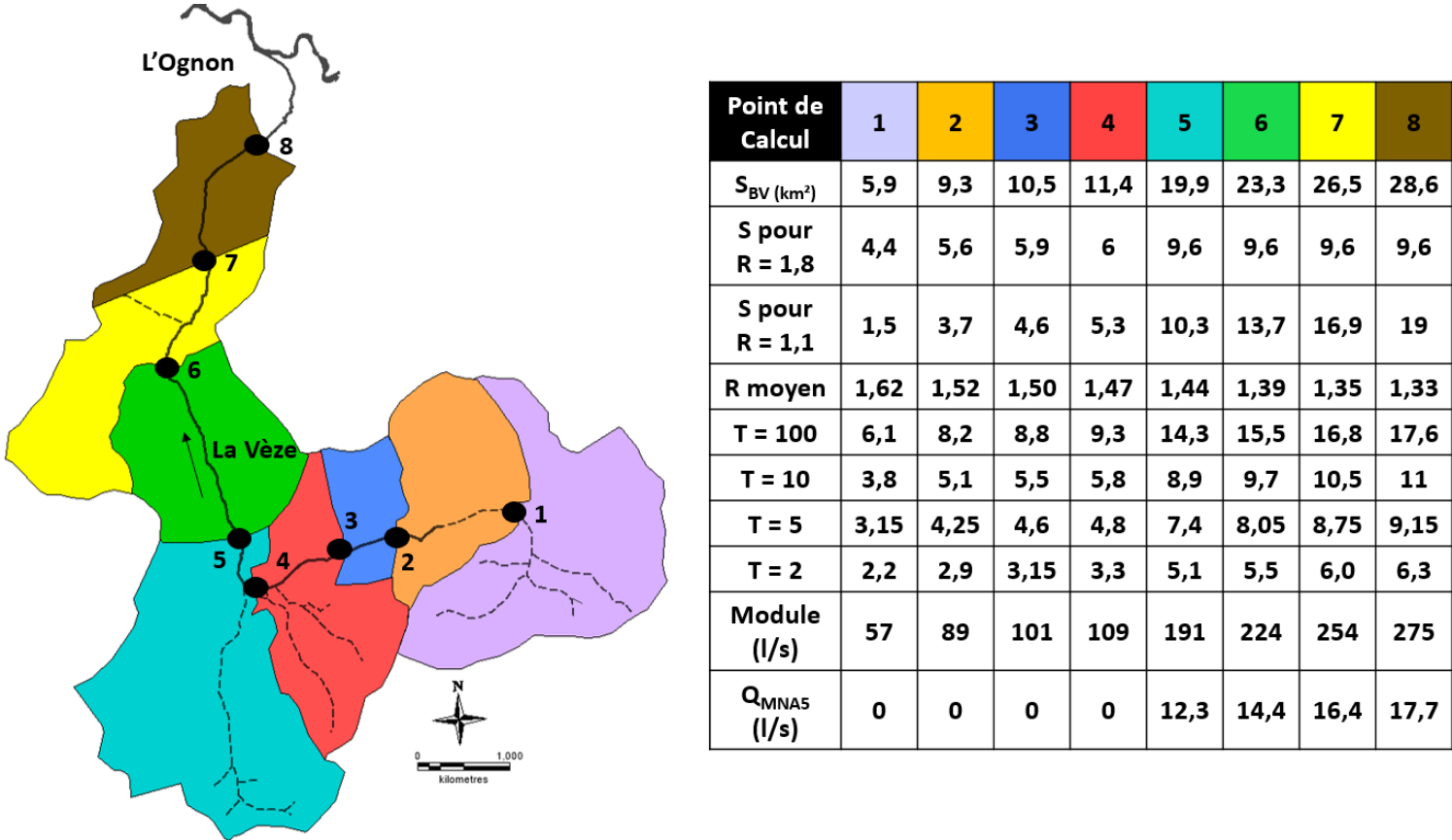
Figure 15.3 : Débits extrapolés pour les sous-bassins de la Vèze d'Ougney
