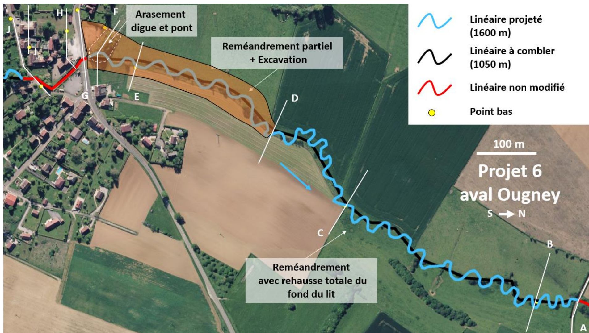
Figure 21.7 : Détails du projet 6 Aval Ougney
