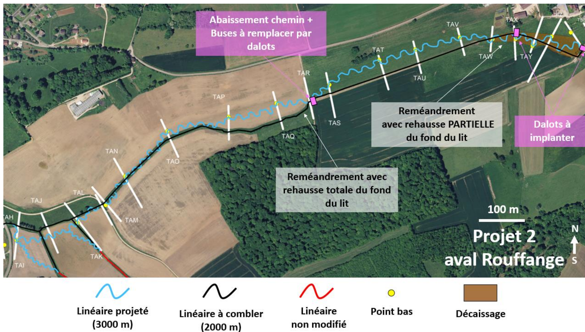
Figure 21.3 : Détails du projet 2 Aval Rouffange
