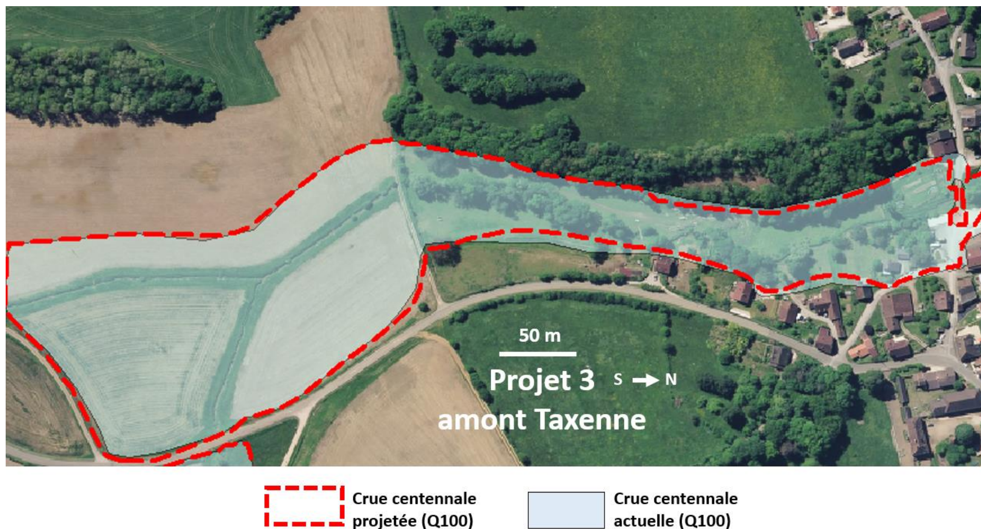
Figure 15.38 : Zones inondables actuelles et futures en crue centennale pour le projet « 3 Amont Taxenne »
