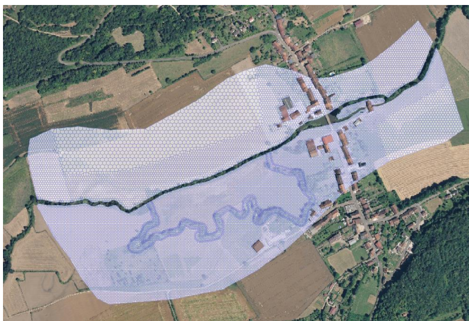
Fig. 22. Présentation du maillage du modèle
