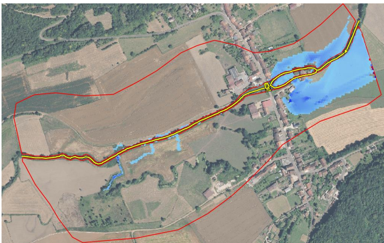
Fig. 26. Enveloppe inondable – Q5
