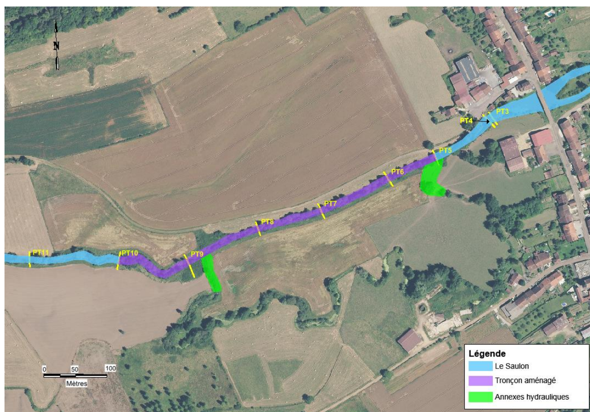
Fig. 60. Scénario 3 : Tracé en plan
