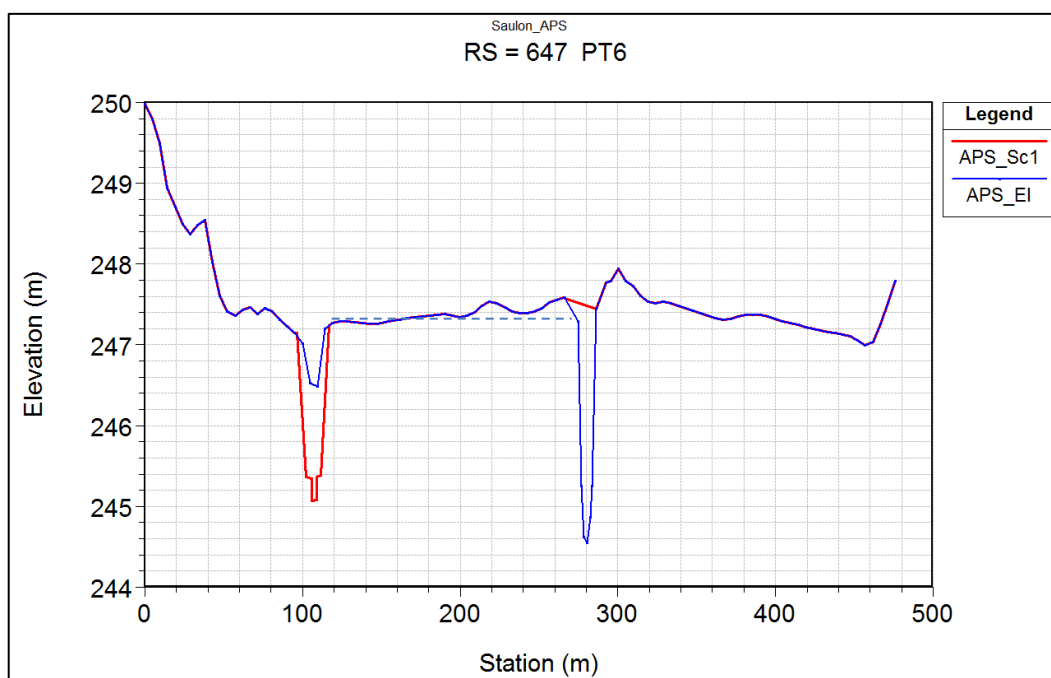
Fig. 50. Scénario 1 - Coupe en travers - PT6
