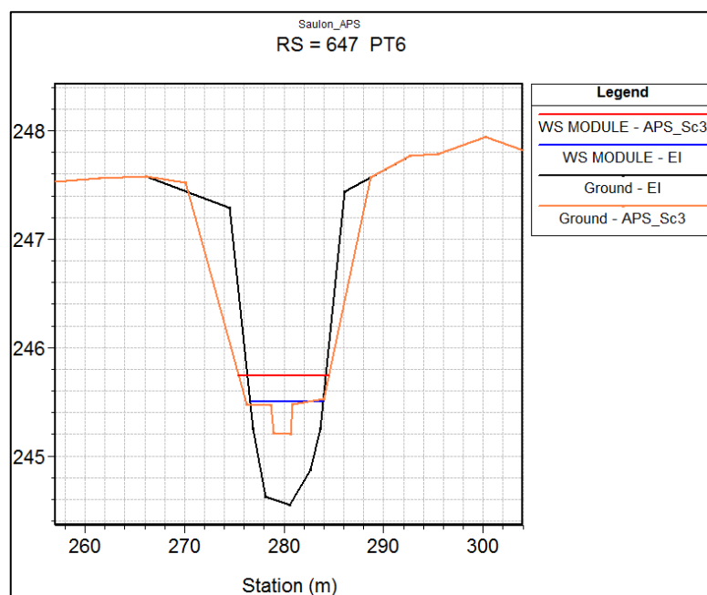
Fig. 64. Exemple de coupe en travers du scénario 3 (Ne - MODULE)
