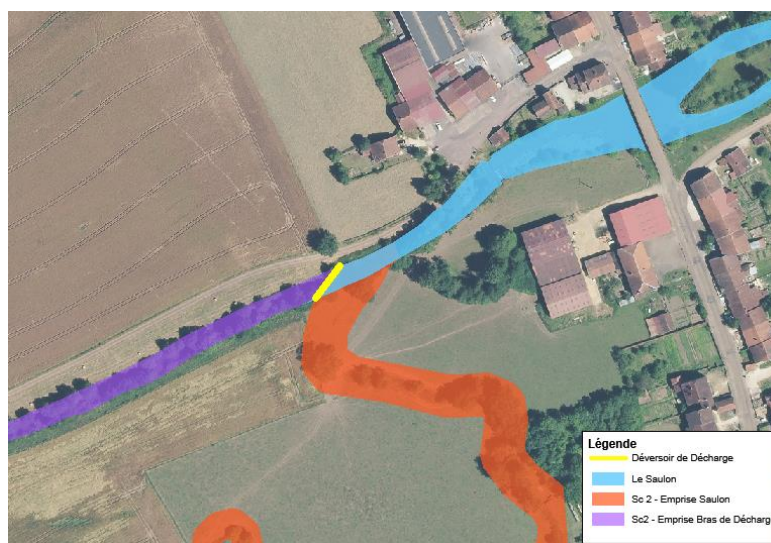
Fig. 57. Localisation de l'ouvrage de décharge
