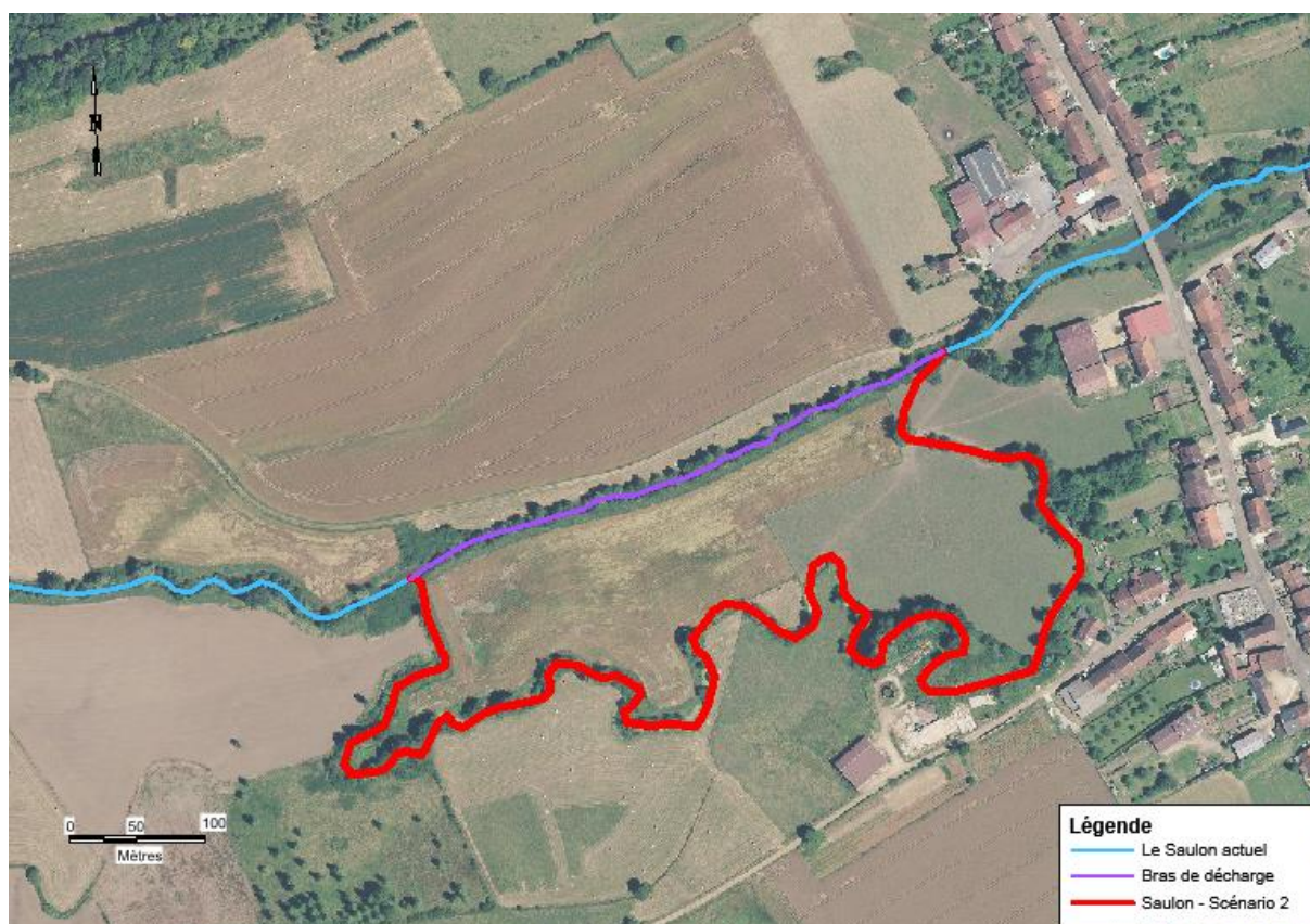
Fig. 55. Scénario 2 : Tracé en plan
