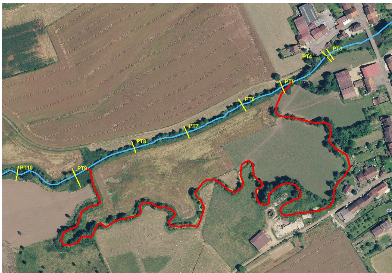
Fig. 48. Scénario 1 : Tracé en plan
