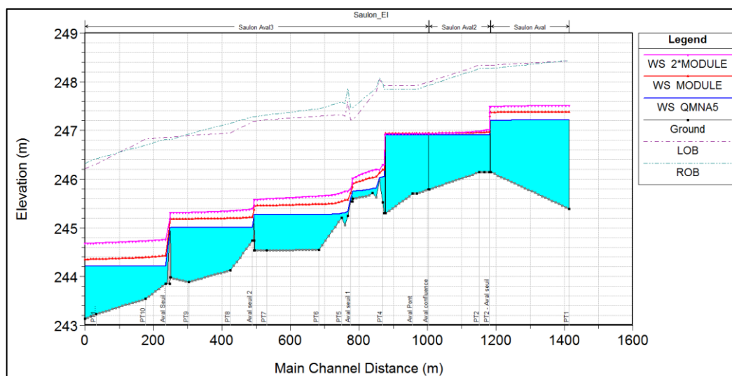
Fig. 24. Influence des ouvrages pour différents débits
