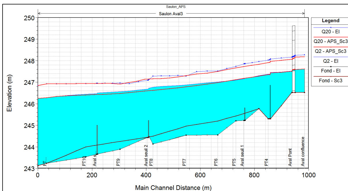
Fig. 63. Impact de la ligne d'eau en crue – Sc3
