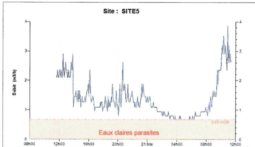
Graphique 1 : débit de temps sec caractéristique théorique
