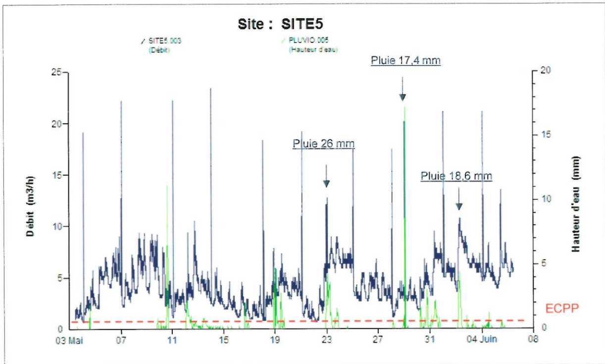
Graphique 5 : Courbe de débit en fonction de la pluviométrie – site 5 (Traversière)
