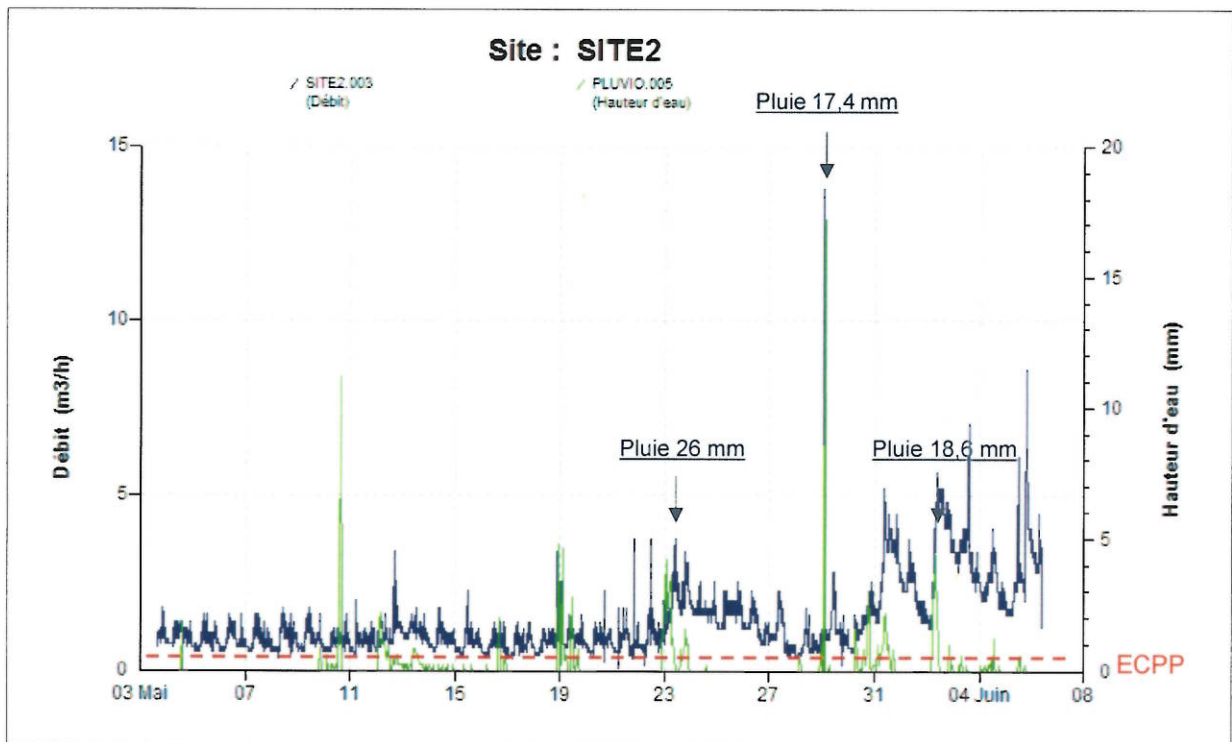
Graphique 2 : Courbe de débit en temps sec – site 2 (Petitmagny)
