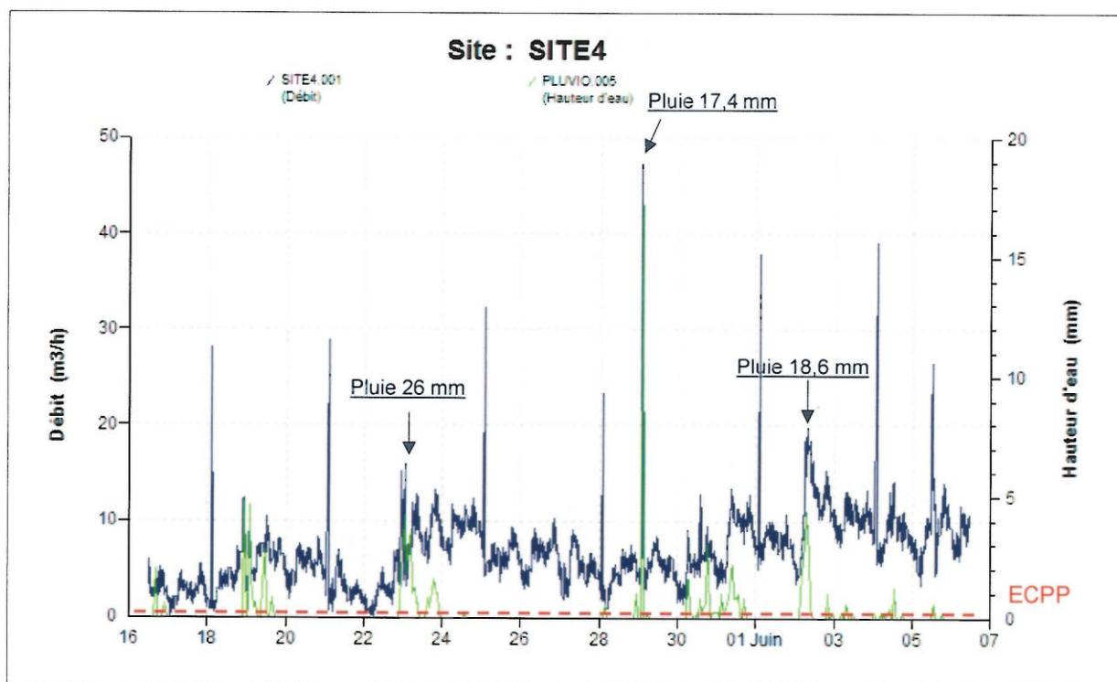
Graphique 4 : Courbe de débit en fonction de la pluviométrie – site 4 (Rue d'Eloie)
