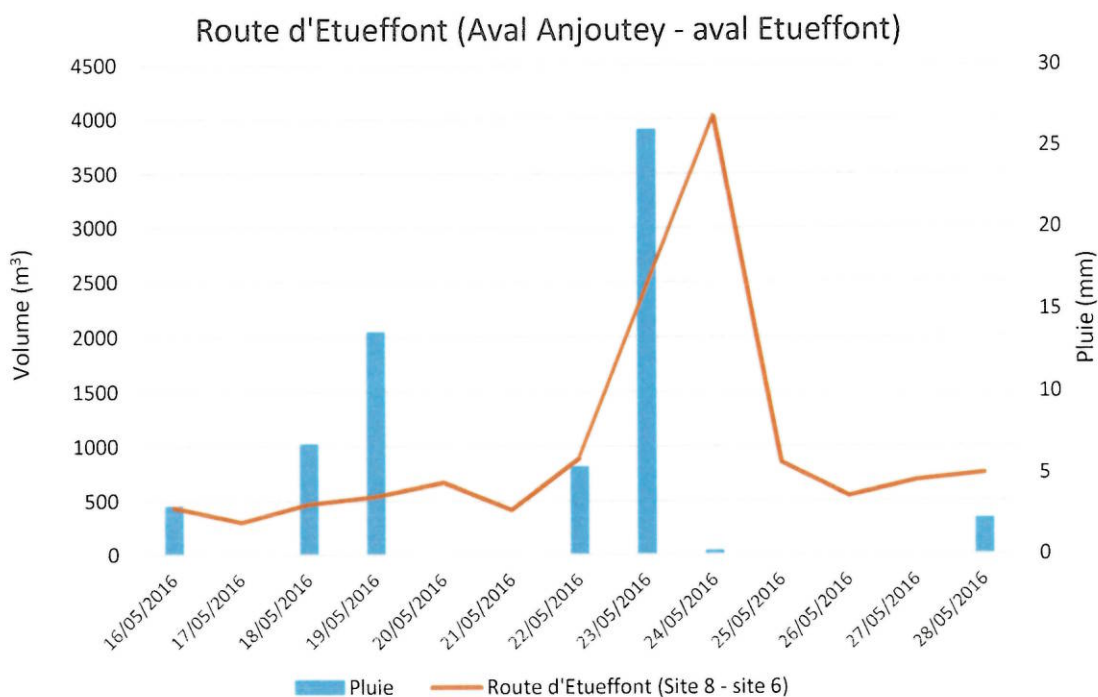
Graphique 10 : Courbe de débit en fonction de la pluviométrie – Route d'Etueffont
