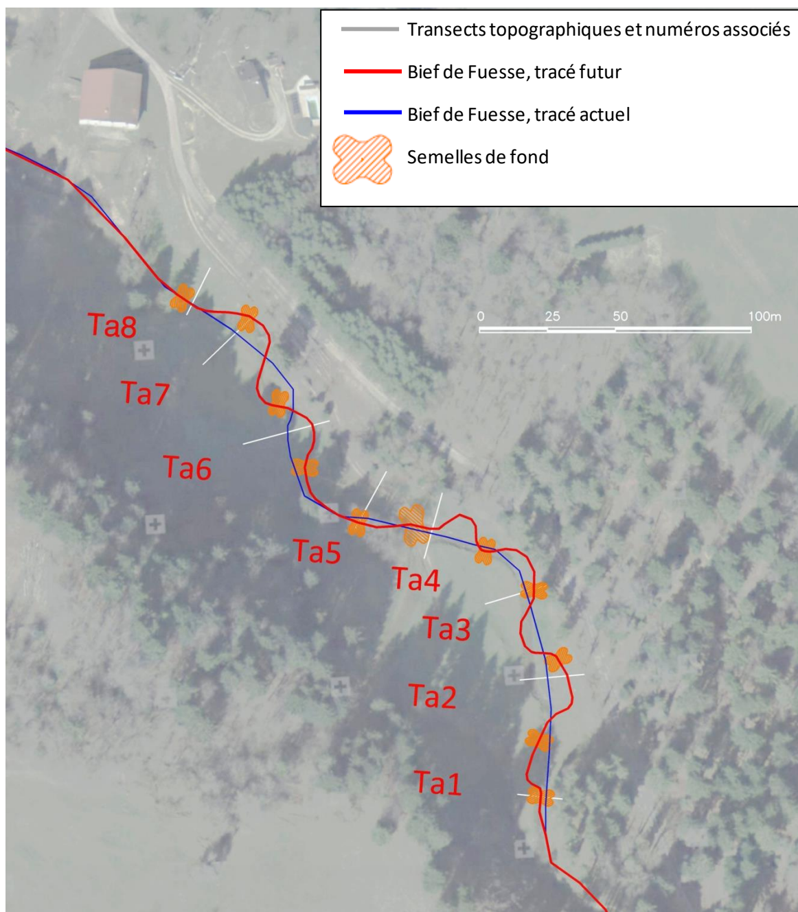
Figure 38 : Tracé actuel et projeté du bief de Fuesse sur le secteur médian.
