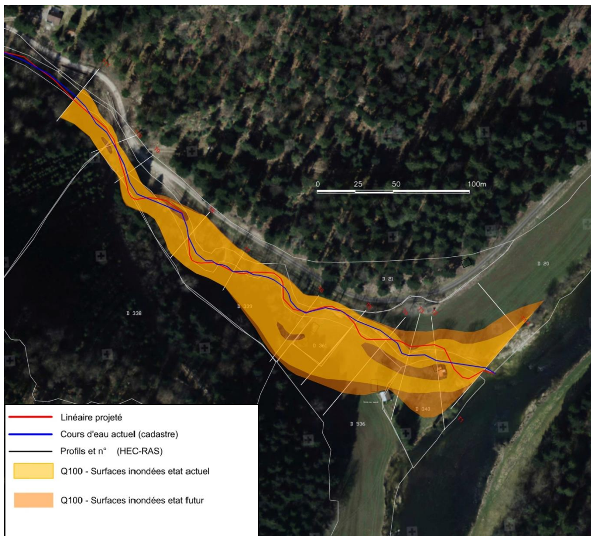
Figure 51: Fuesse aval - zone inondable en crue centennales avant et après travaux.
