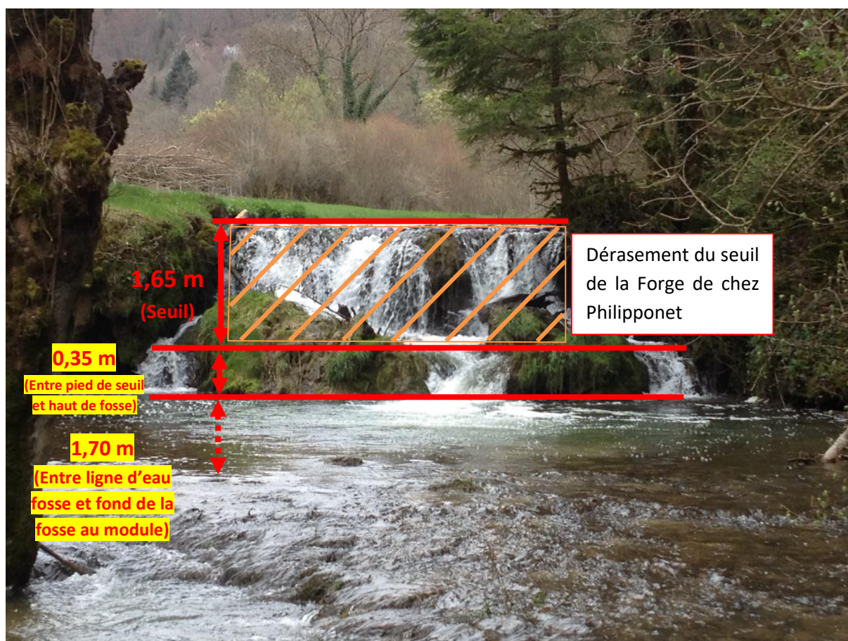
Figure 37 : Dérasement du seuil de la Forge de chez Philipponet.
