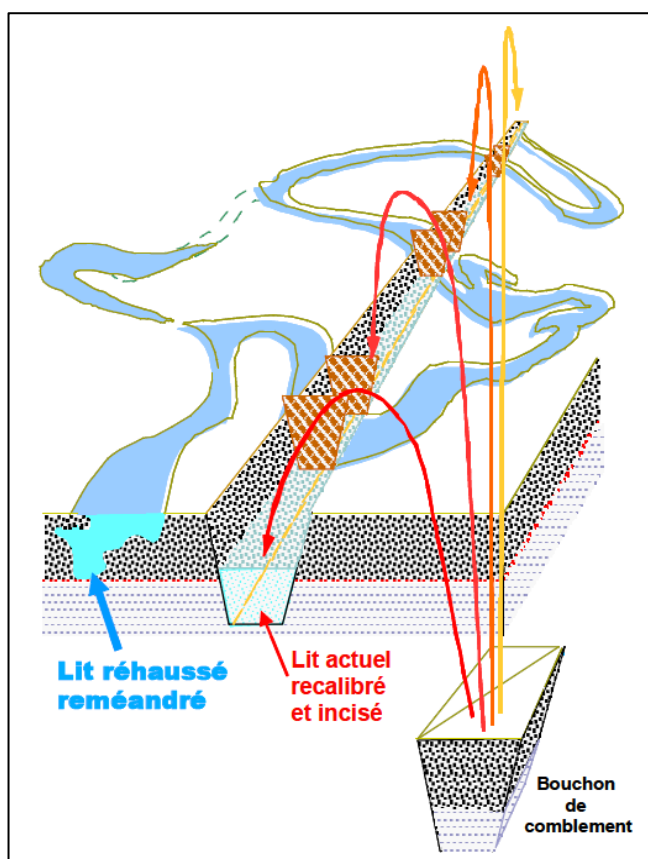
Figure 26: Principe du reméandrement.
