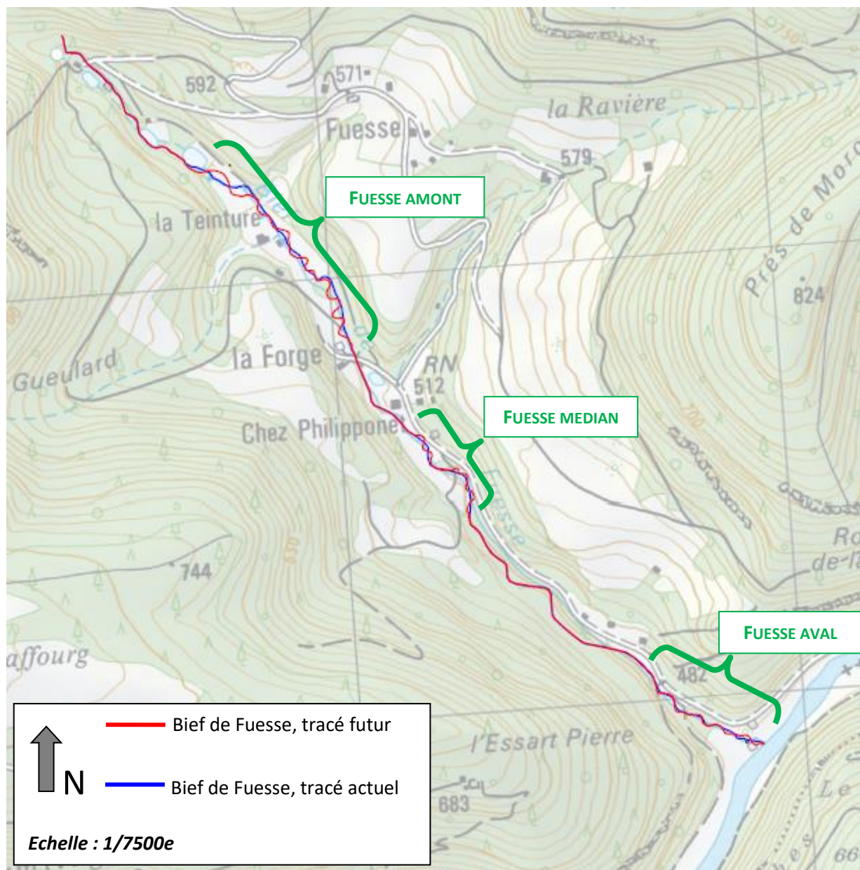
Figure 33: Secteur d'intervention et évolution du profil en long du Bief de Fuesse avant et après travaux de restauration.
