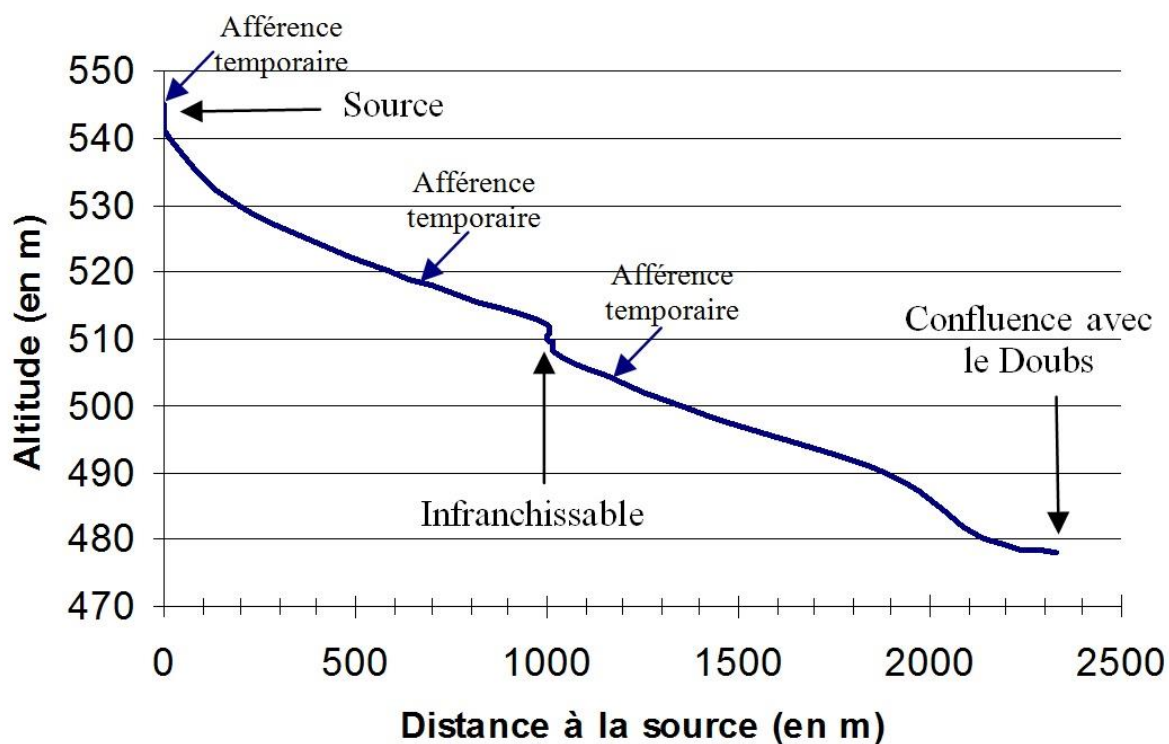
Figure 3: Profil longitudinal du Bief de Fuesse.
