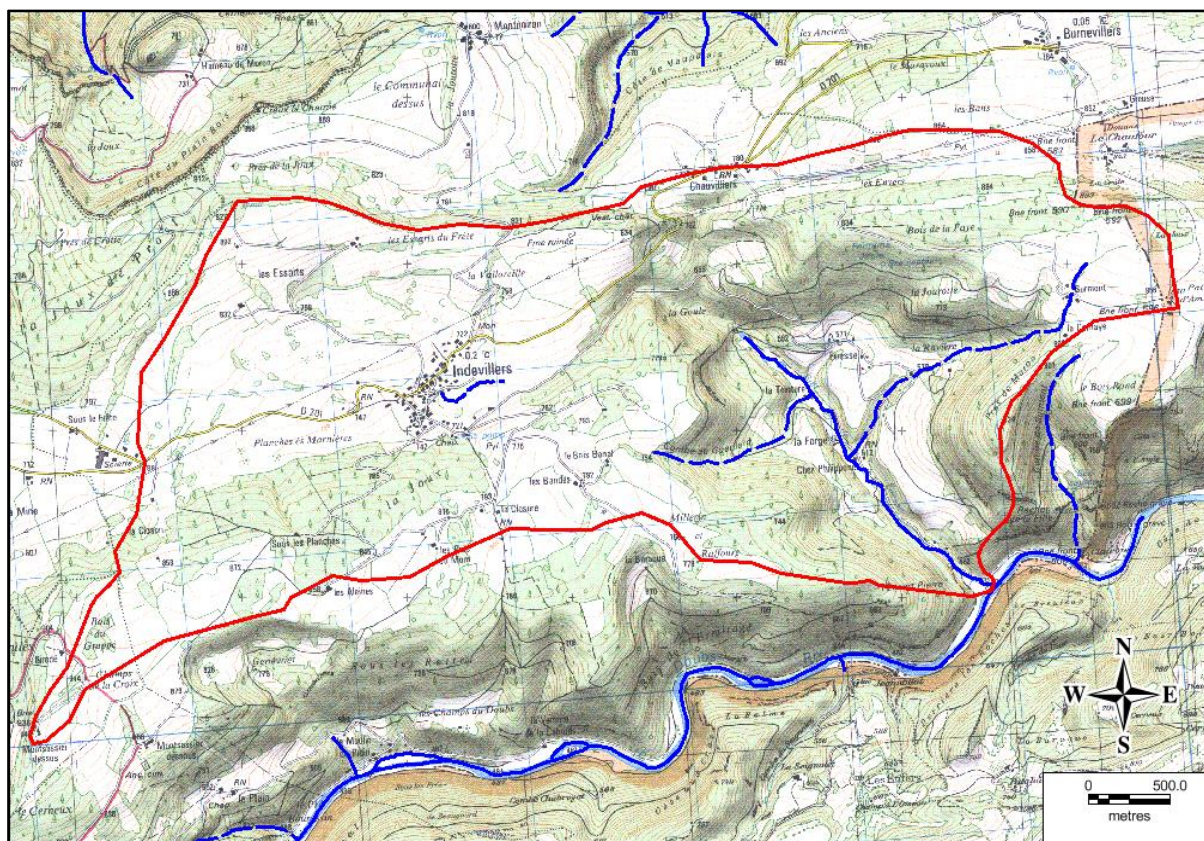
Figure 2: Le Bief de Fuesse et son bassin versant.
