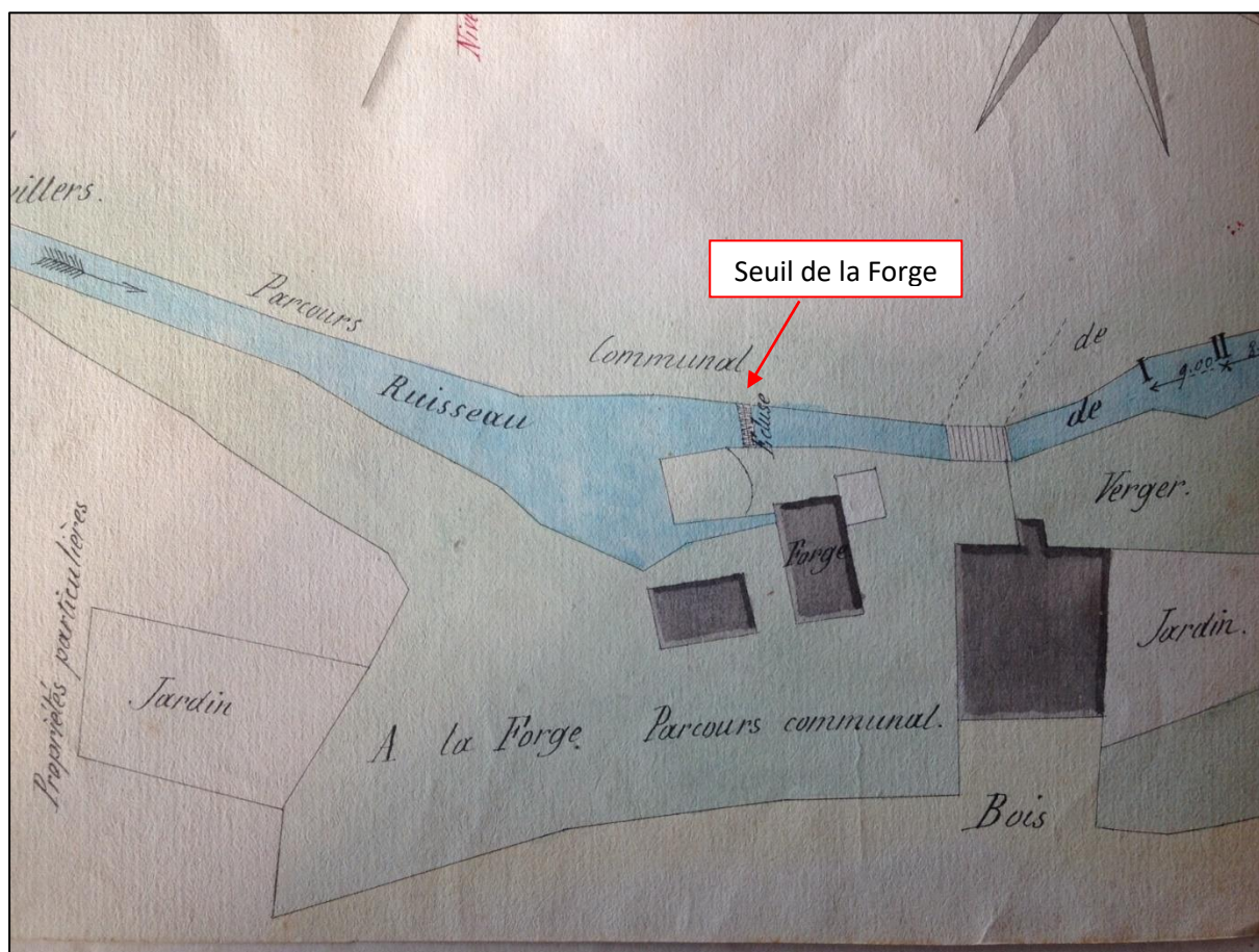
Figure 31: Plan des lieux aux abords du seuil de la Forge nommé écluse dans un dossier de 1858 (demande de mise en place d'une machine à battre et création d'un autre seuil (empilement de pierres sèches couronnés d'une pièce de bois) en aval de la Forge.
