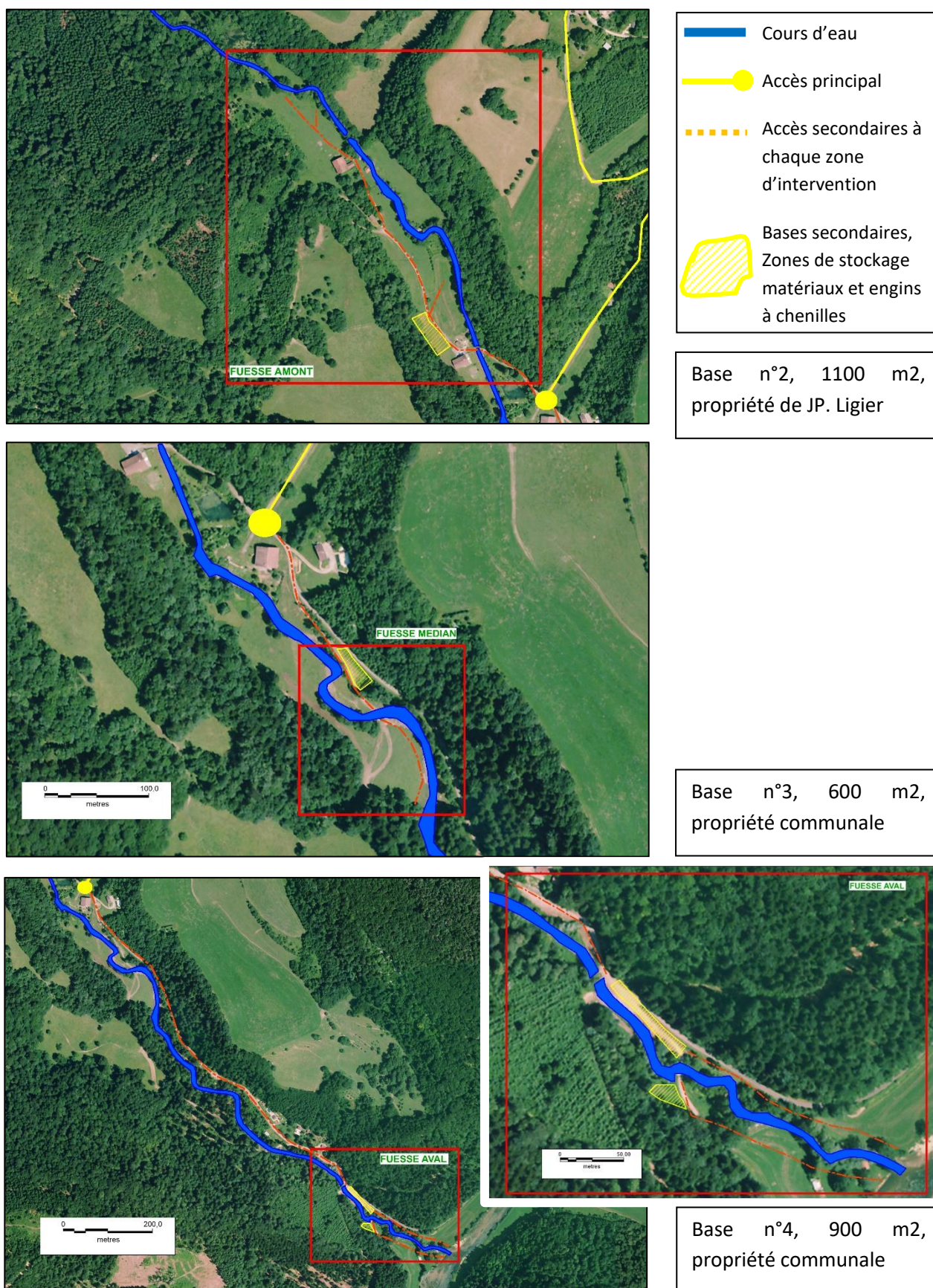
Figure 53: Accès secondaires des engins et zones de stockage des matériaux et engins à chenilles (pelleteuses, ...). Note : la zone humide du secteur aval sera balisée afin d'éviter tout débordement par l'entreprise de génie civil.
