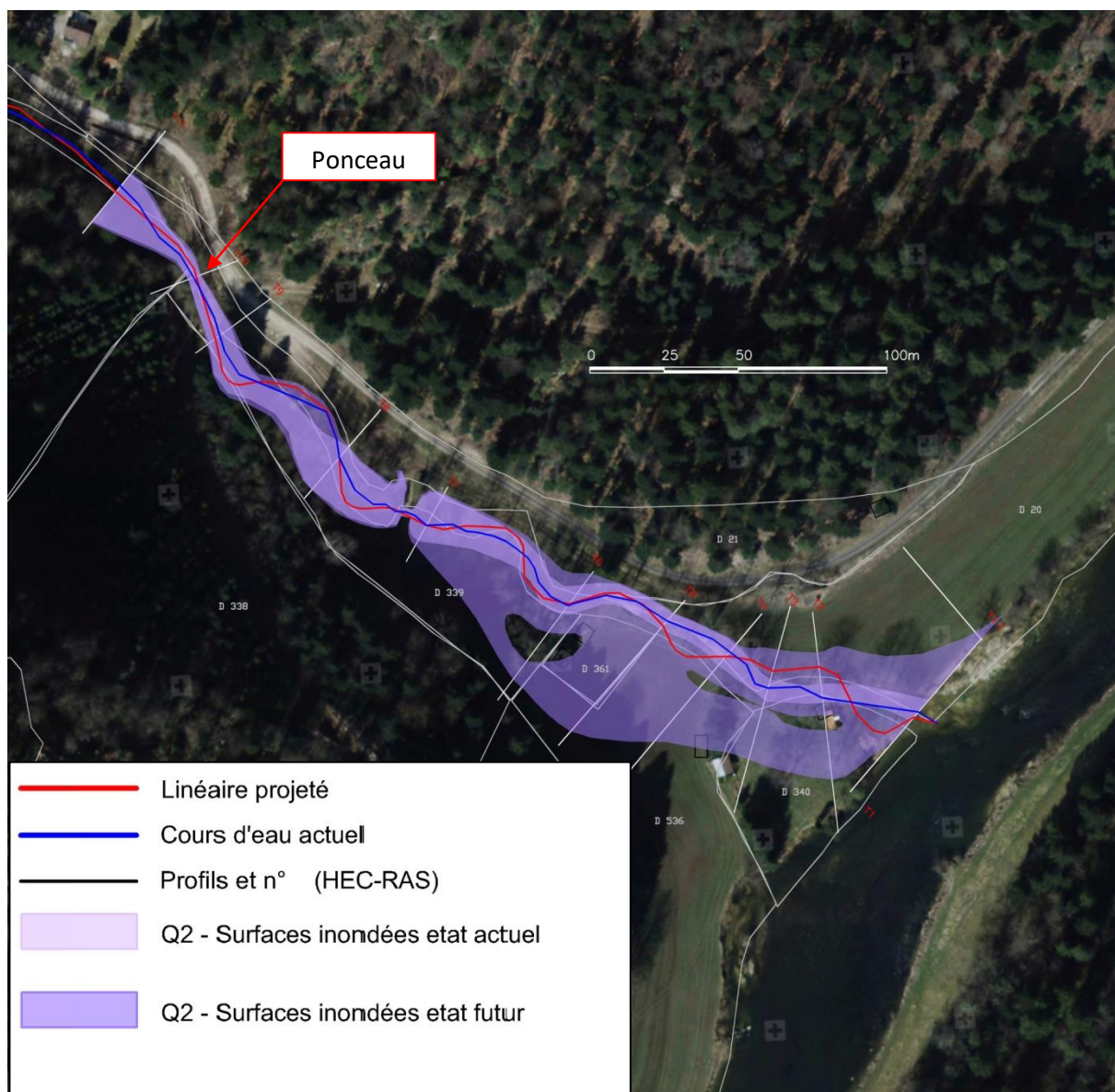
Figure 47: Fuesse aval - zone inondable en crue biennale avant et après travaux.
