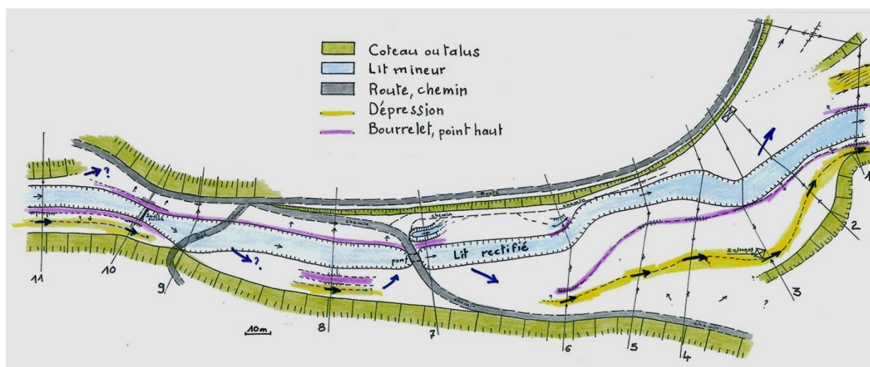
Figure 42: Bief de Fuesse aval- Analyse morphologique.
