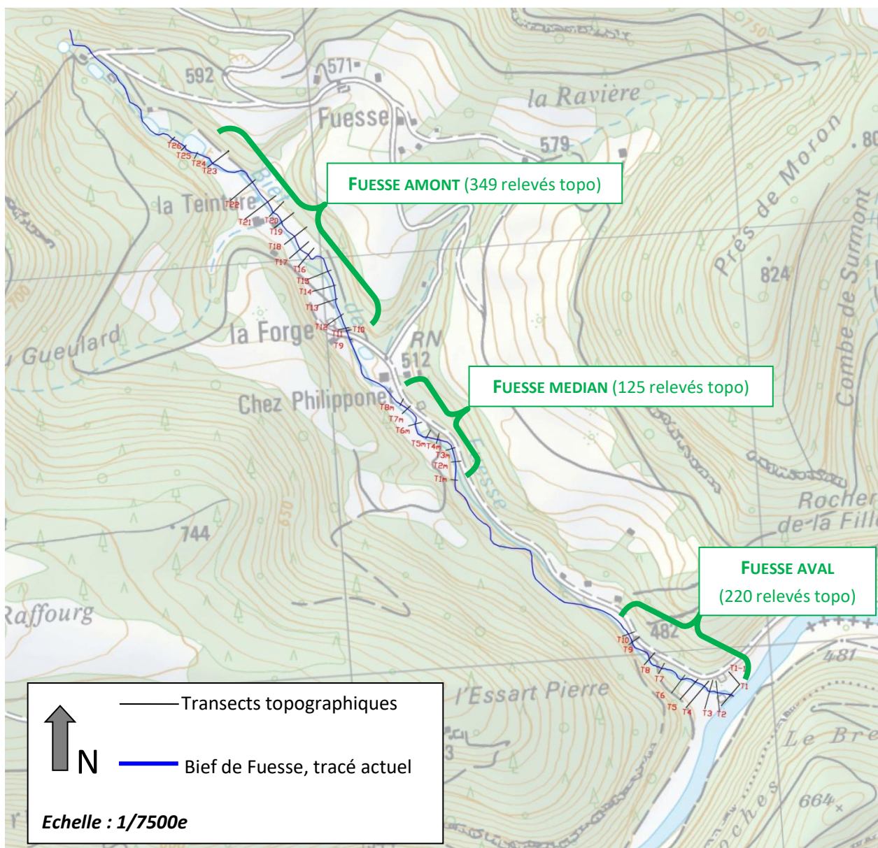
Figure 28: Localisation des transects de relevés topographiques et secteurs d'intervention.
