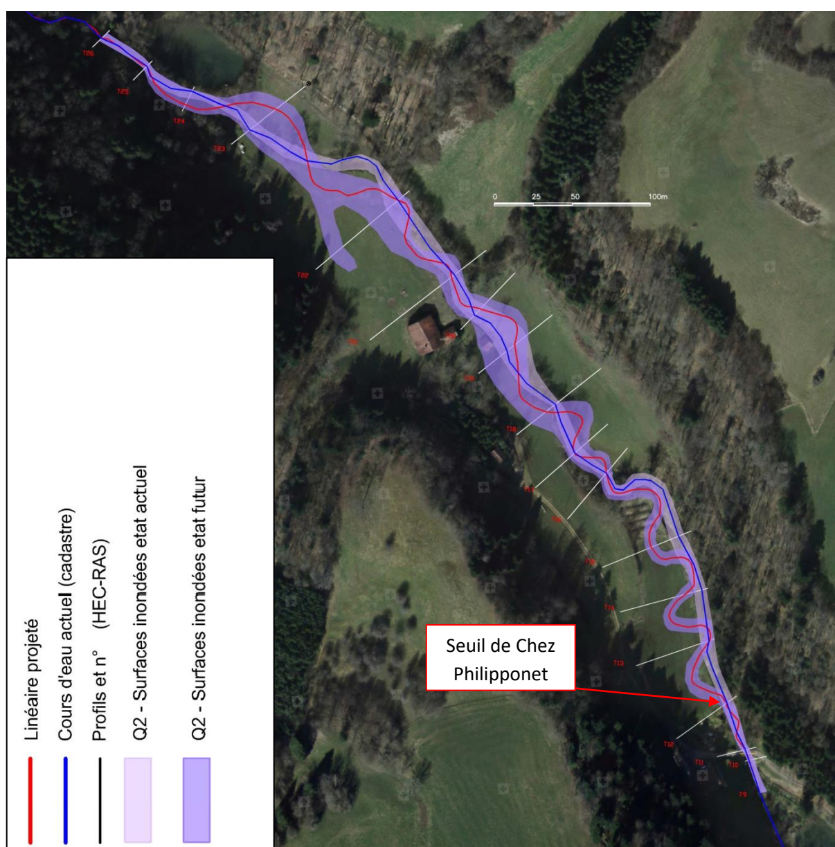
Figure 45: Fuesse amont - zone inondable en crue biennale avant et après travaux.
