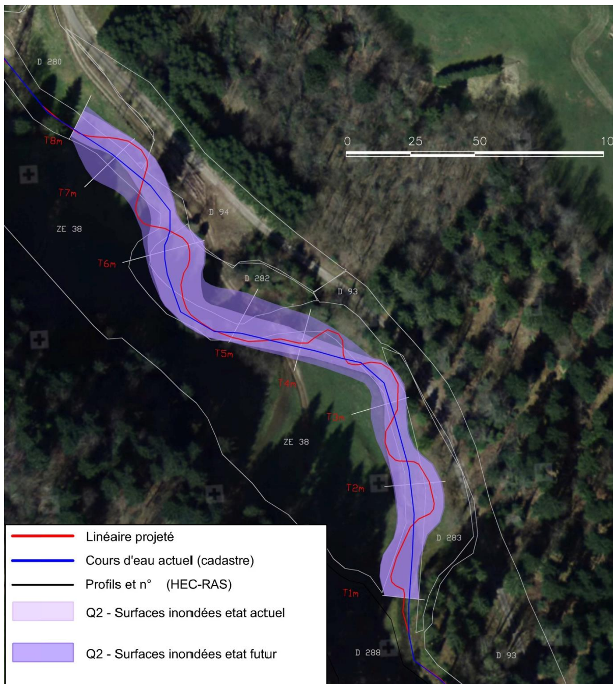
Figure 46: Fuesse médian - zone inondable en crue biennale avant et après travaux.
