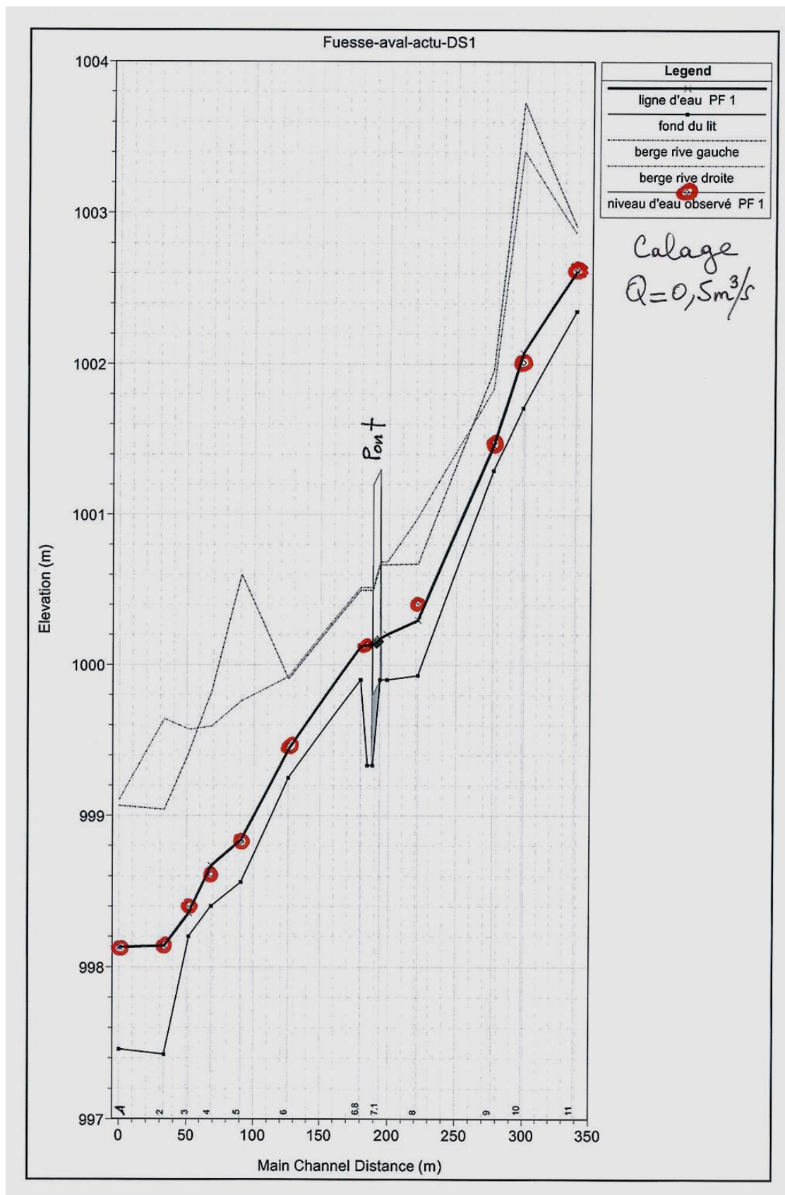
Figure 43: Bief de Fuesse aval - Calage
