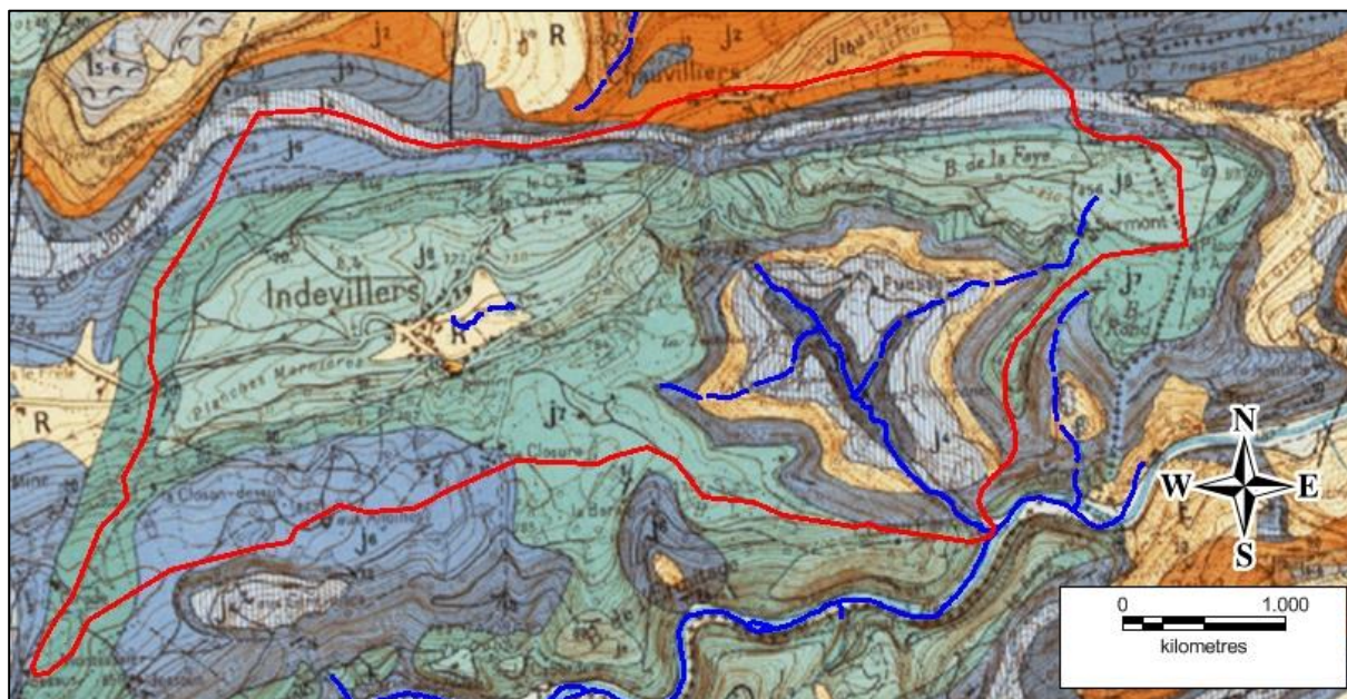
Figure 5: Contexte géologique du bassin versant du Bief de Fuesse.
