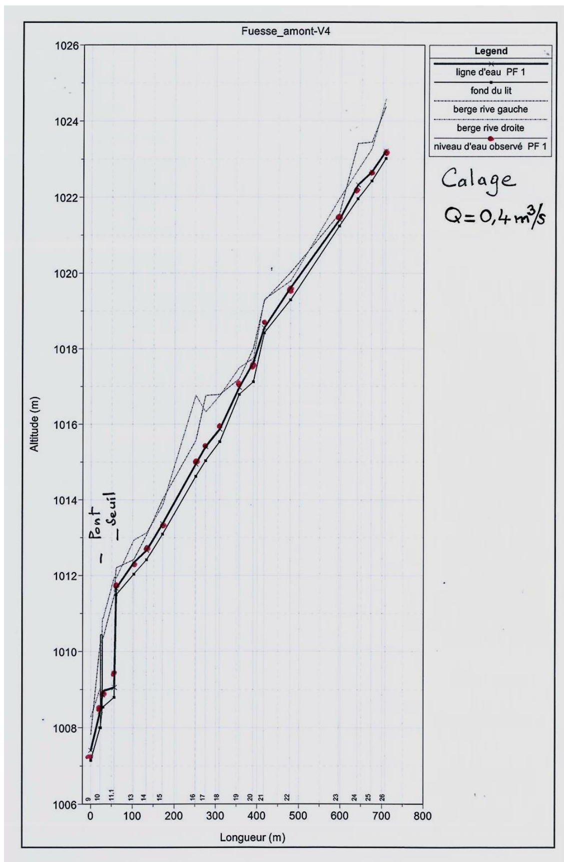
Figure 36 : Bief de Fuesse amont - Calage.
