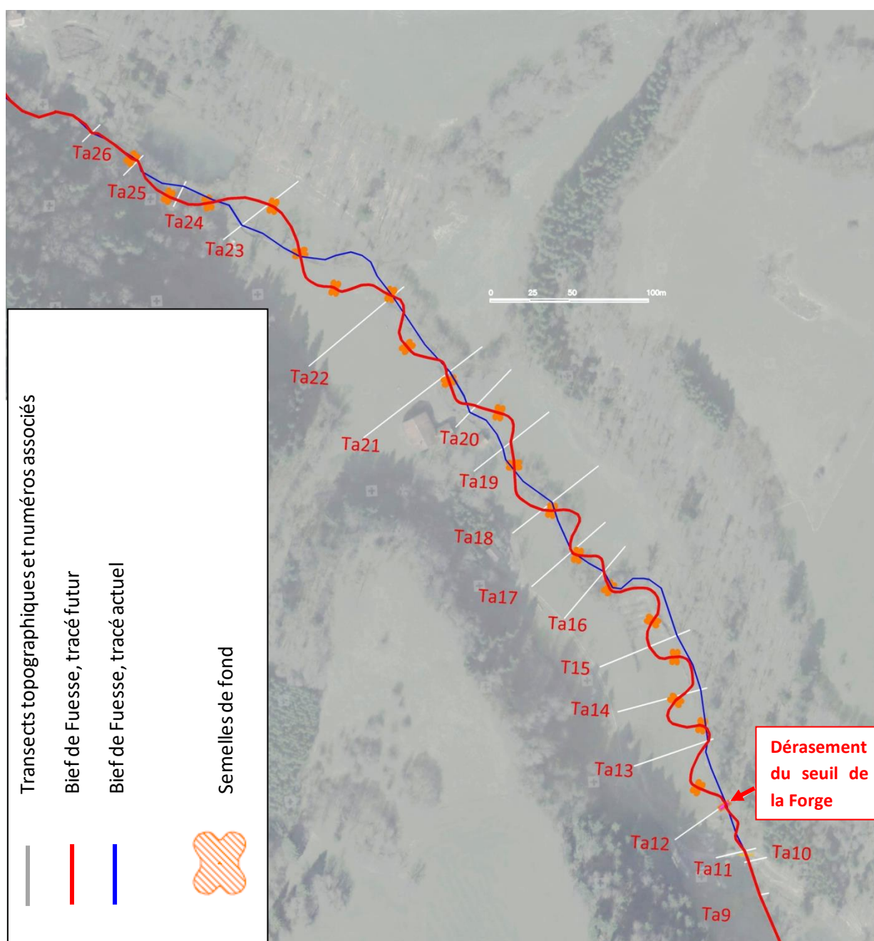
Figure 34 : Tracé actuel et projeté du bief de Fuesse sur le secteur amont.
