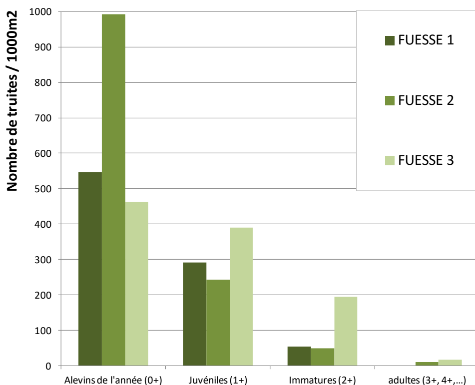
Figure 22: Répartition des différents écostades de chaque station et confrontation interstationnelle (inventaires 2013).
