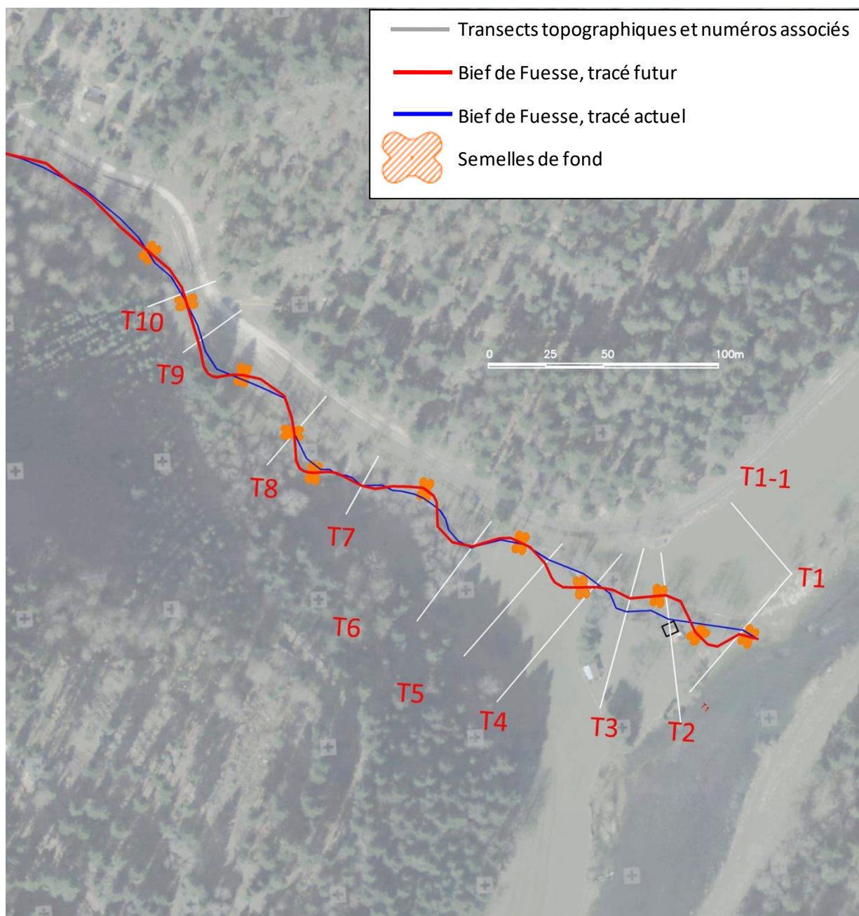
Figure 41 : Tracé actuel et projeté du bief de Fuesse sur le secteur aval.
