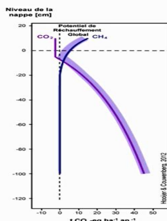
Figure 39. Relation entre le niveau de la nappe et les émissions de \text{CO}_2 en \text{t CO}_2 \text{ eq.ha}^{-1}.\text{an}^{-1} , d'après Hooijer et Couwenberg (2012).
