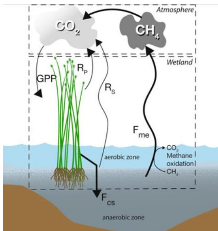
Figure 36. Dans Mitsch et al. (2013): Modèle conceptuel du cycle du carbone dans les zones humides, en tenant compte des échanges avec l'atmosphère. F cs : flux de séquestration du carbone ; F me : flux d'émissions du méthane ; GPP : productivité primaire ; R p : respiration par les plantes ; R s : respiration par le sol.
