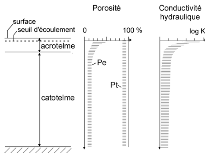
Figure 22. Modifiée d'après Wastiaux (2008) : Profil schématisé d'une tourbière haute et de quelques paramètres hydro-physiques. K : conductivité hydraulique à saturation. Pt : porosité totale. Pe : porosité efficace.
