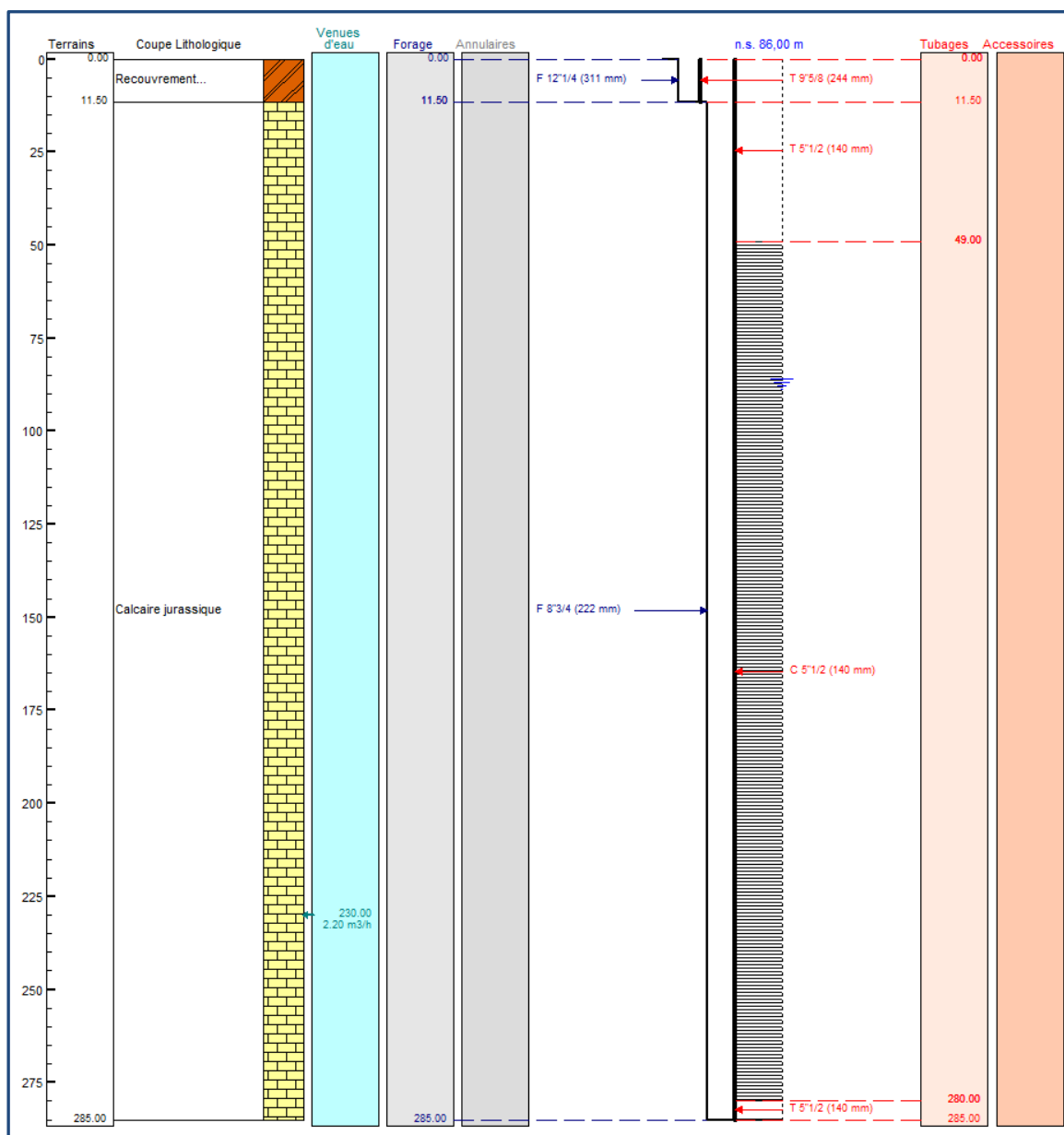
Illustration 6 : Coupe technique du forage BLAU (forage équipé PVC)
