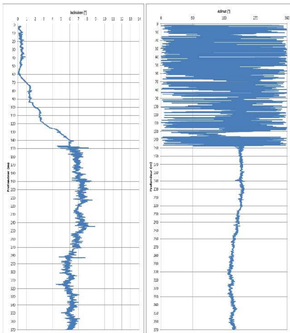
Figure 8 : Mesure de l'inclinaison et de l'azimut du forage d'Espezel
