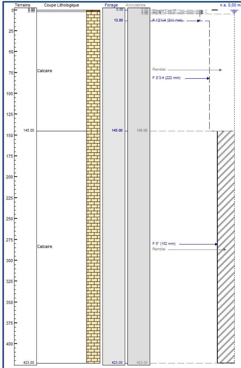
Illustration 6 : Coupe technique du forage ESPEZEL (forage rebouché)
