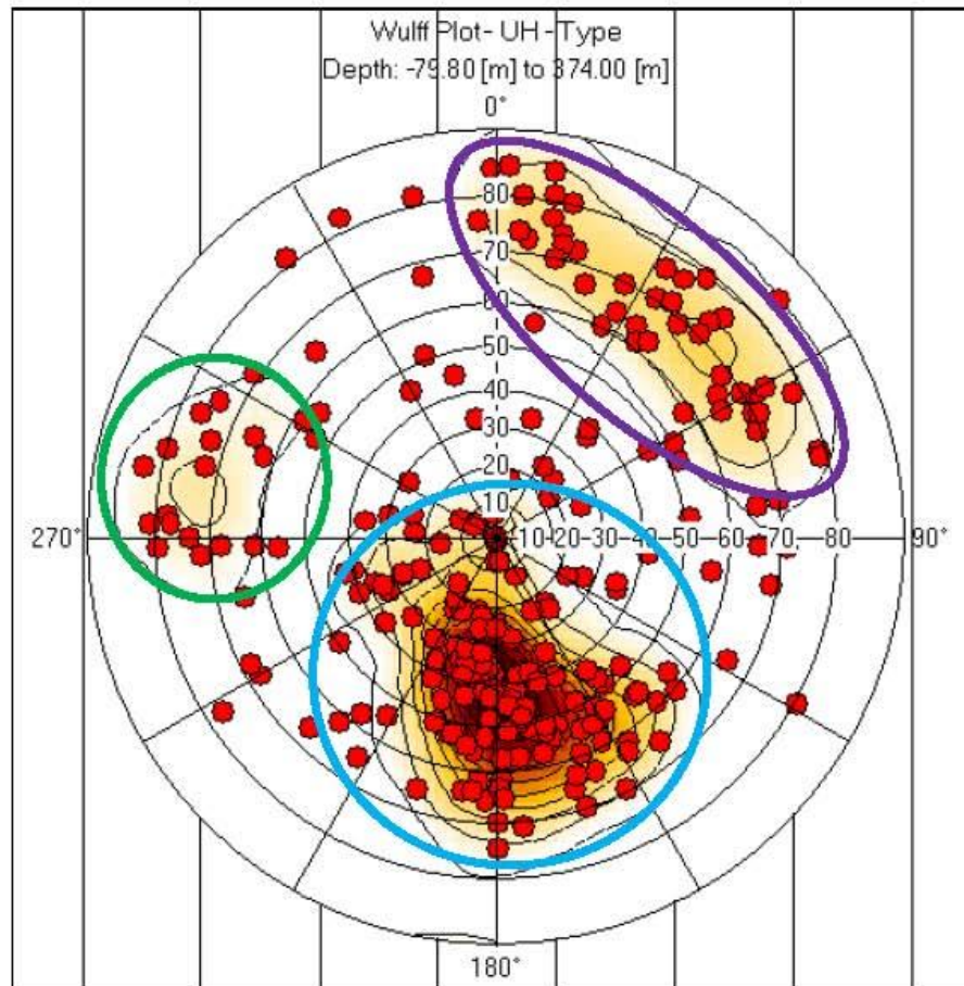
Figure 11 : Représentation des structures sur canevas de Wulff
