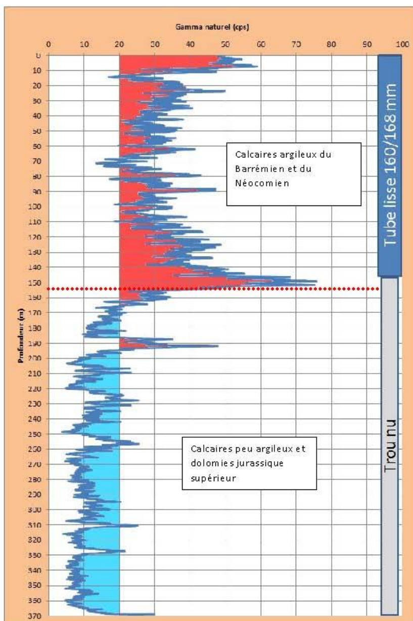
Figure 7 : Résultats de la diagraphie gamma naturel
