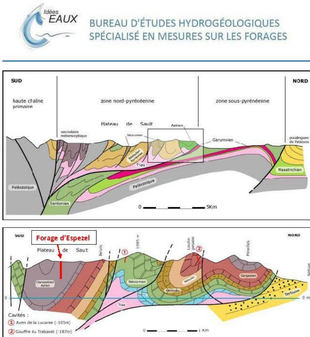
Figure 4: Coupe géologique Nord-Sud du Pays de Sault (d'après Souquet et al., 1980).
