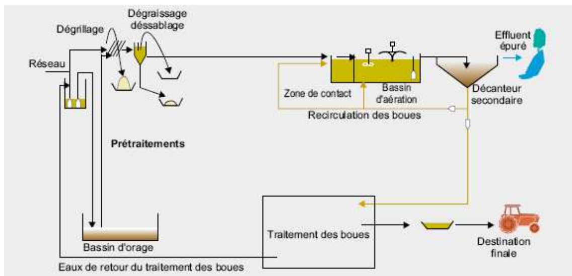
Figure 43 : Principe de traitement par boues activées en aération prolongée
