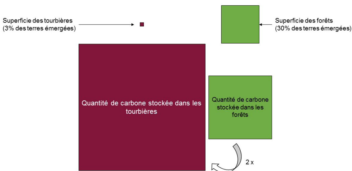
Figure 6 - Illustration de la disproportion de carbone stocké dans les tourbières par rapport à leur surface en comparaison avec les forêts (© G. Bernard)
