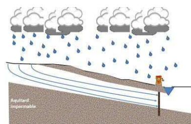
Modèle piston : zone de recharge localisée, écoulement isolé de la surface
