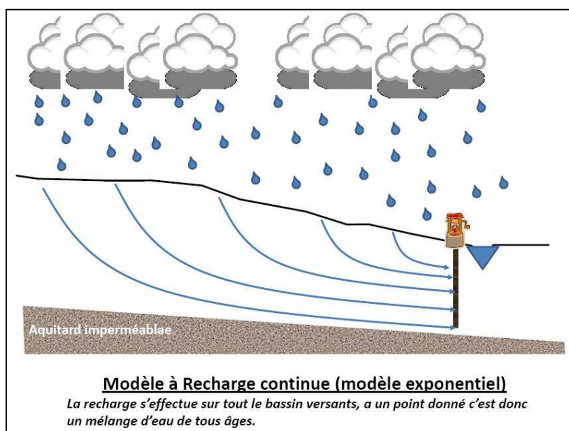
Figure 6 : Illustration du modèle Exponentiel (CONDATE EAU)
