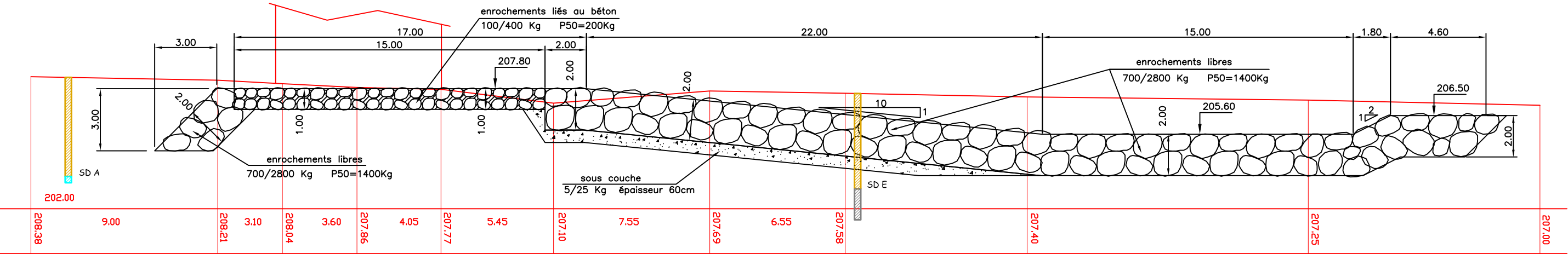
Coupe B-B
