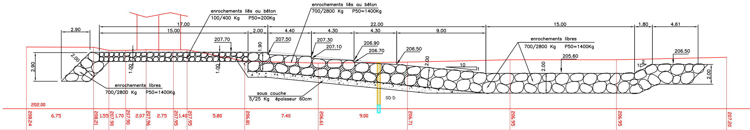
Coupe A-A zone d' coulement pr f rentiel
