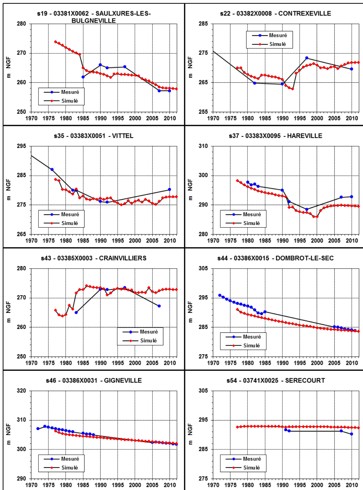
Figure 4 : Niveaux mesurés et niveaux simulés de 1977 à 2010 – Secteur sud-ouest du SAGE (Vittel-Contrexéville).
