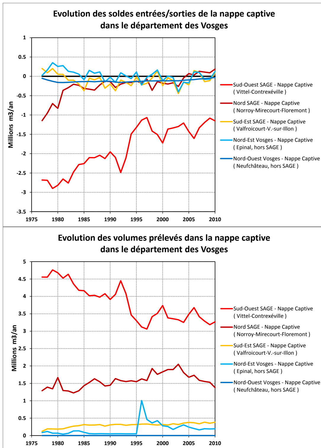
Figure 7 : Evolution des soldes entrées/sorties de la nappe captive des GTI et des volumes prélevés par secteurs géographiques du département des Vosges (1977-2010).
