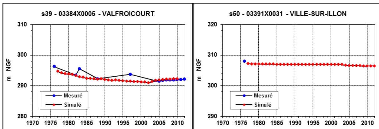
Figure 6 : Niveaux mesurés et simulés de 1977 à 2010 – Secteur sud-est du SAGE (Valfroicourt-Ville-sur-Illon).
