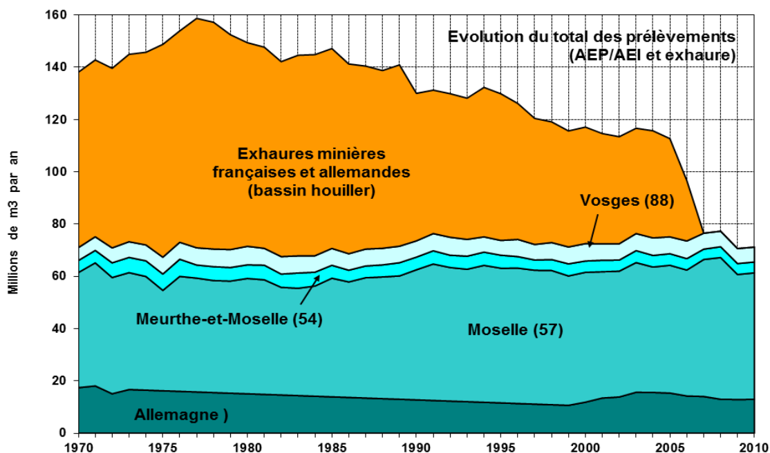
Figure 2 : Evolution de 1968 à 2010 du total des prélèvements effectués dans la nappe captive des grès du Trias inférieur et dans la nappe libre du bassin houiller.
