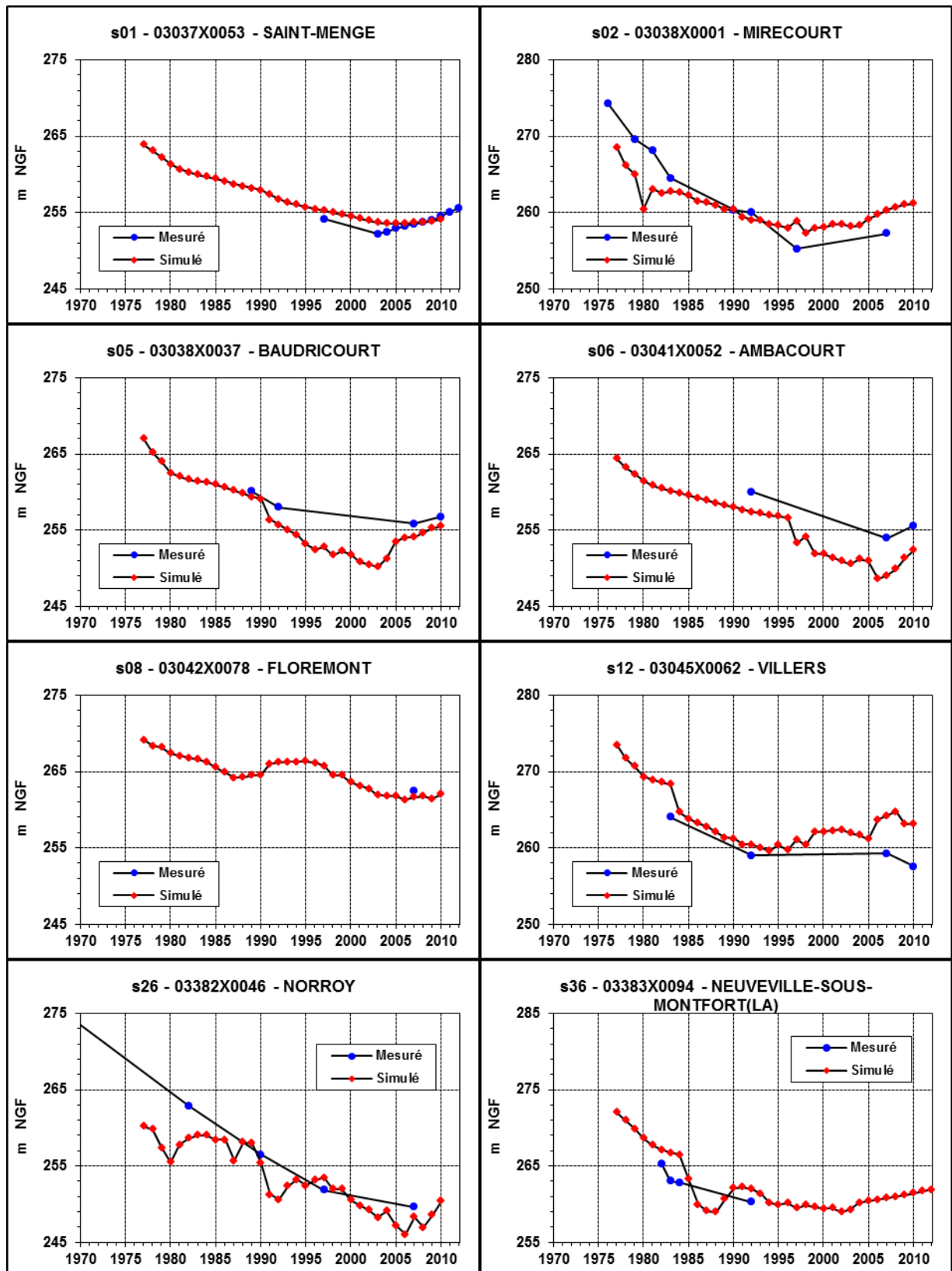
Figure 5 : Niveaux mesurés et simulés de 1977 à 2010 – Secteur nord du SAGE (Norroy-Mirecourt-Floremont).
