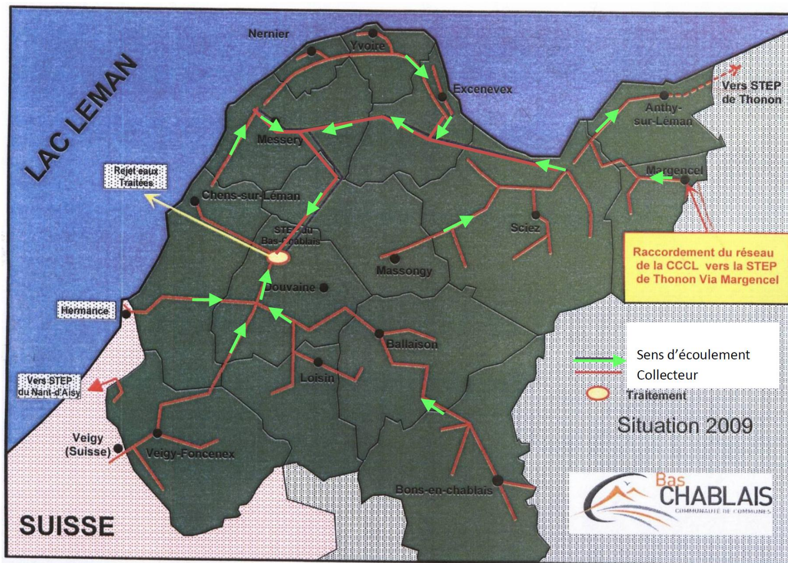
Figure 44 : Schéma général d'assainissement de la région du Bas Chablais (Source : CCBC- 2009)
