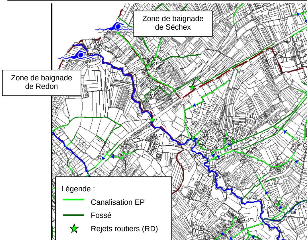
Figure 58 : Réseau des eaux pluviales et rejets routiers dans la partie aval du Redon (source : Burgeap 2010)
