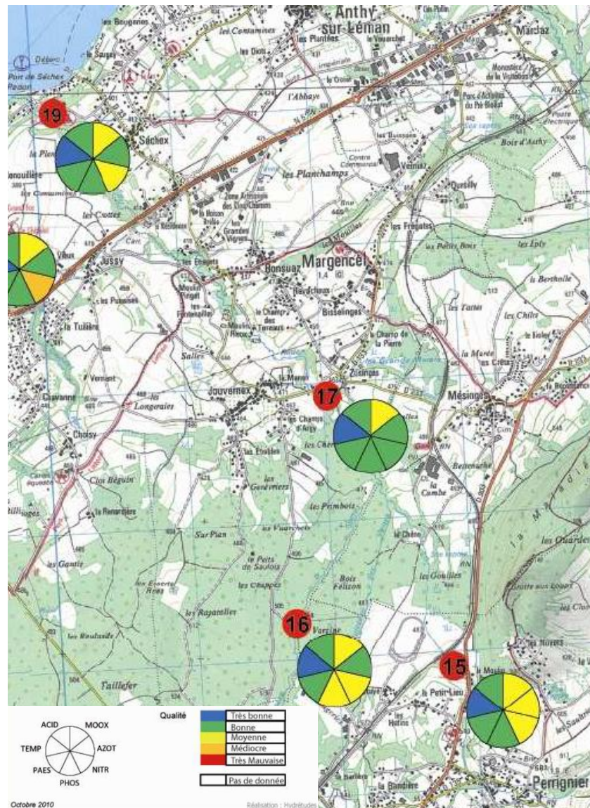
Figure 53 : Localisation des stations et détails de la qualité des paramètres physico-chimiques du bassin versant du Redon à l'aval de Perrignier (Source : Hydrétudes, 2009-2010)
