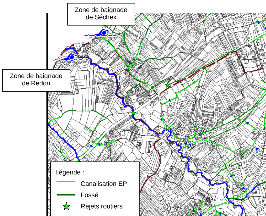
Figure 43 : Réseaux des eaux pluviales ayant pour exutoire le Redon sur sa partie aval
