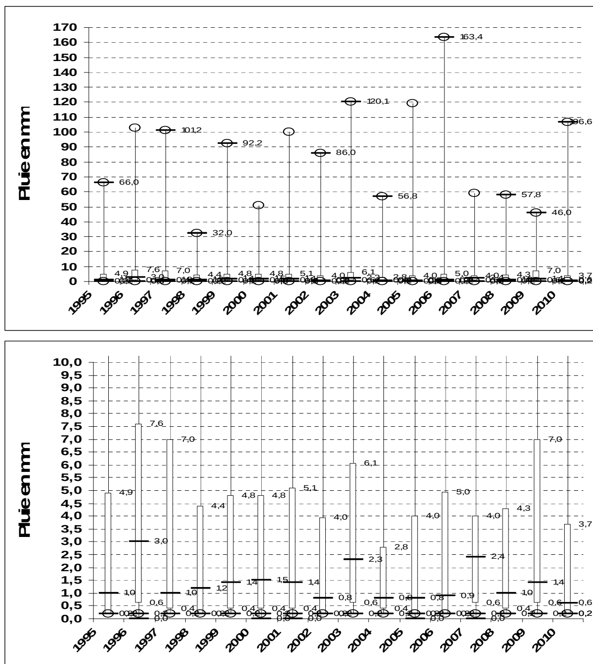
Figure 4 : Boîtes à moustaches des distributions des intensités de pluies des années 1995 à 2010 avec 2 échelles de représentation, en haut pour voir les pluies maximales et en bas pour voir les pluies médianes et les quartiles
