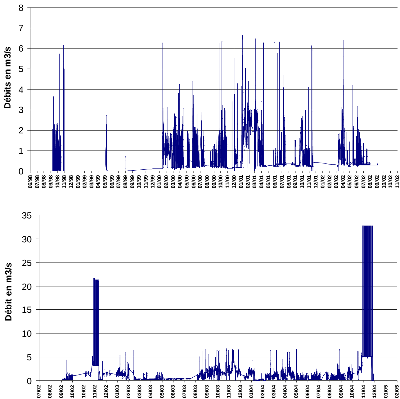
Figure 8 : Données de débits au déversoir du Canélou (Mandirac) de 1998 à 2002 (en haut) et de 2002 à 2005 (en bas)
