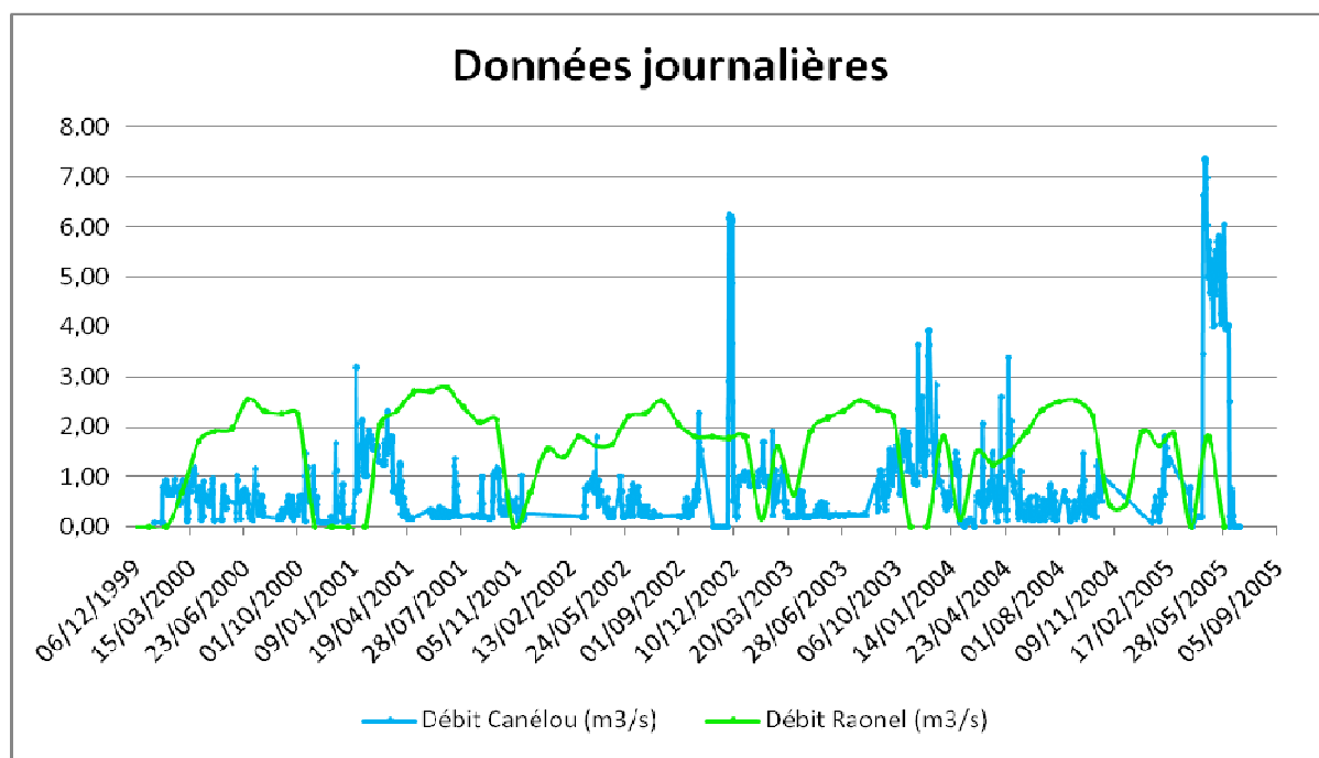
Figure 7 : Evolution des débits mesurés au niveau de la prise d'eau sur l'Aude à Raonel et du déversoir du Canérou sur la période de 2000 à 2005 (Le Noc et De Witt, 2010)
