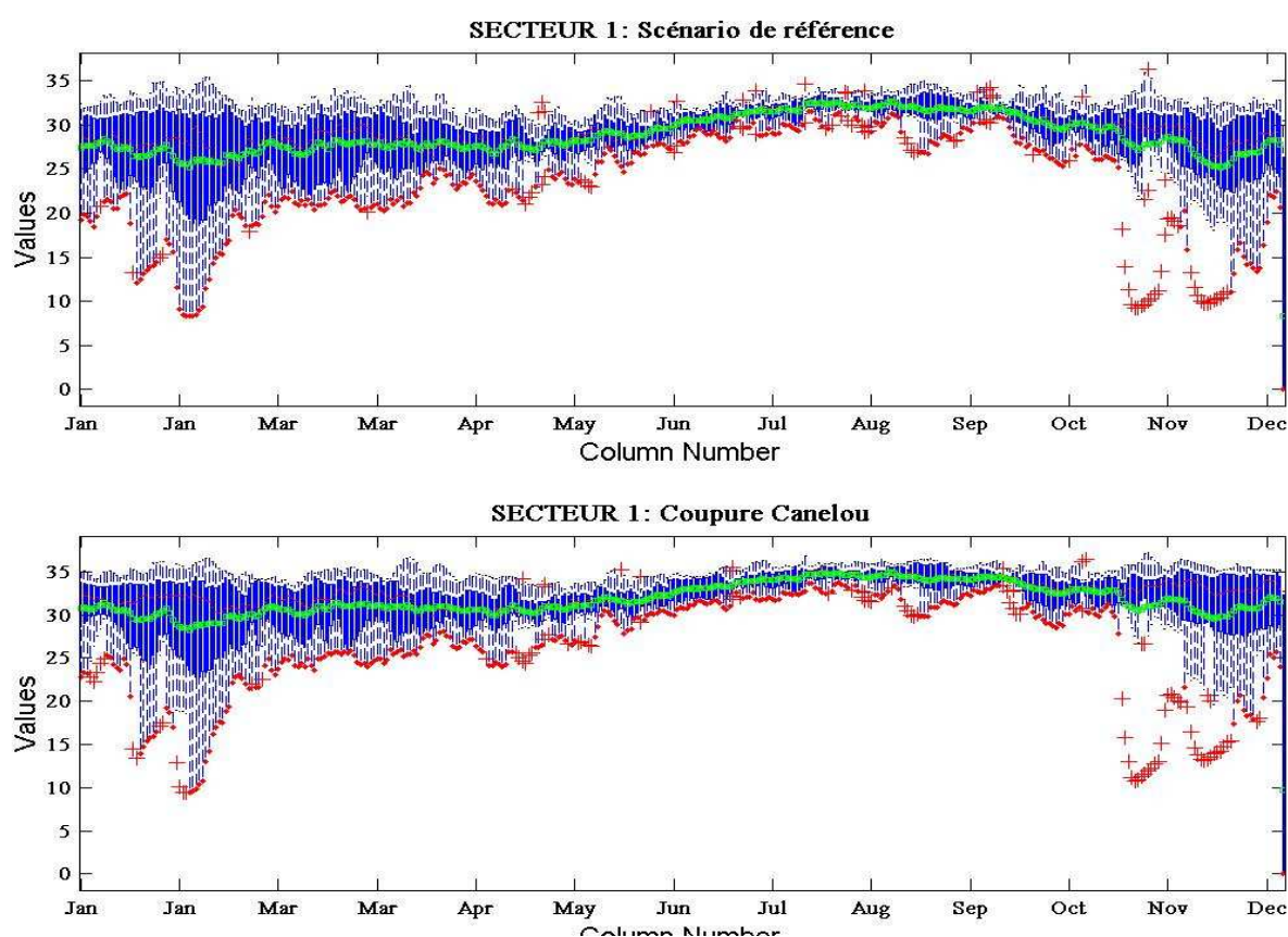
Figure 54 : Boxplot journalieres (2000-2004) pour le secteur 1 de la situation de référence et du scénario de coupure du Canelou.
