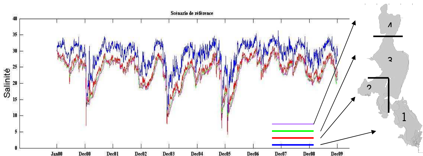
Figure 42 : Evolution de la salinité moyenne pour les 4 secteurs et sous-bassins choisis entre 2000 et 2010 pour le scénario de référence
