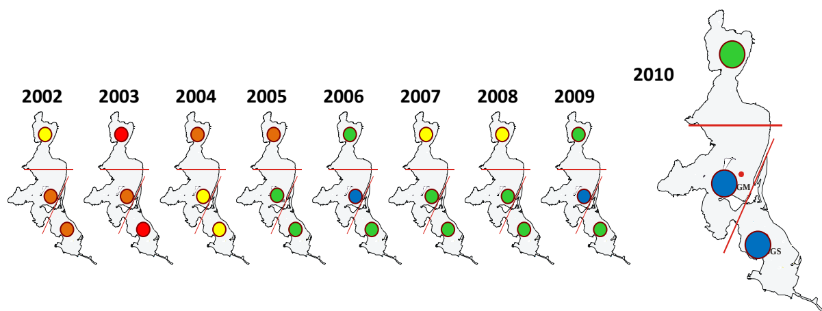
Figure 2 : Etat vis-à-vis de l'eutrophisation de la colonne d'eau (résultats du RSL 2002-2010)
