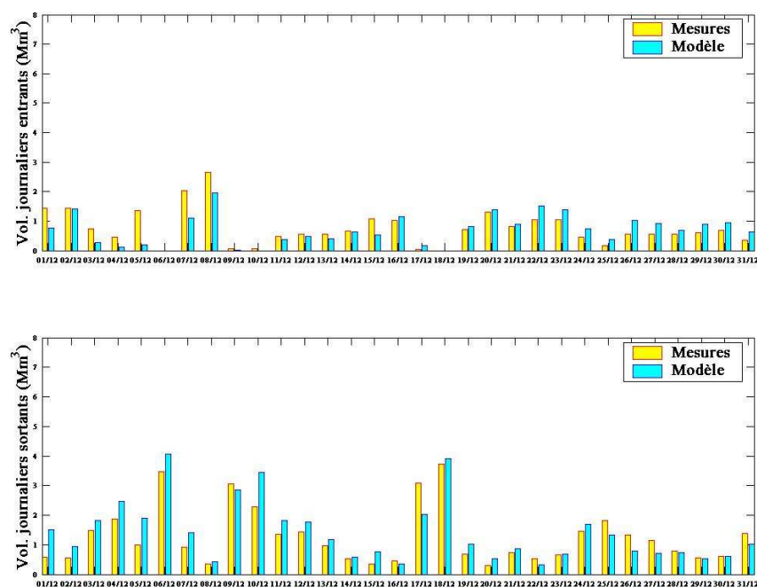
Figure 80 : Volumes journaliers entrants et sortants de la lagune simulés (bleu) et observés (jaune) au cours du mois de décembre 2006
