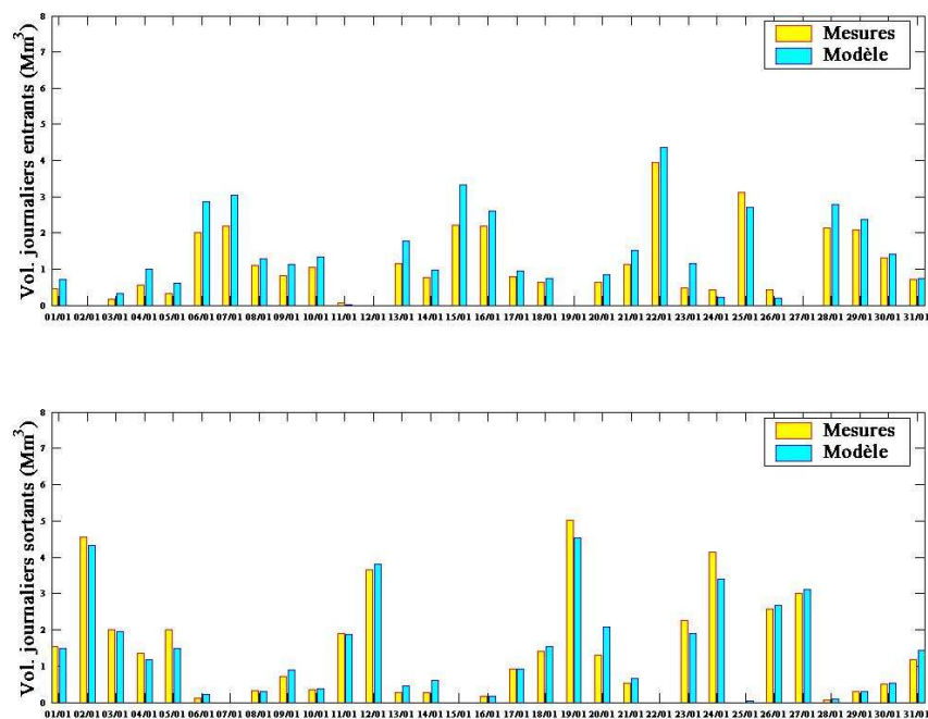
Figure 81 : Volumes journaliers entrants et sortants de la lagune simulés (bleu) et observés (jaune) au cours du mois de janvier 2007
