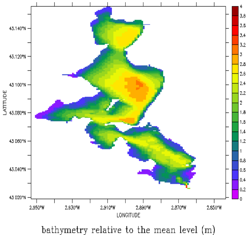
Figure 14 : Grille de calcul bathymétrique du modèle MARS 3D (65m de résolution) sur la lagune de Bages-Sigean
