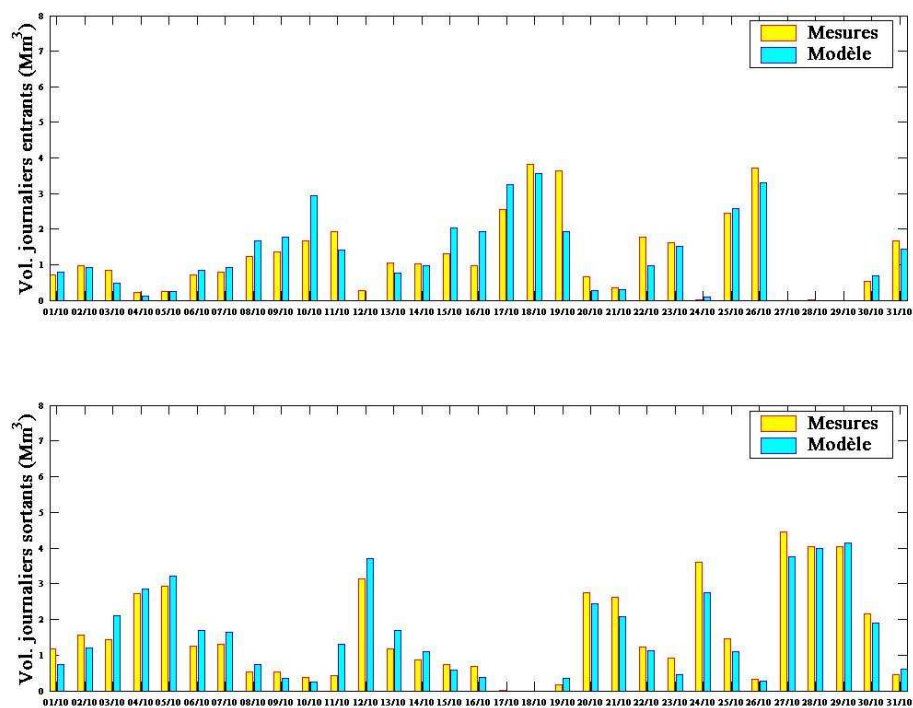
Figure 78 : Volumes journaliers entrants et sortants de la lagune simulés (bleu) et observés (jaune) au cours du mois d'octobre 2006
