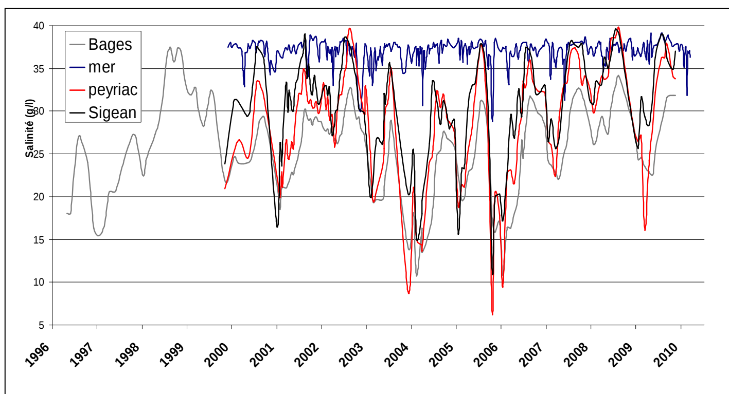
Figure 13 : Salinité mesurée en différentes stations entre 1995 et 2010, en mer (bleu, à Sigean (noir), à Peyriac (rouge) et à Bages (en gris) (données RSL-FILMED)
