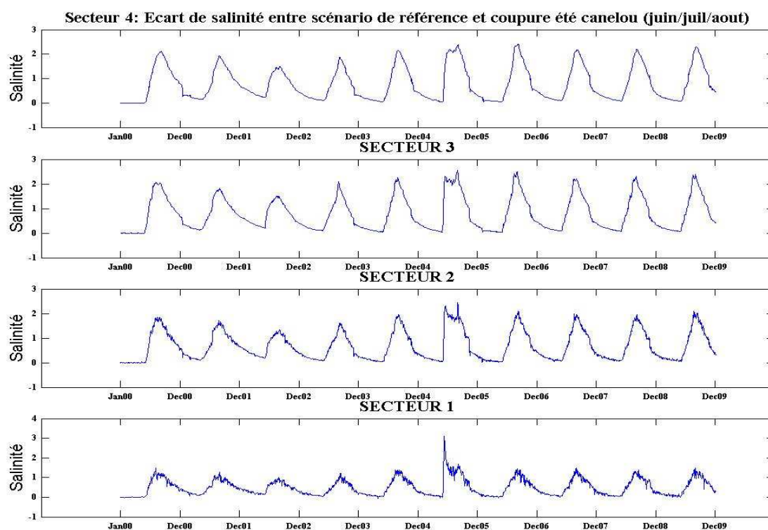
Figure 57 : Différence de la Salinité moyenne pour les 4 secteurs définis entre 2000 et 2010 entre le scénario de référence et le scénario de coupure estivale (juin/juillet/août) du Canélon
