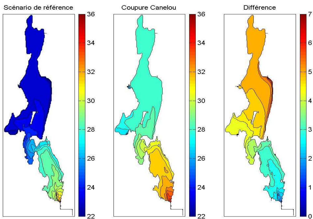
Figure 50 : Salinité moyenne (2000-2004) du scénario de référence (à gauche), le scénario « coupure du Canélon » (au centre) et la différence des deux scénarii (à droite)
