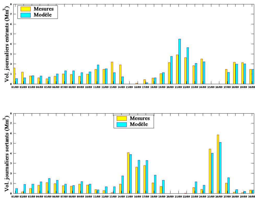
Figure 77 : Volumes journaliers entrants et sortants de la lagune simulés (bleu) et observés (jaune) au cours du mois de septembre 2006
