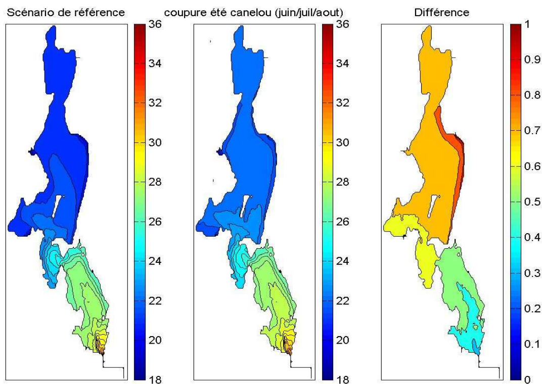
Figure 56 : Salinité moyenne (2000-2011) du scénario de référence (à gauche), le scénario « coupure des apports estivaux du Canélon » (au centre) et la différence des deux scénarii (à droite)
