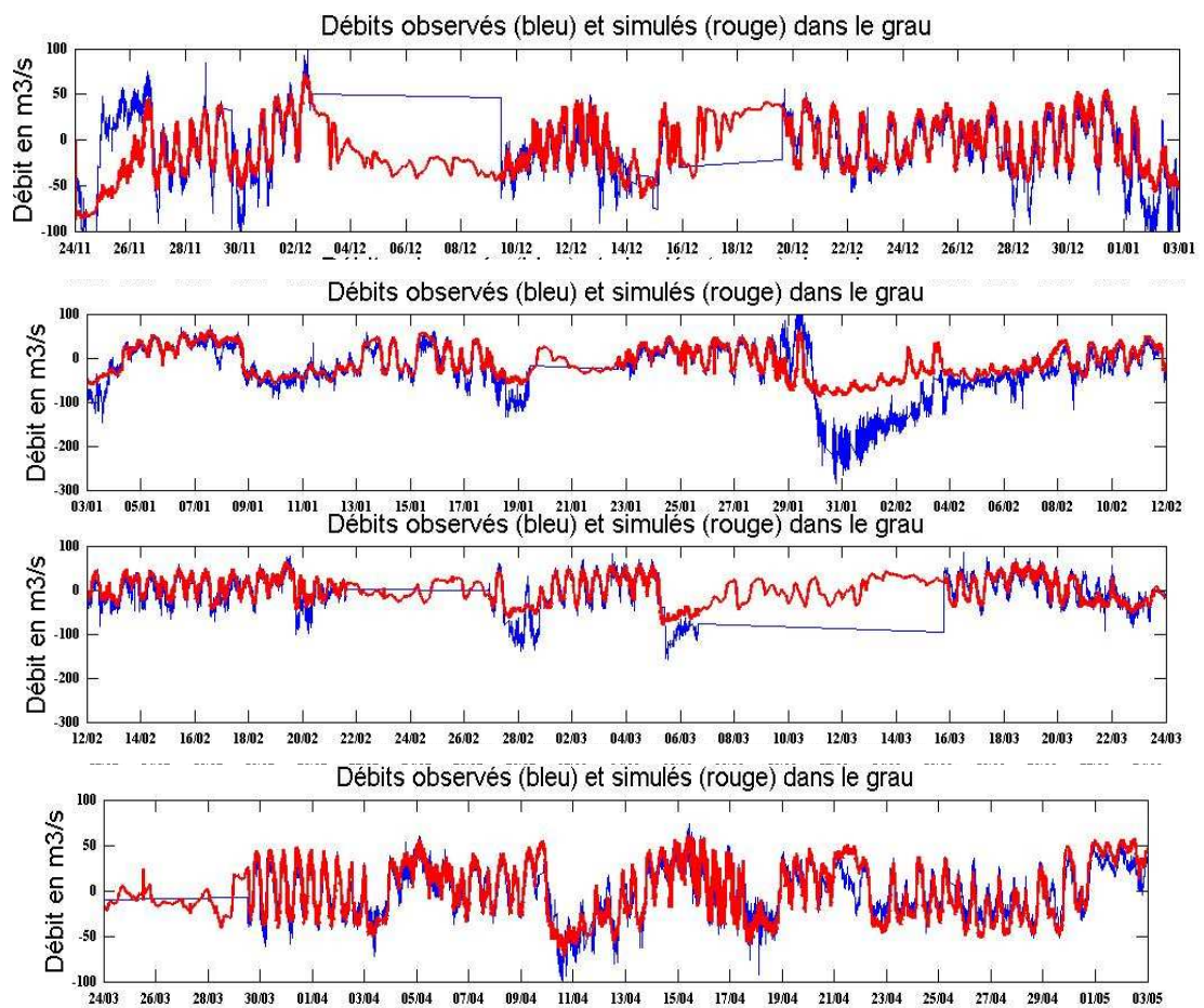
Figure 15 : Débit observés (en bleu) et simulés (en rouge) du 24 novembre 2005 au 03 mai 2006
