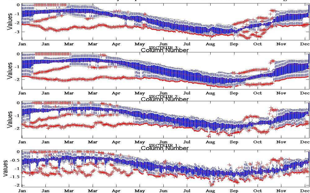
Figure 66 : Boxplots journalieres (2000-2010) pour les 4 secteurs 4 des différences de salinité moyenne sur l'année entre la situation de référence et du scénario d'apports agricoles (50%)
