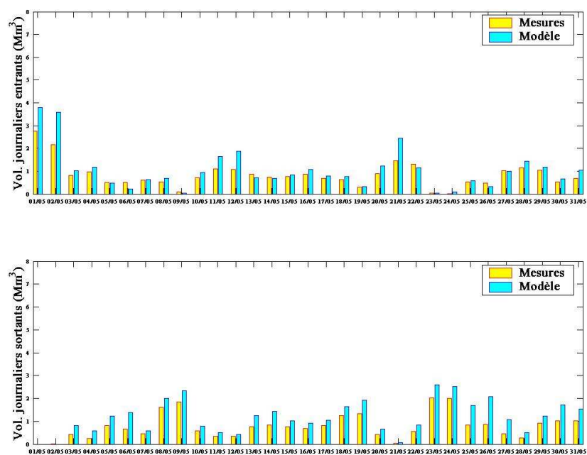
Figure 73 : Volumes journaliers entrants et sortants de la lagune simulés (bleu) et observés (jaune) au cours du mois de mai 2006
