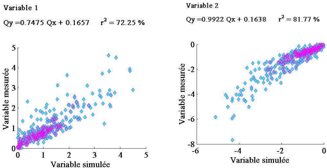
Figure 21 : Comparaison et régression statistiques des volumes journaliers entrants (à gauche) et sortants (à droite) simulés et observés sur la période de mars 2006 à Avril 2007 (on enlève la période du gros évènement pluvieux de février 2006)
