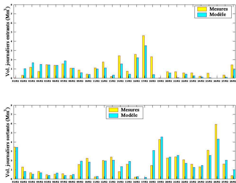
Figure 82 : Volumes journaliers entrants et sortants de la lagune simulés (bleu) et observés (jaune) au cours du mois de février 2007
