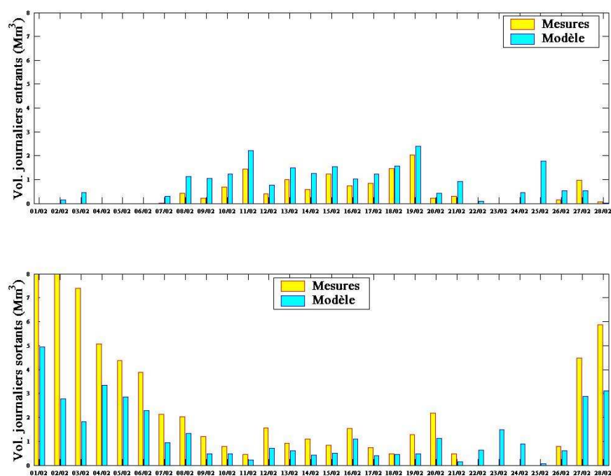
Figure 72 : Volumes journaliers entrants et sortants de la lagune simulés (bleu) et observés (jaune) au cours du mois de février 2006
