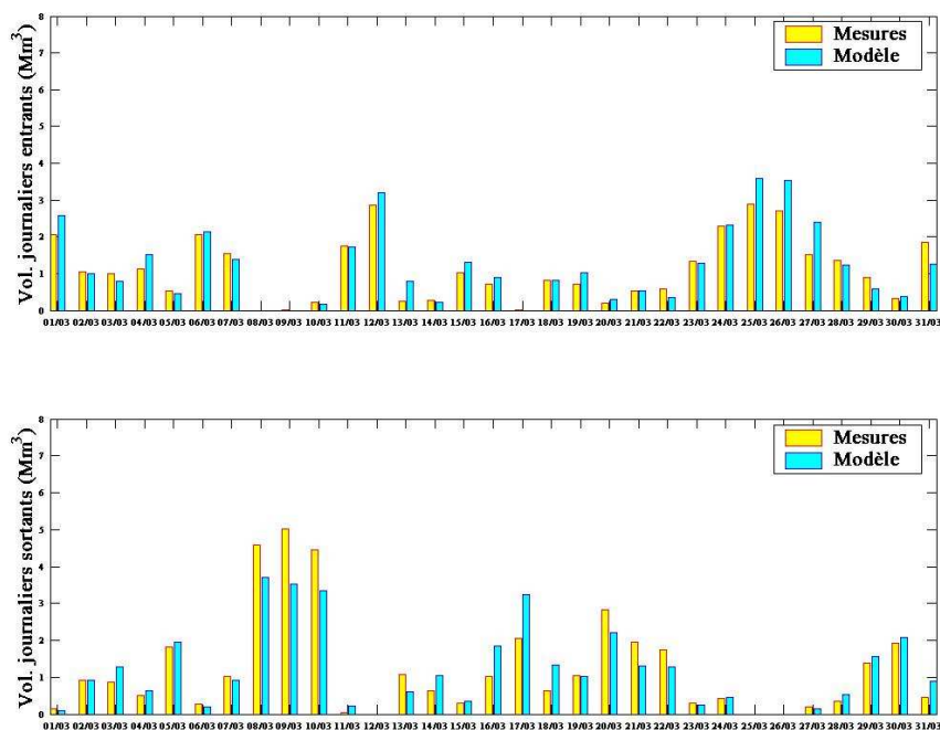
Figure 83 : Volumes journaliers entrants et sortants de la lagune simulés (bleu) et observés (jaune) au cours du mois de mars 2007
