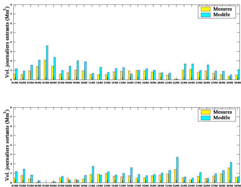
Figure 74 : Volumes journaliers entrants et sortants de la lagune simulés (bleu) et observés (jaune) au cours du mois de juin 2006
