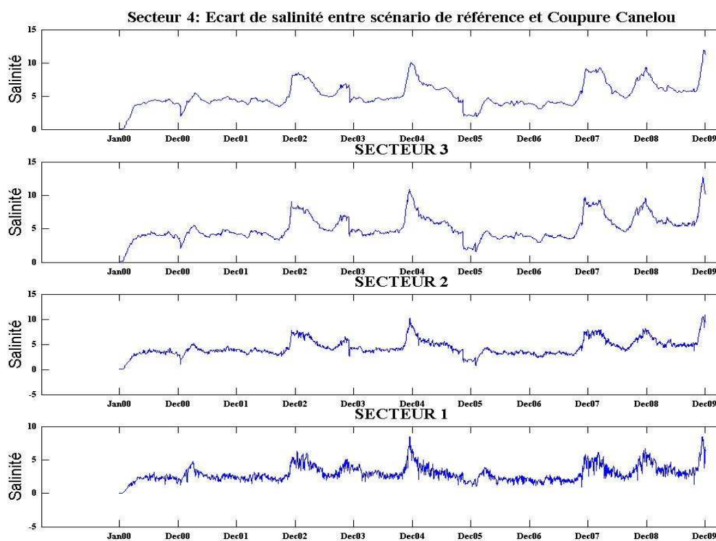
Figure 51 : Différence de la Salinité moyenne pour les 4 secteurs définis entre 2000 et 2010 entre le scénario de référence et le scénario de coupure totale du Canélon
