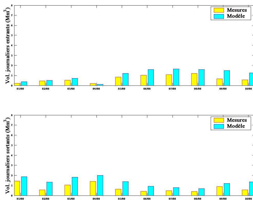
Figure 76 : Volumes journaliers entrants et sortants de la lagune simulés (bleu) et observés (jaune) au cours du mois de août 2006
