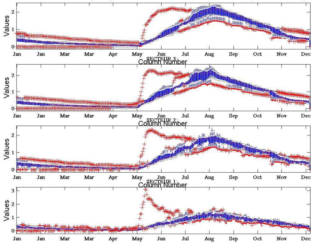
Figure 58 : Boxplot journalières (2000-2010) pour les 4 secteurs 4 des différences de salinité moyenne sur l'année entre la situation de référence et du scénario de coupure estivale du Canérou.
