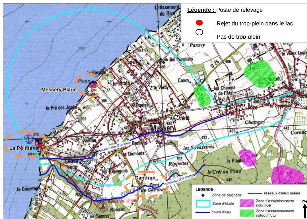
Figure 47 : Localisation des postes de relevage dans la zone d'étude
