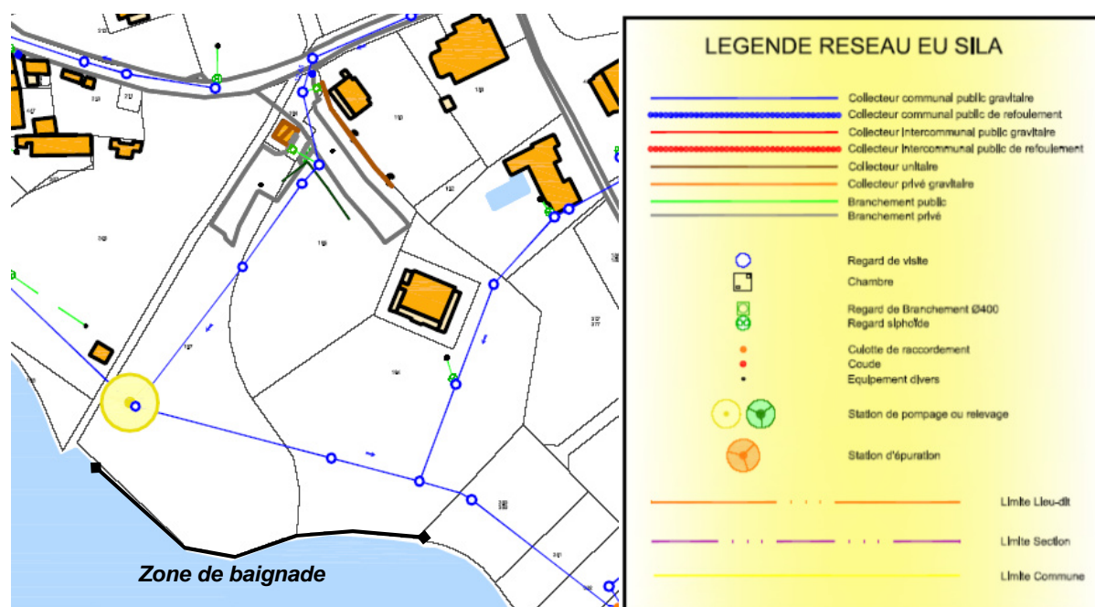
Figure 42 : Réseau d'assainissement collectif dans l'enceinte de la plage (source : SILA)
