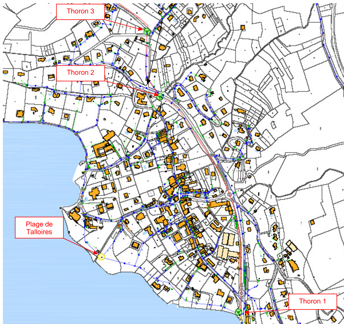
Figure 41 : Localisation des postes de relevage dans la zone d'étude (source : SILA)
