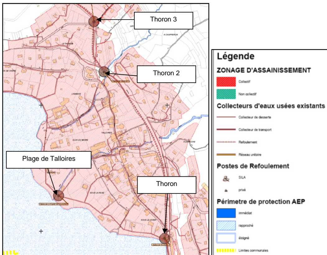
Figure 34 : Localisation des stations de pompage de la zone d'étude (source : SILA)
