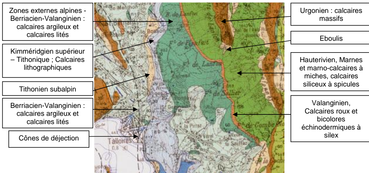
Figure 30 : Extrait de la carte géologique au niveau de la zone d'étude (Source: BRGM)
