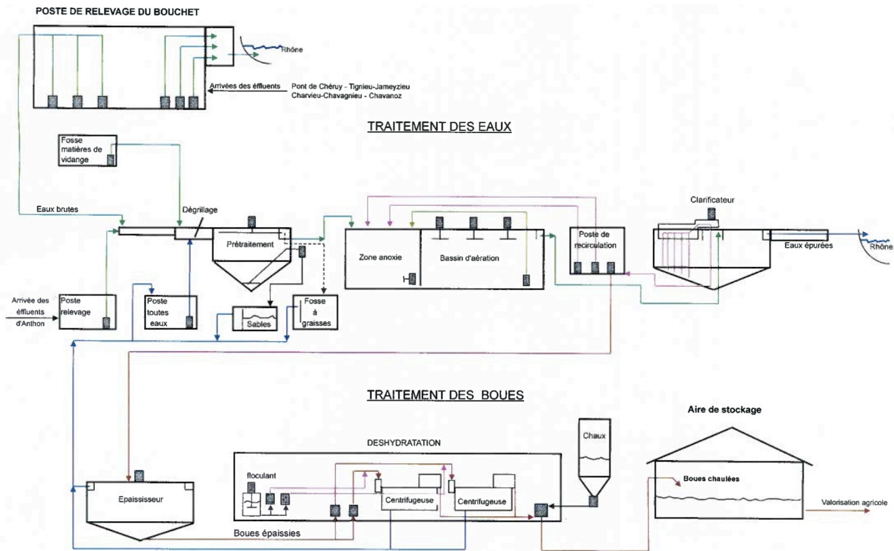
Figure 1 : Schéma des installations de la station d'épuration de Chavanoz
