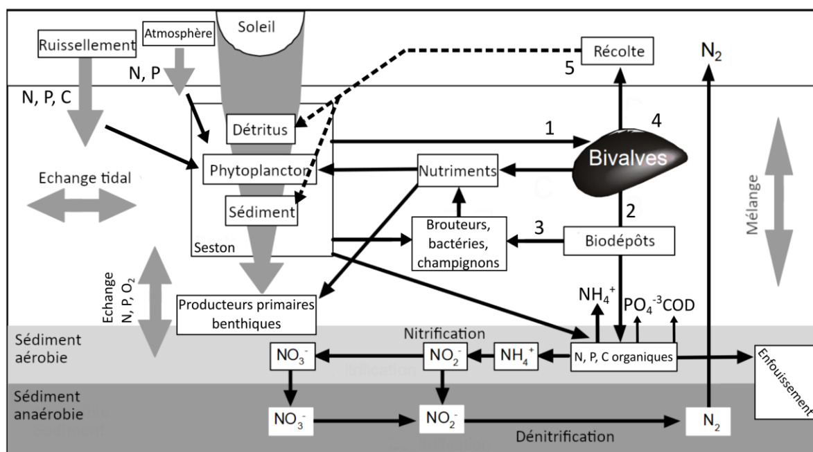
Figure 4 : diagramme conceptuel des interactions entre l'élevage de bivalves et les écosystèmes côtiers. 1 : retrait de la matière particulaire en suspension (sésion 37 ) au cours de l'alimentation par filtration ; 2 : biodépôt de la matière organique non digérée sous forme de fèces ou de pseudofèces ; 3 : excrétion de nutriments (principalement sous forme d'ammoniac ionisé en ammonium et aussi sous forme de phosphate et autres nutriments organiques) ; 4 : retrait de matériel biologique (N, P et carbone organique) lors de la récolte des bivalves ; 5 : remise en suspension de nutriments, de débris et de sédiments dans la colonne d'eau lors des activités de récolte (traduit d'après Burkholder & Shumway (2011) modifié de Cranford et al. 2006).
