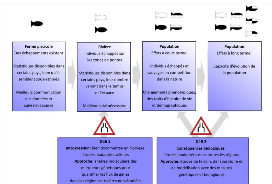
Figure 21 : les deux défis majeurs limitant la documentation sur les impacts génétiques des individus échappés de saumon atlantique sur les populations sauvages (traduit de Glover et al. (2017)).
