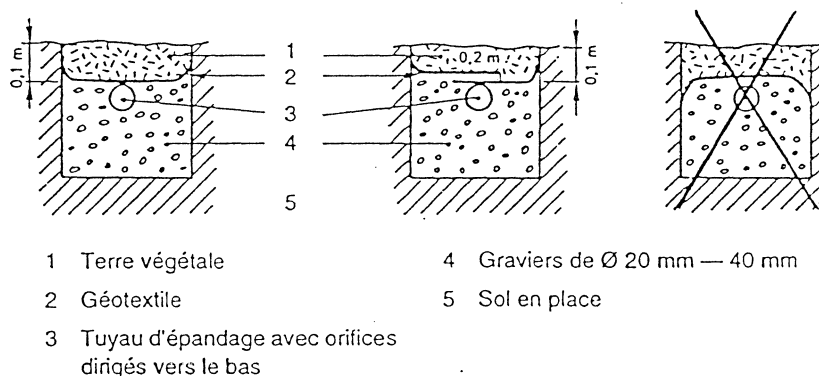
Figure 3 : Coupe : disposition du géotextile
