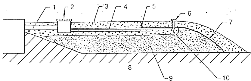
Figure 9 : Tètre d'infiltration hors sol
