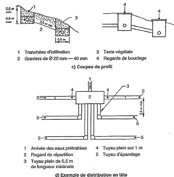
Figure 5 : Tranchées d'infiltration en terrain en pente (fin)
