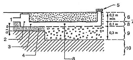
b) Coupe transversale d'une tranchée
