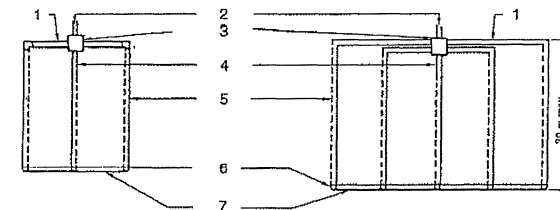
Figure 3 : Coupe : disposition du géotextile
