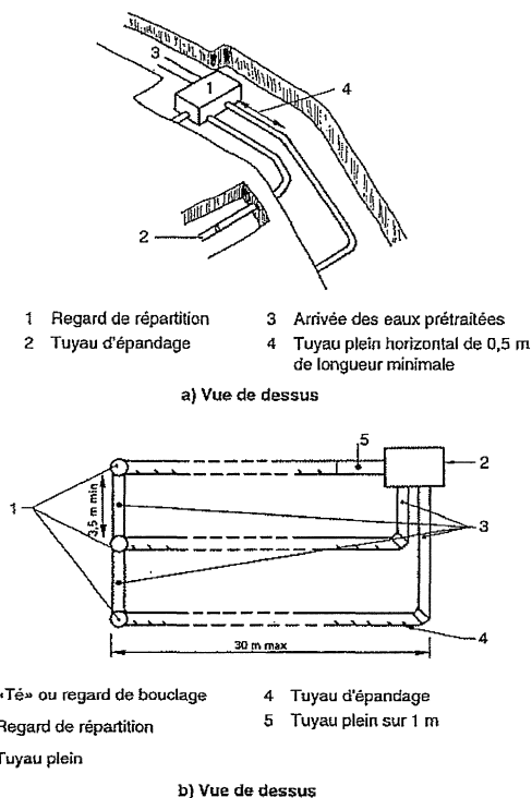
Figure 5 : Tranchées d'infiltration en terrain en pente
