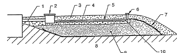
Figure 9 : Tertre d'infiltration hors sol
