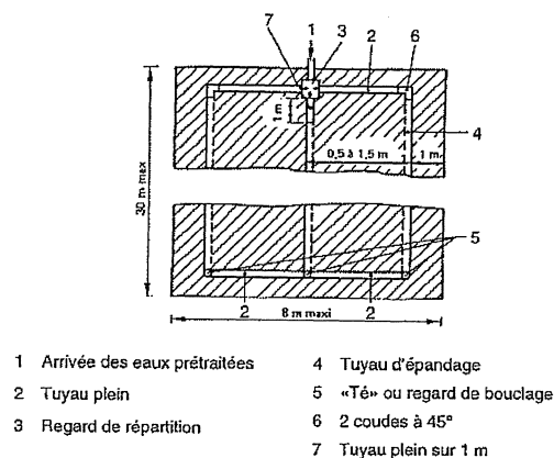
Figure 6 : Lit d'épandage
