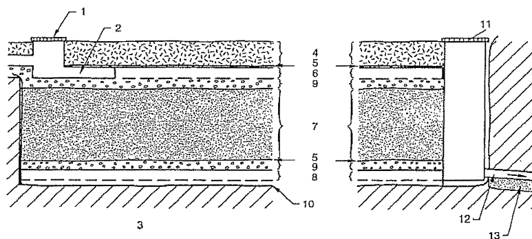
b) Coupes transversales (suite)
