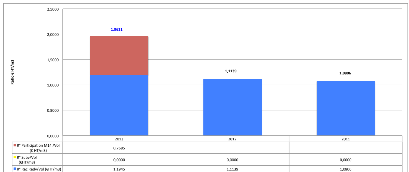
Graph 26 : Ratio économique de référence du service Eau Potable (en €HT/m 3 )
