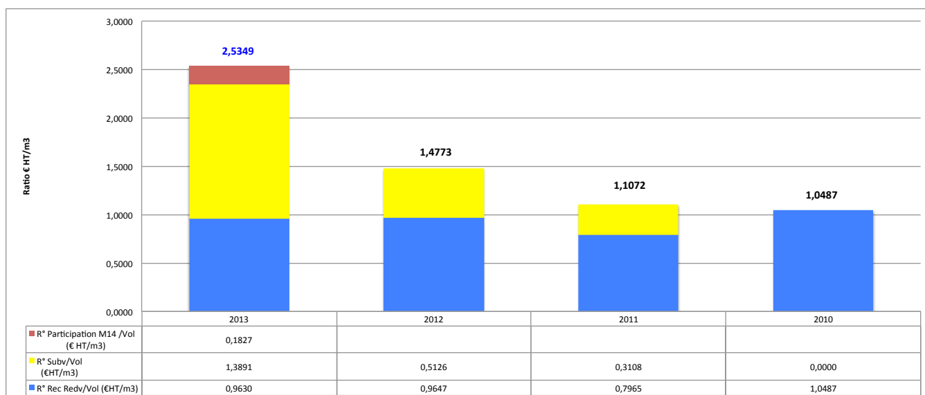
Graph 44 : Ratio économique de référence du service Assainissement (en €HT/m 3 )
