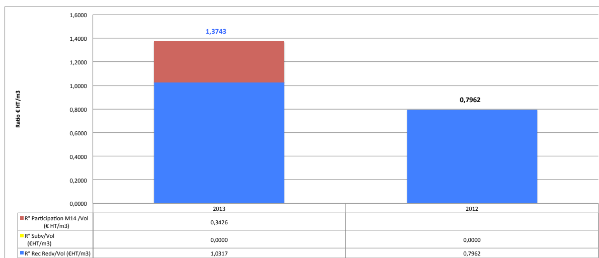
Graph 34 : Ratio économique de référence du service Assainissement Collectif (en €HT/m 3 )
