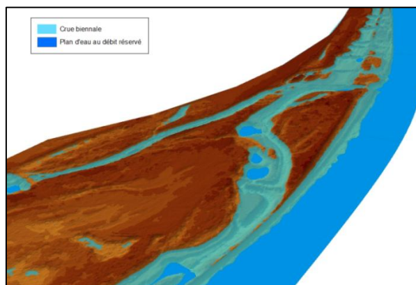
Figure 3 : Illustration en trois dimensions de la projection de la ligne d'eau de Q_2 issue du modèle 1D sur le MNT réalisé à partir du Lidar de 2009 au droit du site de Ciselande (n°13).
