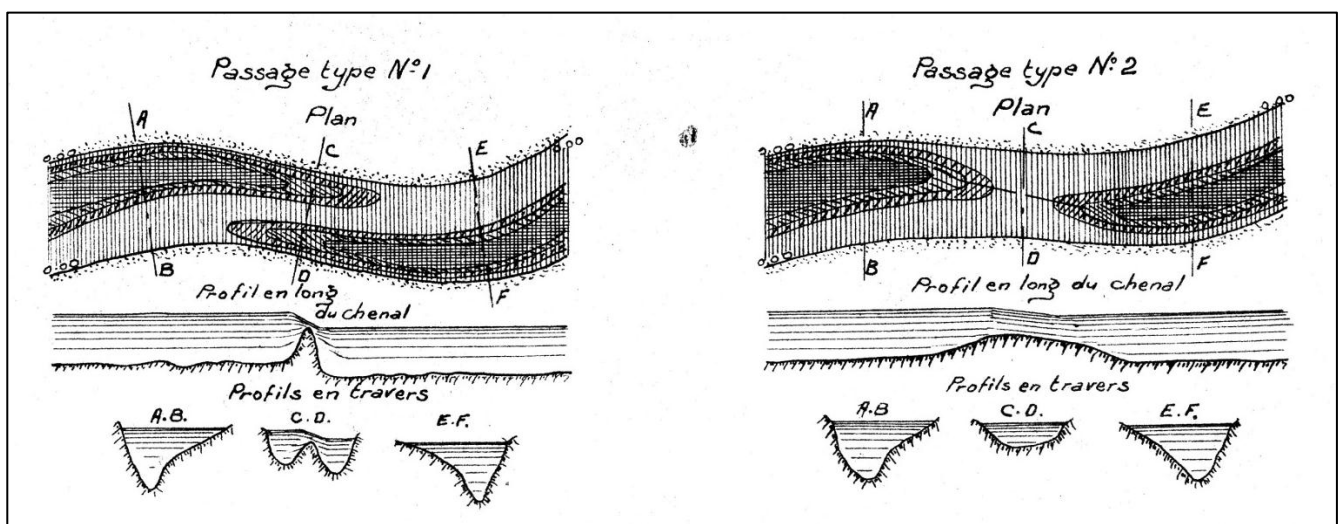
Figure 1 : Schéma type d'un mauvais passage (n°1) et d'un bon passage (n°2) (Girardon, 1894).
