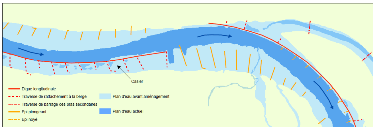
Figure 2 : Schéma de principe des aménagements Girardon.
