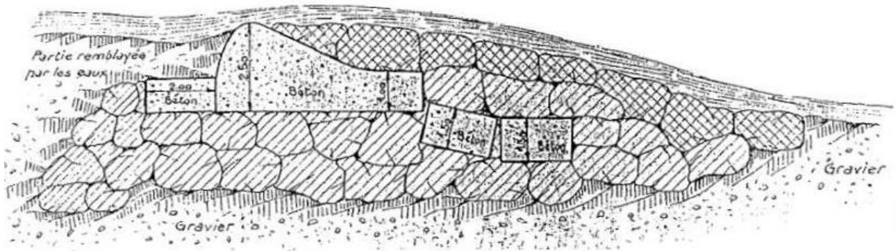
– Coupe transversale 1 ère réalisation (1901) –
