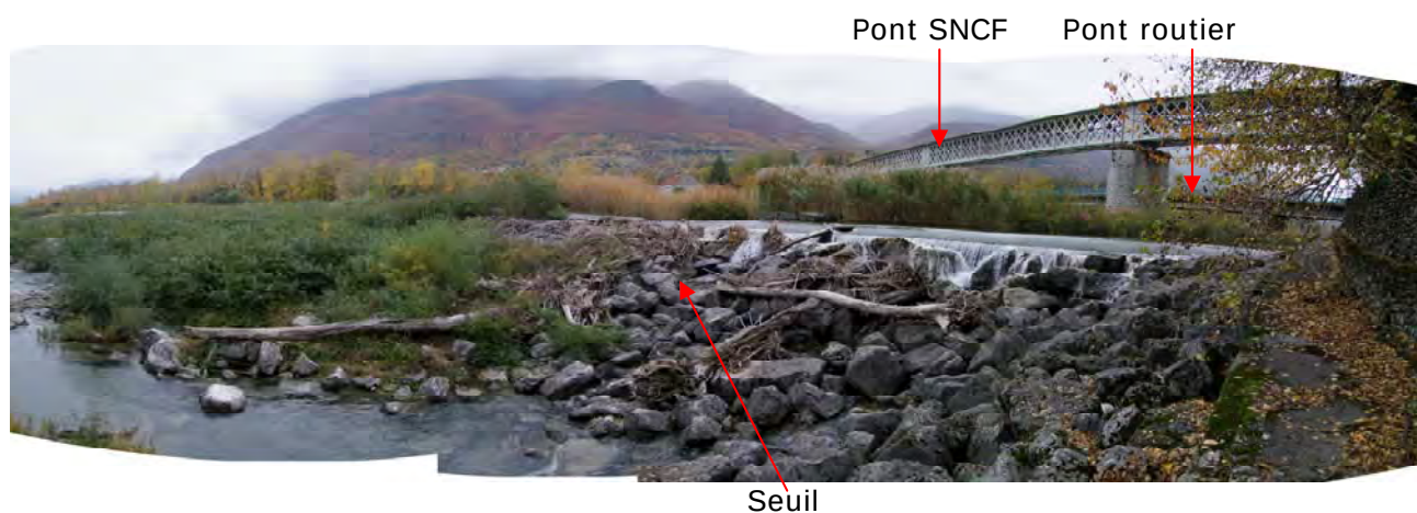
Vue générale du seuil depuis la rive gauche
