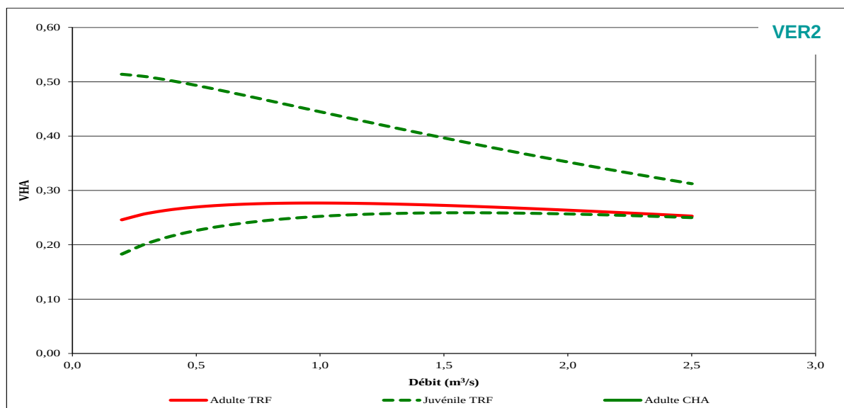
Évolution de la VHA en fonction du débit
