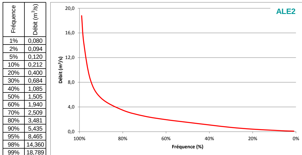
Graphique 4 : Courbe des débits classés de l'Allemogne à Thoiry
