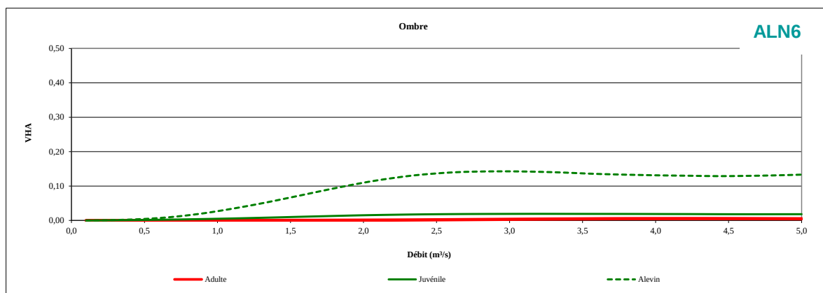
Évolution de la VHA en fonction du débit pour l'ombre
