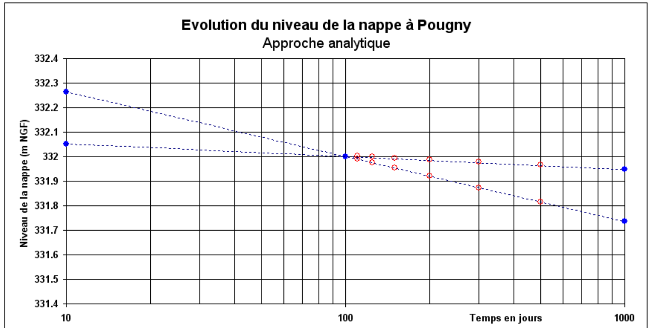
Graphique 27 : Approche analytique : évolution du niveau de la nappe à Pougny
