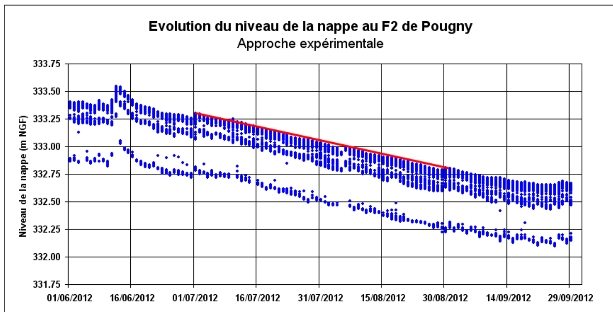
Graphique 26 : Approche expérimentale : évolution du niveau de la nappe au F2 à Pougny
