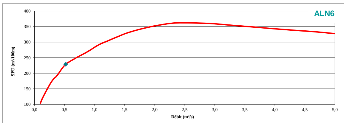
Évolution de la SPU en fonction du débit pour le chabot
