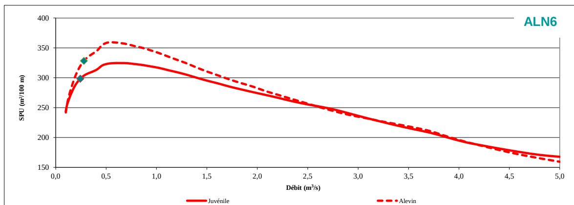
Évolution de la SPU en fonction du débit : truites juvéniles et alevins
