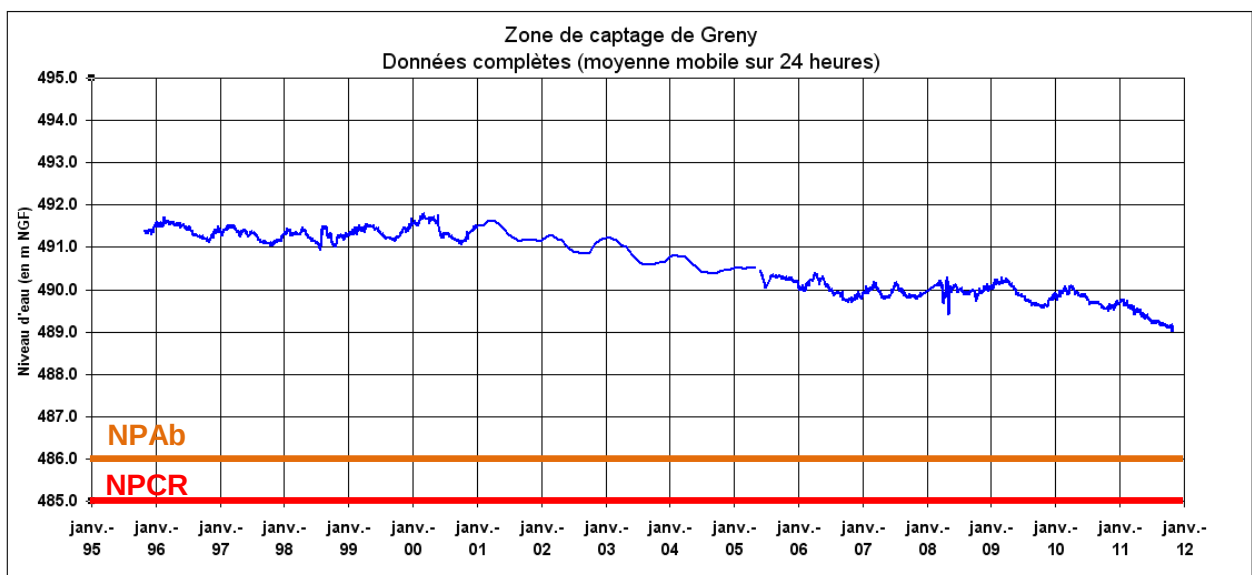
Graphique 22 : Représentation graphique des seuils d'alertes piézométriques pour Greny
