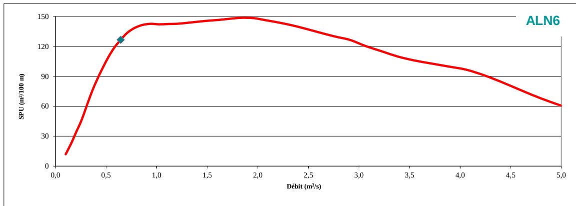
Évolution de la SPU en fonction du débit pour la reproduction de la truite
