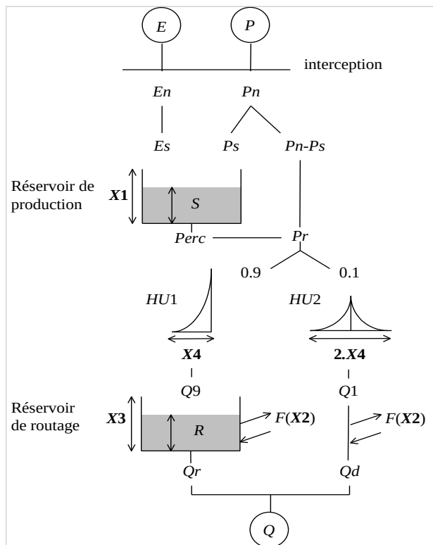
Figure 17 : Schéma de la structure du modèle GR4J
