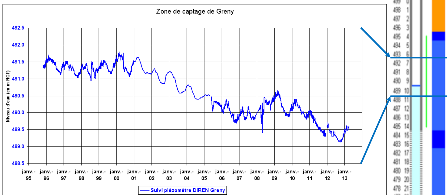
Graphique 10 : Suivi piézométrique de Greny
