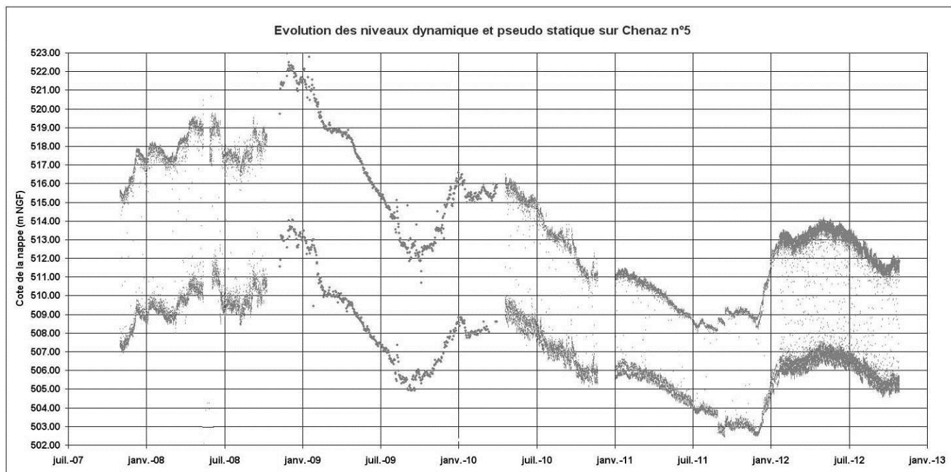
Graphique 38 : Evolution des niveaux dynamiques et pseudostatiques sur le forage de Chenaz n°5
