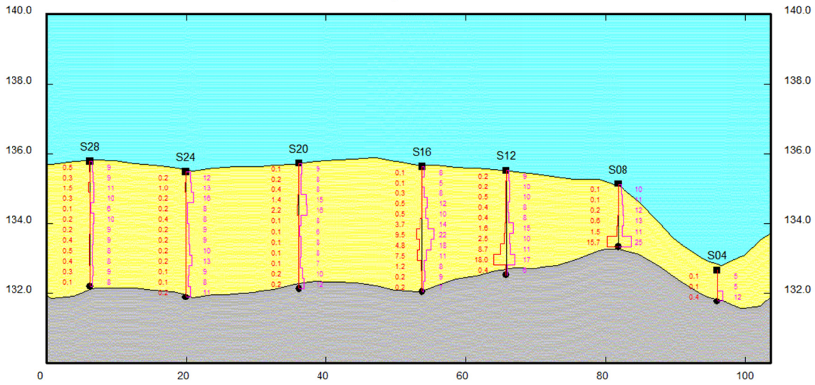
Coupe: 0004
