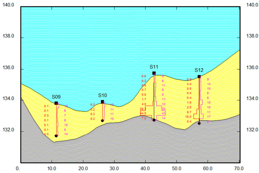
Coupe C
