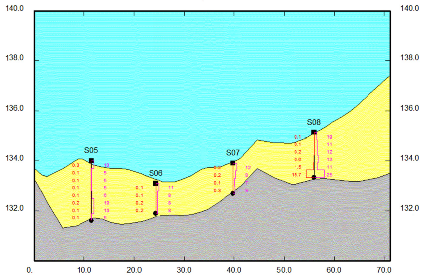
Coupe B
