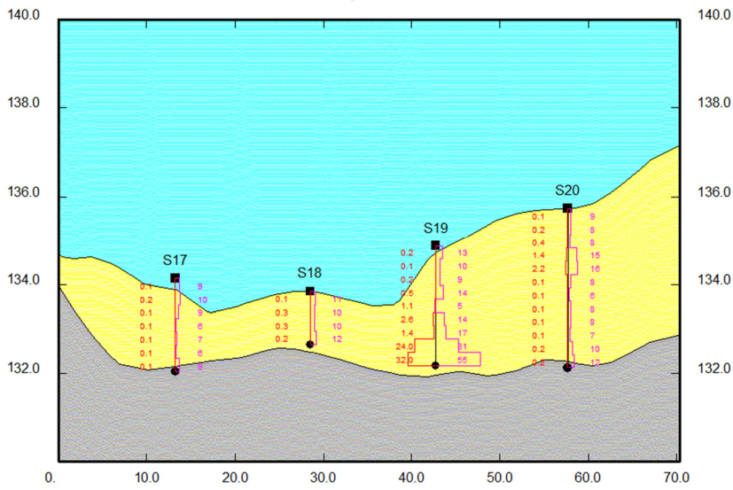
Coupe E
