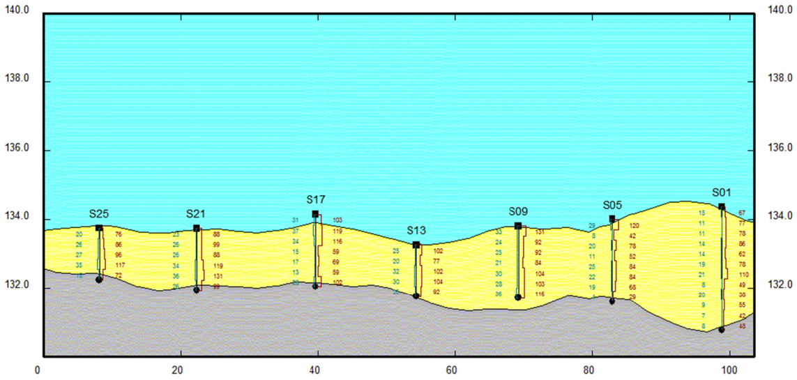
Coupe: 0001
