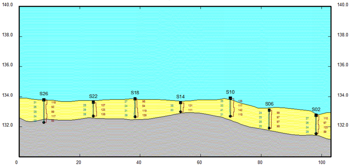
Coupe: 0002
