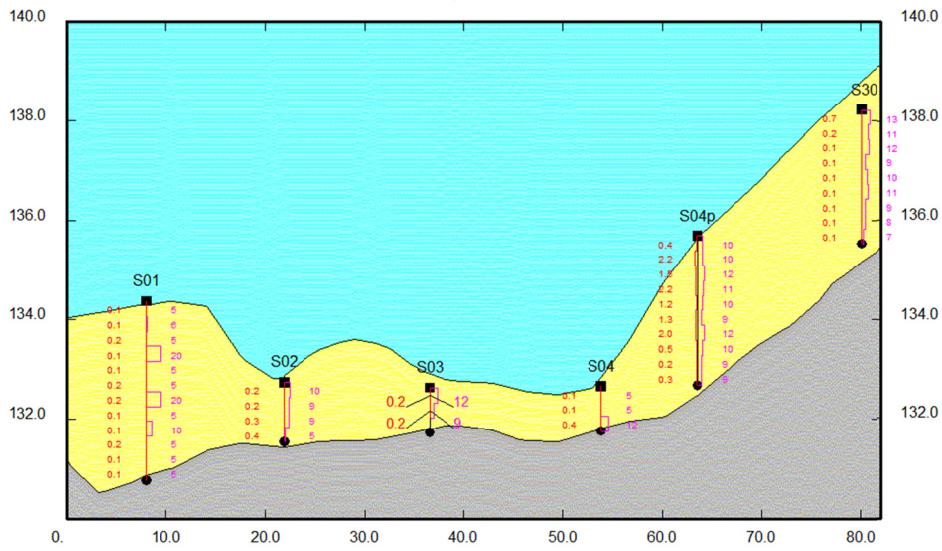
Coupe A
