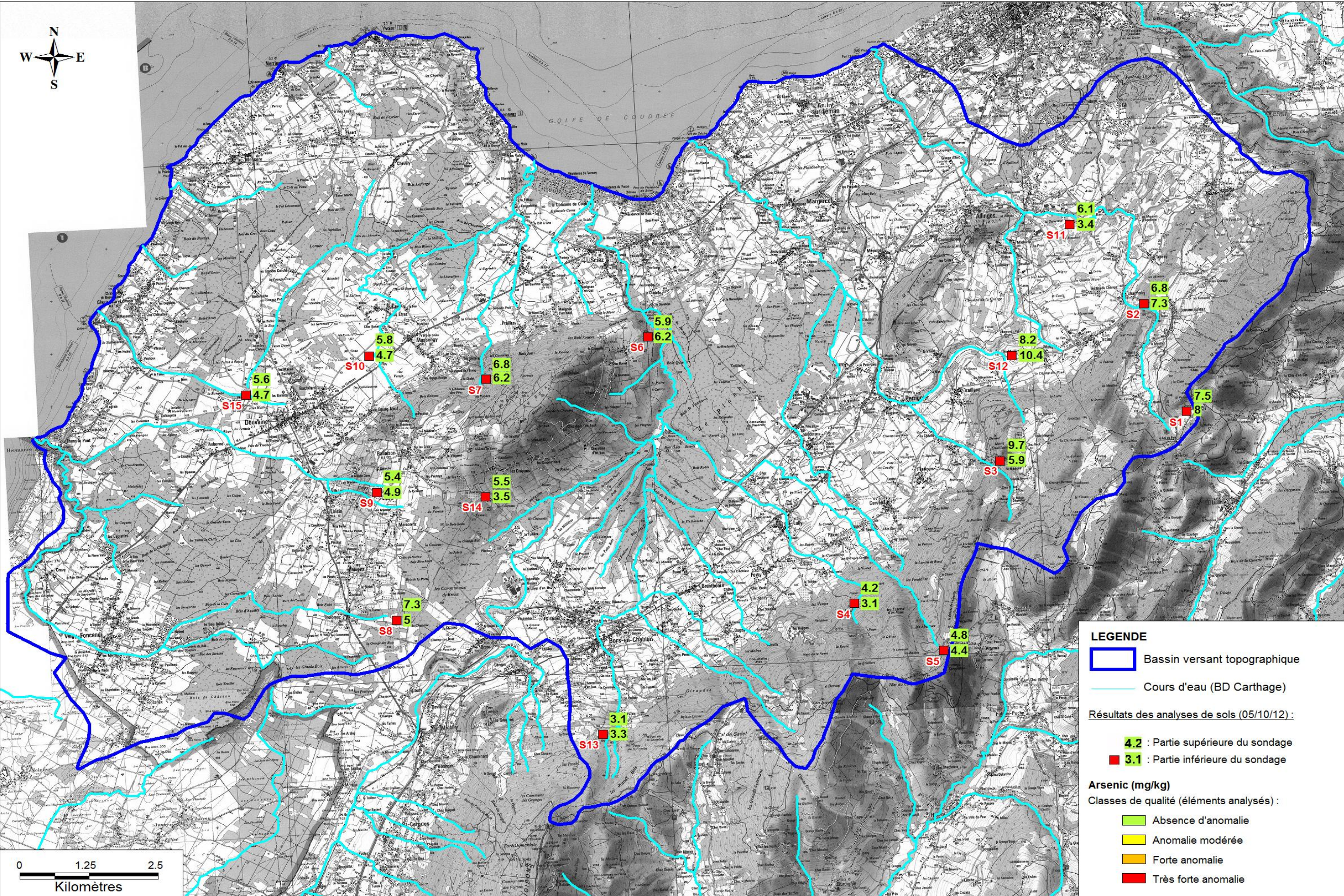
Figure 5 - a: Cartographie fond géochimique Arsenic
