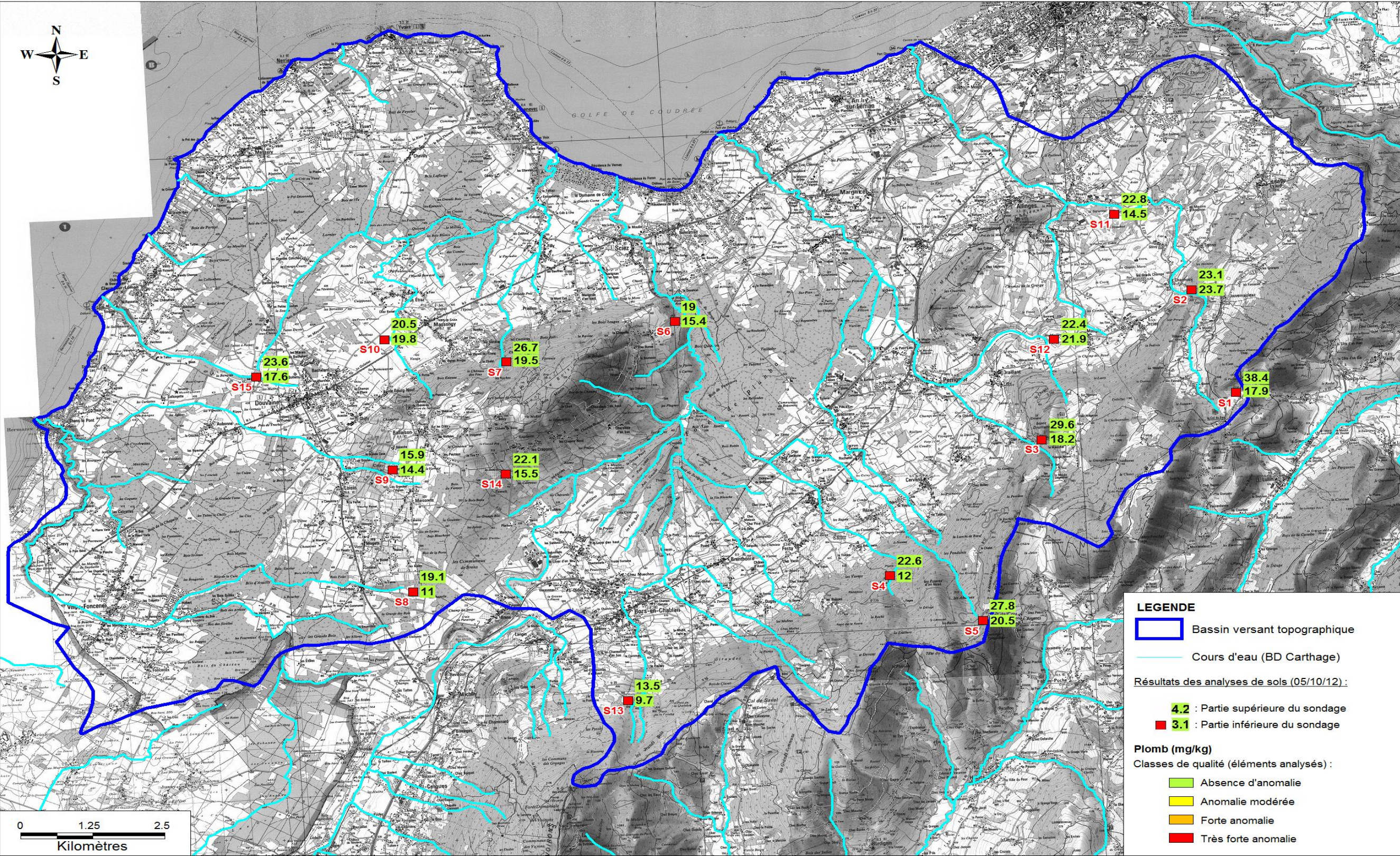
Figure 5 - c : Cartographie fond géochimique Plomb
