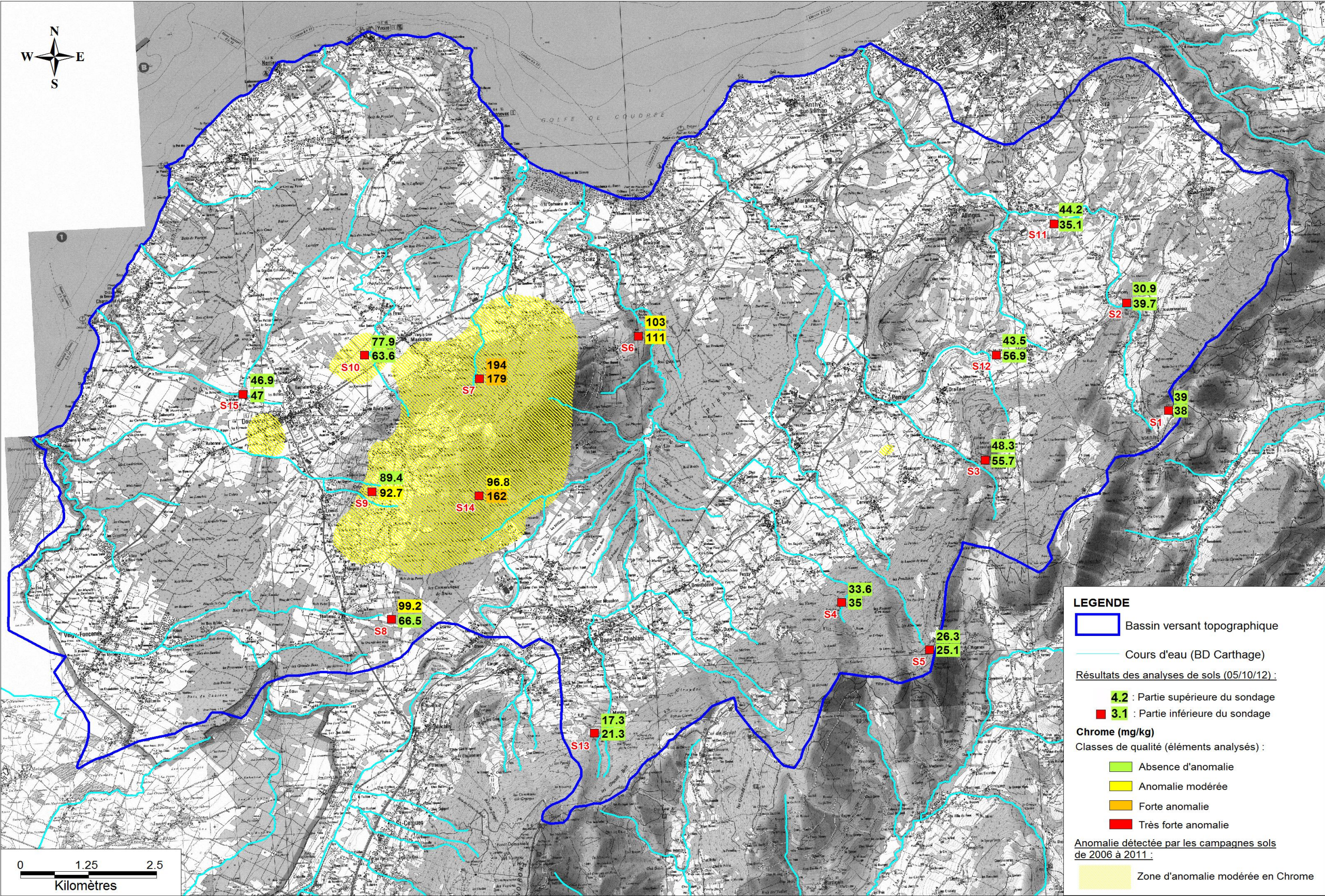
Figure 5 - d : Cartographie fond géochimique Chrome
