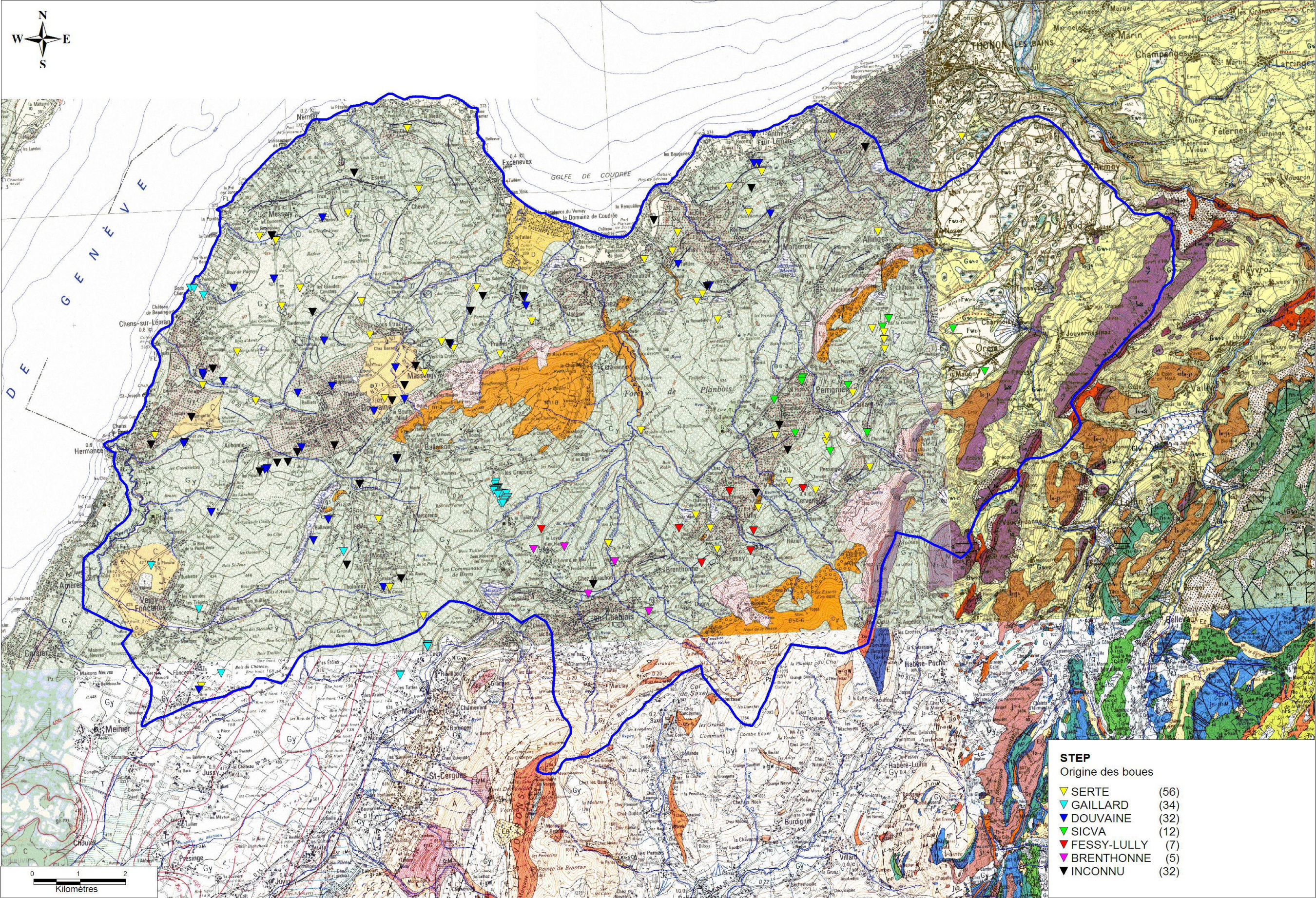
Figure 4 : carte de localisation des points de prélèvements sols « épandage » et origine des boues (BE BIRRAUX)
