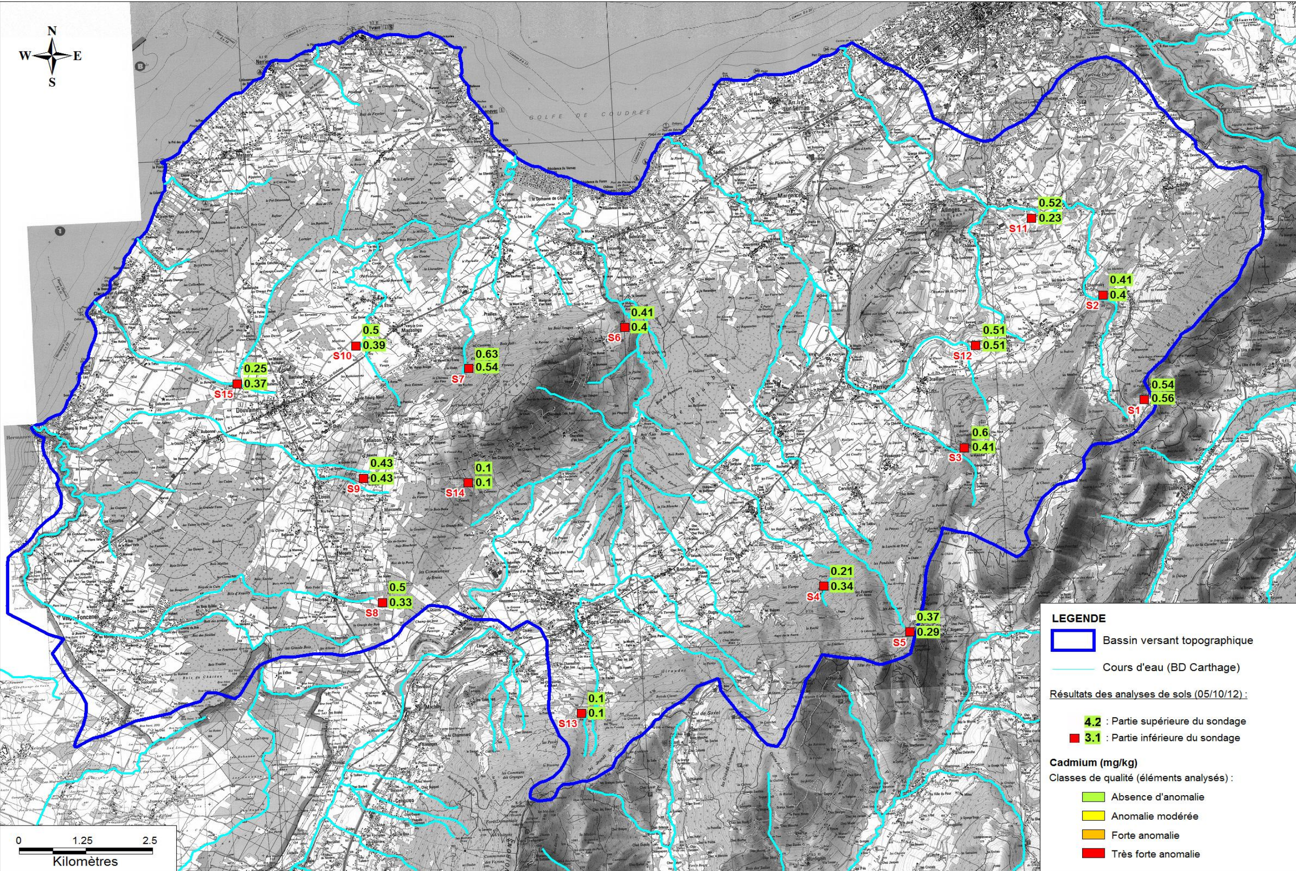
Figure 5 - b : cartographie fond géochimique Cadmium
