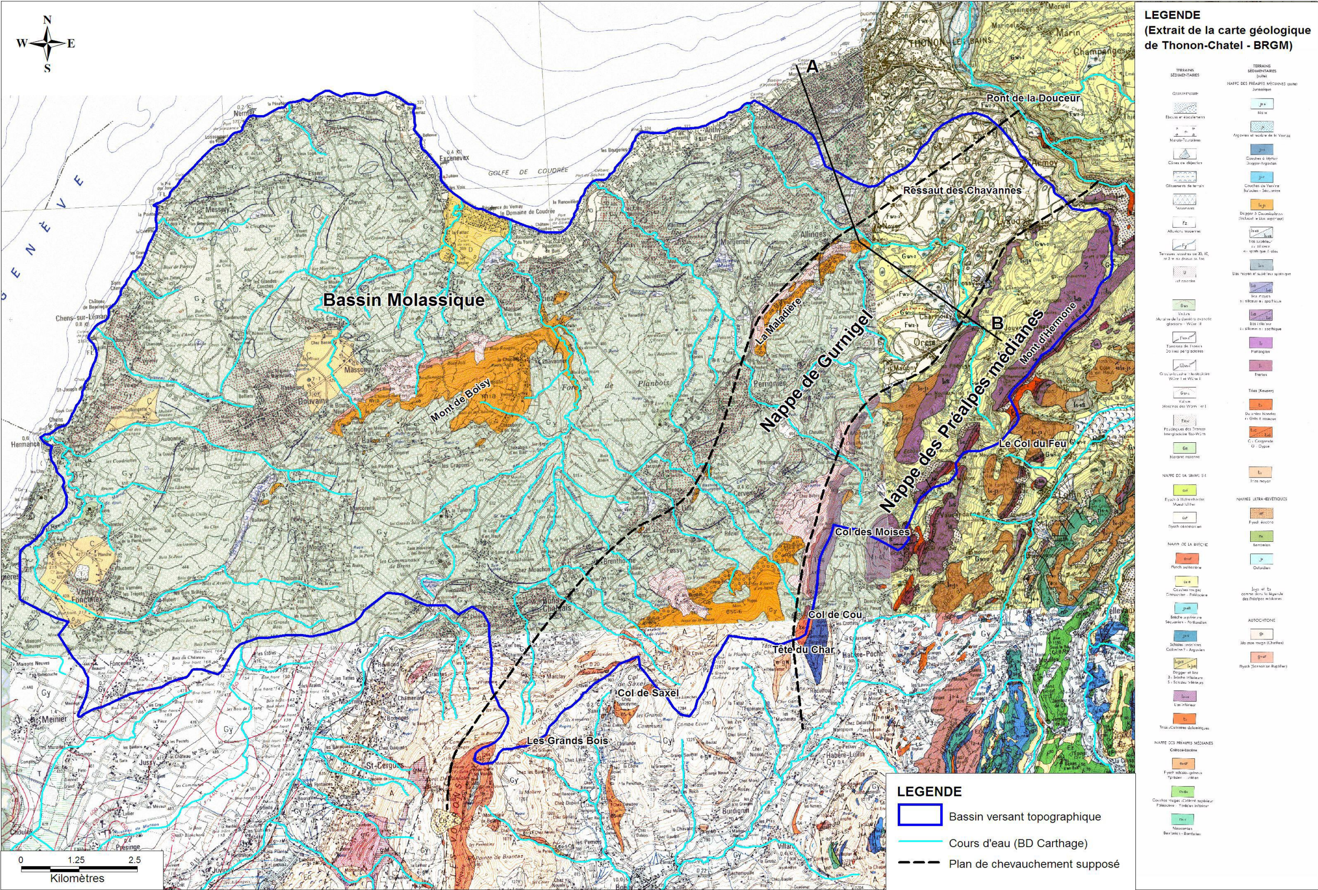
Figure 2 : Extrait des cartes géologiques de Thonon-Chatel et de Douvaine (Cartes BRGM au 1/50000)
