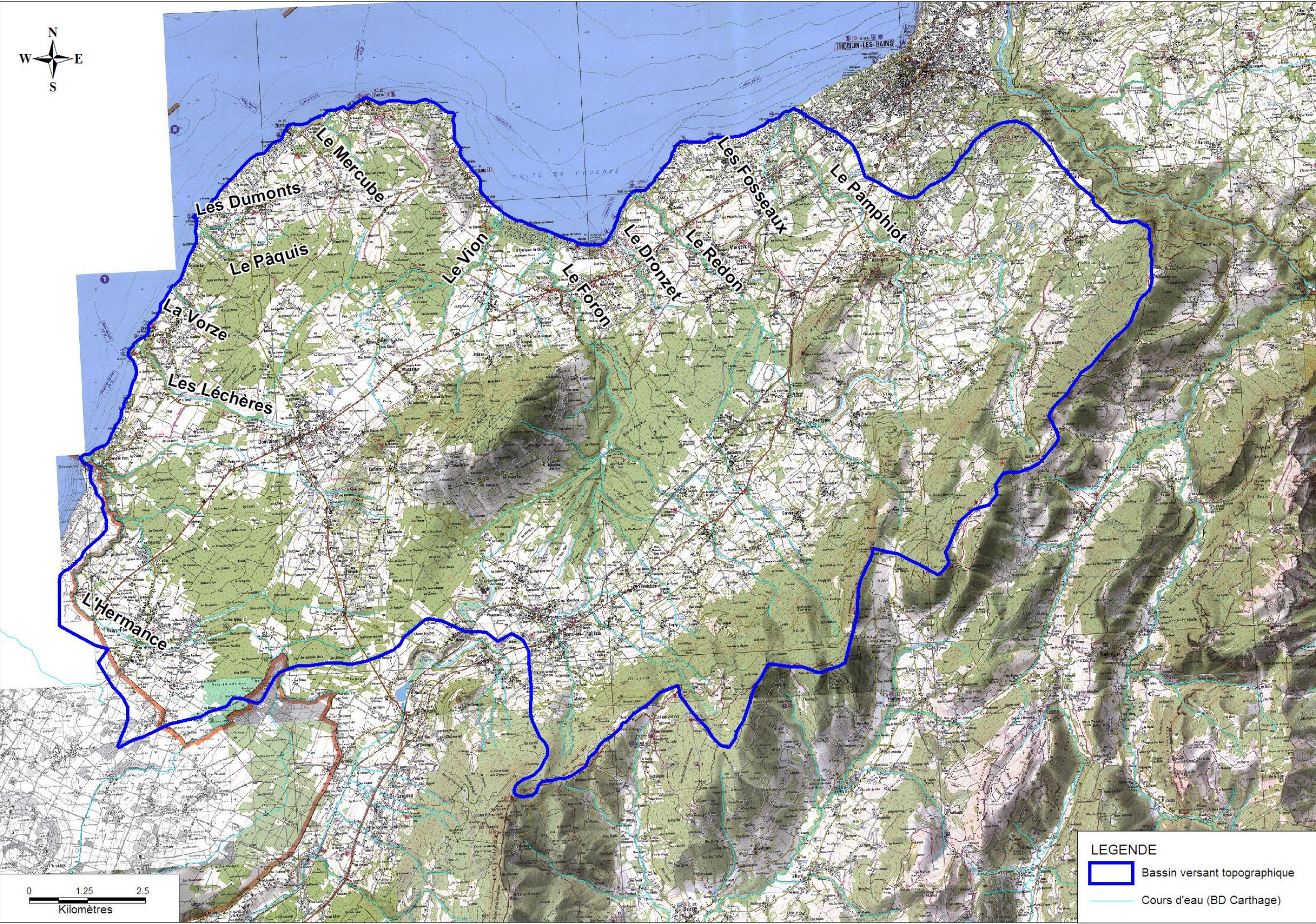
Figure 1 : Bassin versant topographique des affluents du sud-ouest lémanique
