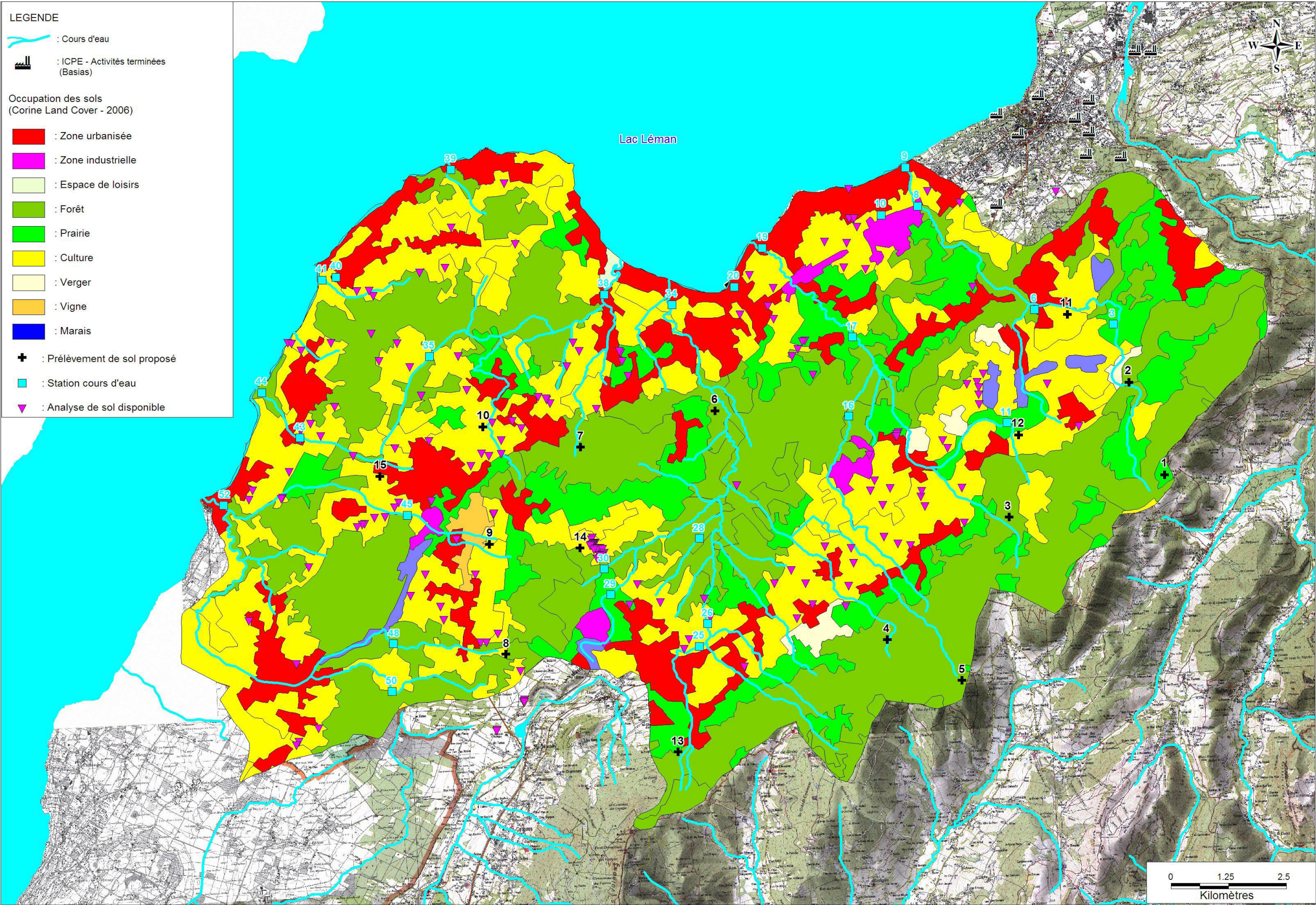
Figure 3 : carte de localisation des stations de mesures « sols »
