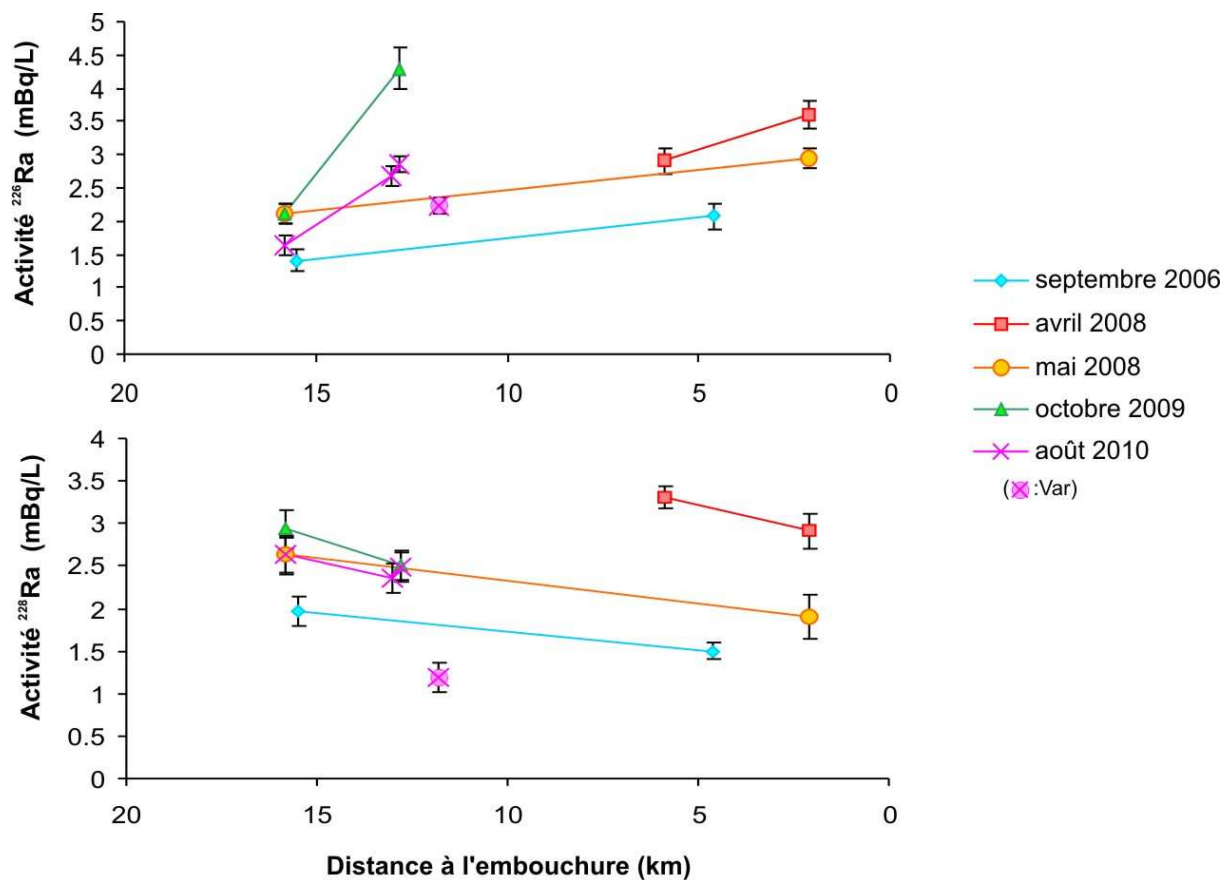
Figure 6. 4: Profils d'activité du ^{226}\text{Ra} et du ^{228}\text{Ra} (en \text{mBq.L}^{-1} )
