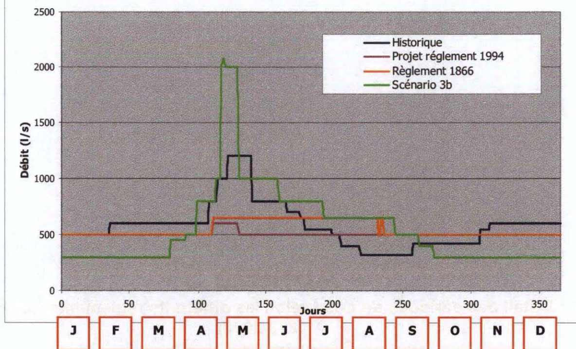
Débits d'alimentation de la Fure en 2005 historiques et recalculés
