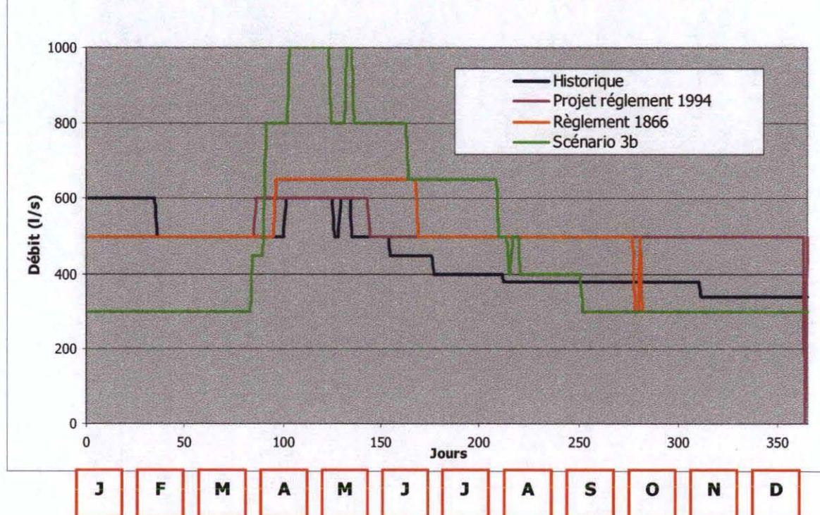
Débits d'alimentation de la Fure en 2006 historiques et recalculés
