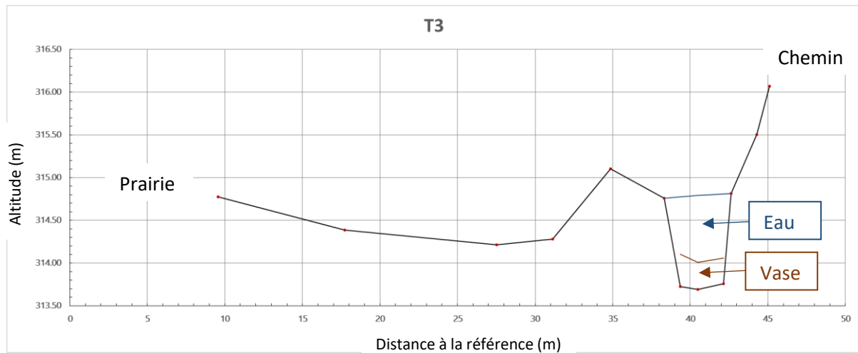
Figure 12. Profil en travers de la mare, transect n°3, cf. Figure 13
