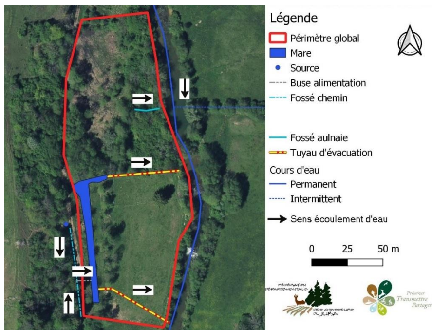
Figure 15. Schéma du fonctionnement hydrologique du site
