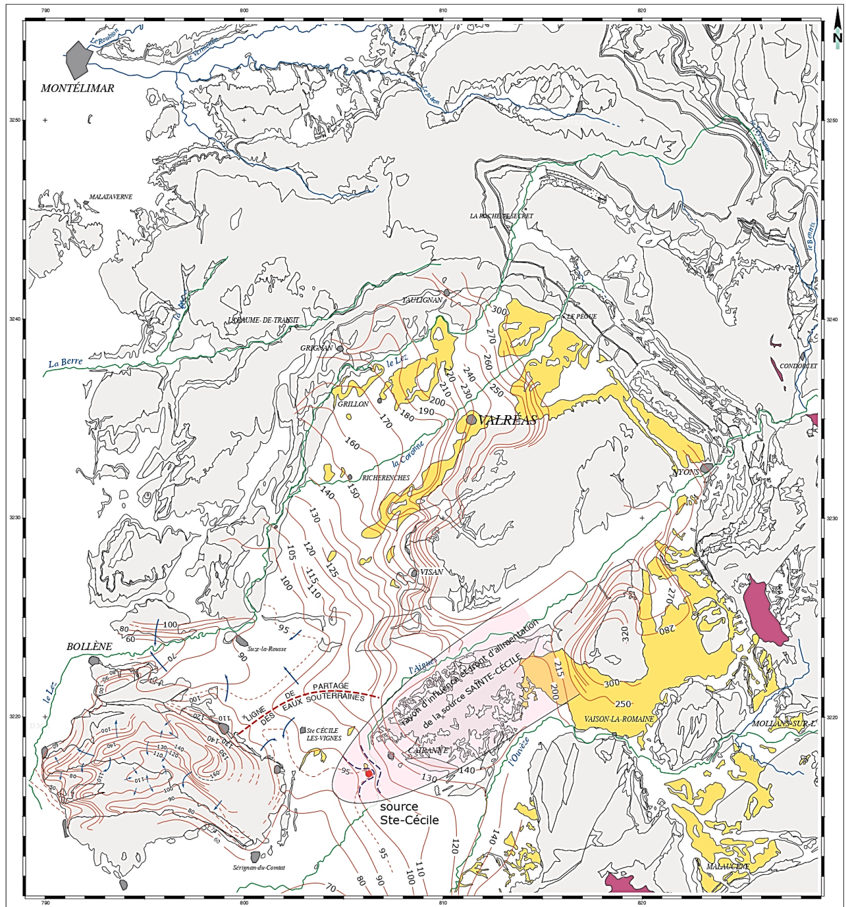
Fig. 12 Représentation piézométrique du toit de la nappe hébergée par le réservoir aquifère du Serravallo dans le bassin de Valréas.
