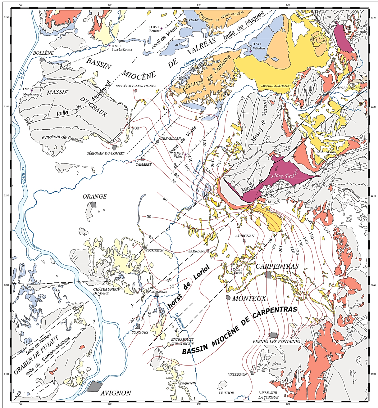
Fig. 13 Représentation piézométrique du toit de la nappe hébergée par le réservoir aquifère du Miocène (Burdigalien-Langhien-Serravallien) dans le bassin de Carpentras.
