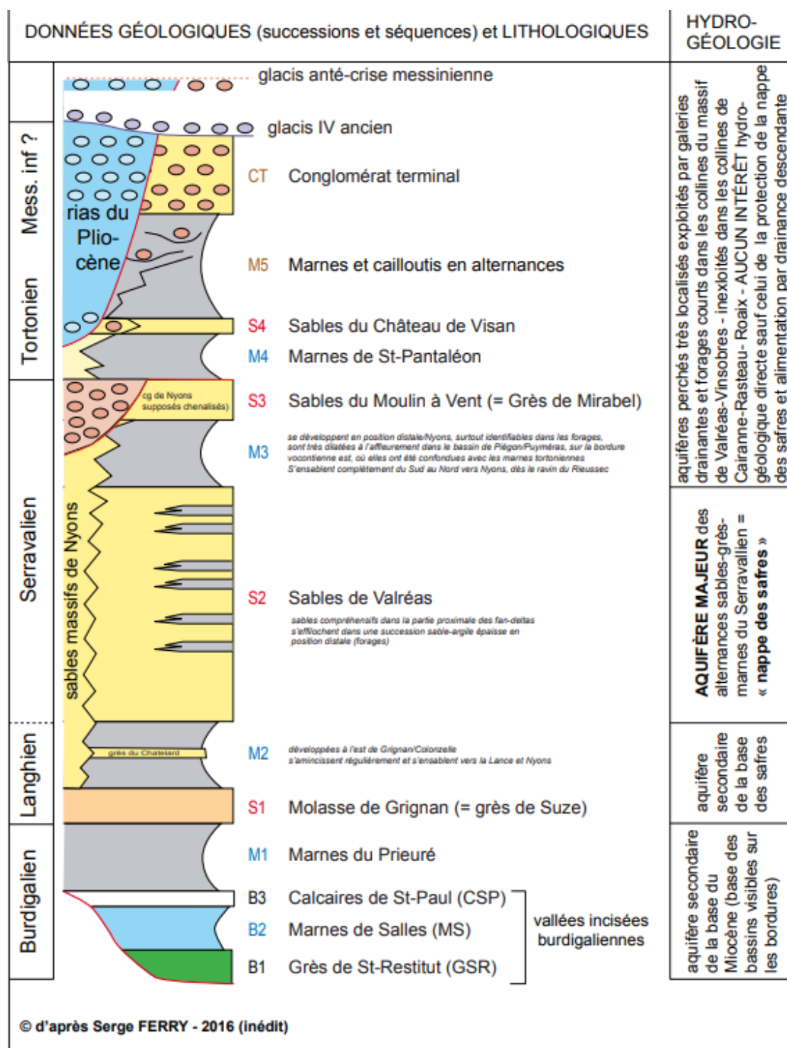
► Figure 6 : Représentation lithostratigraphique schématique des formations miocènes des bassins de Valréas et de Carpentras (GEOAPPLICATION, 2017)
