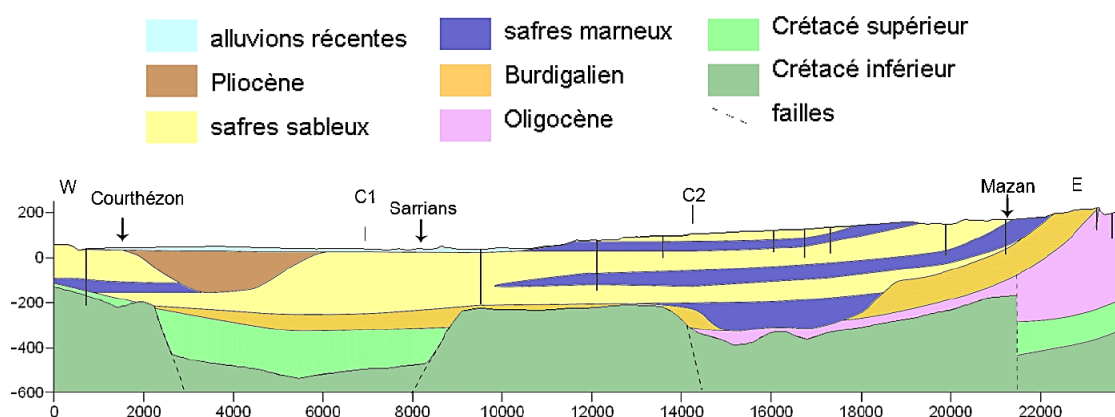
► Figure 14 : Structure schématisée de l'aquifère miocène du bassin de Carpentras (LALBAT, 2006) (les niveaux représentés en bleu constituent des épaves pour ou moins continues et imperméables pouvant stratifier les écoulements au sein de la molasse)
