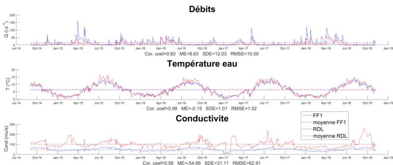
Figure 70. Comparaison entre la sonde FF1 et la sonde RDL a) débits, b) température, c) conductivité
