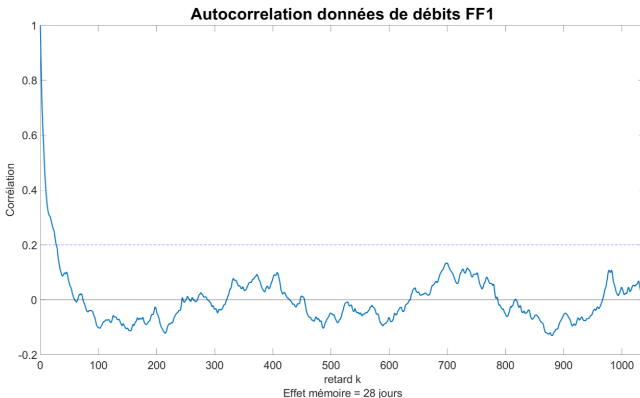
Figure 55. Autocorrélogramme du signal de débits issus de la sonde FF1
