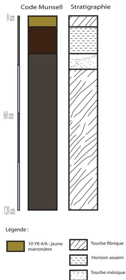
Profil P1-S7
