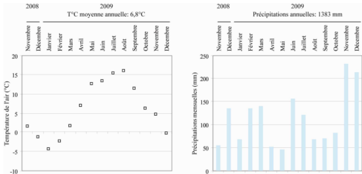
Figure 22. Diagramme ombrothermique, mesures des températures et des précipitations (hors neige) pour la période novembre 2008 – décembre 2009 (Delarue, 2010)
