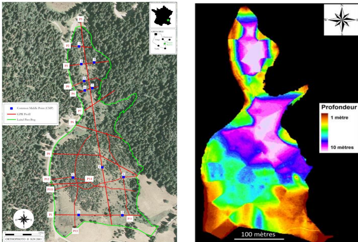
Figure 7. a) Carte des profils d'acquisitions géophysiques (Garambois, 2008) b) Cartographie du socle minéral de la tourbière du Col du Luitel par interpolation des profils géophysiques (Ravatin, 2017)
